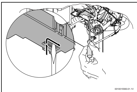
Rys. 26 Resetowanie mikroprzełącznika
