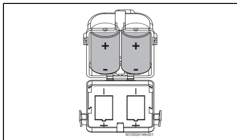
Rys. 3 Montaż baterii
