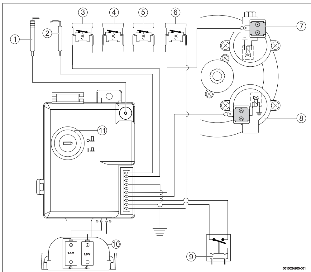
Rys. 28 Schemat elektryczny
