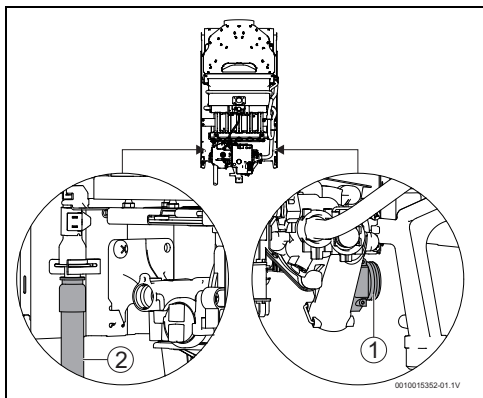
Rys. 11 Przyłącze wody
