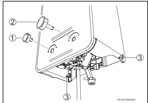
Rys. 14 Zdjąć obudowę
