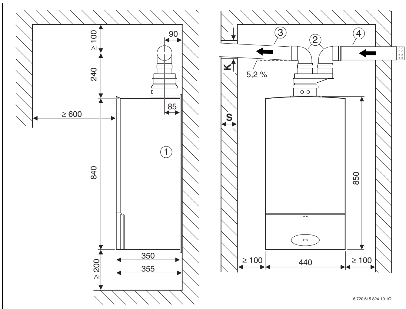
Rys. 14 \varnothing 80/80 mm
