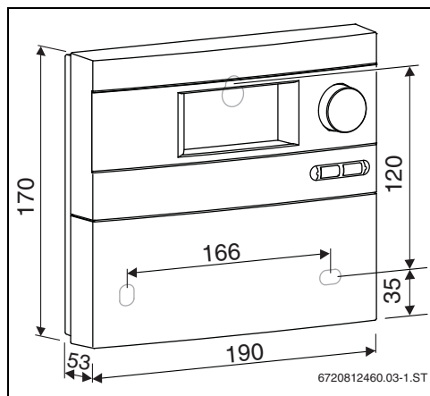
Rys. 4 Wymiary obudowy
