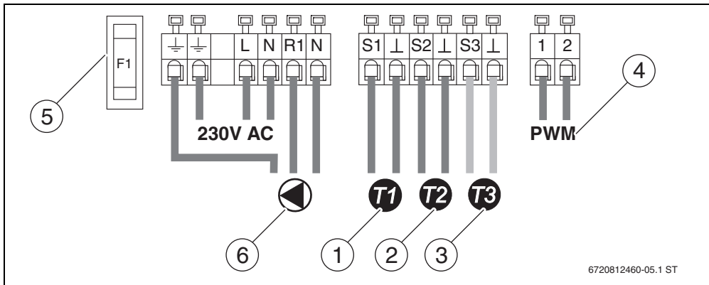
Rys. 8 Schemat połączeń
