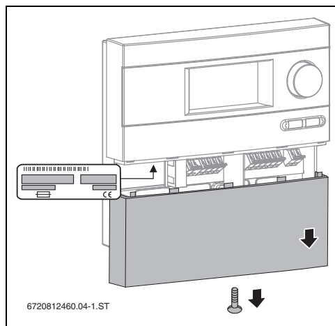
Rys. 5 Tabliczka znamionowa
