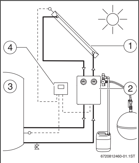
Rys. 3 Schemat instalacji
