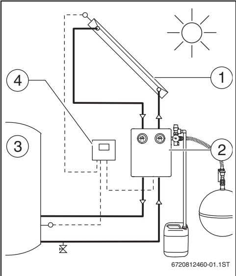
Obr. 3 Schéma systému
