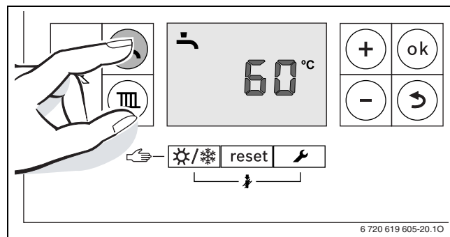
Rys. 43 Wskazanie temperatury c.w.u.
