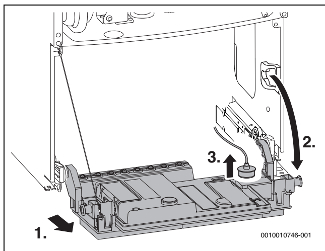
Rys. 78 Odchylenie sterownika ku dołowi
