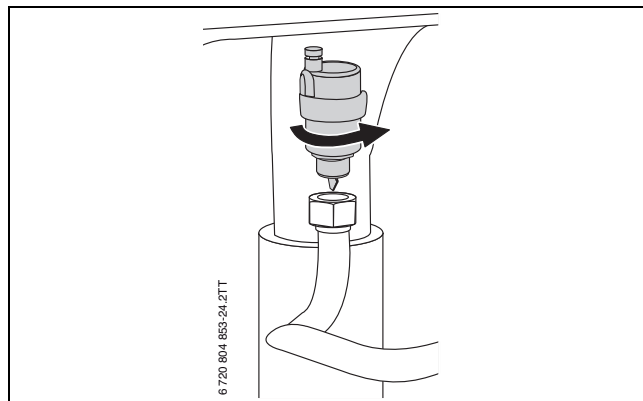
Rys. 71 Demontaż automatycznego odpowietrznika
