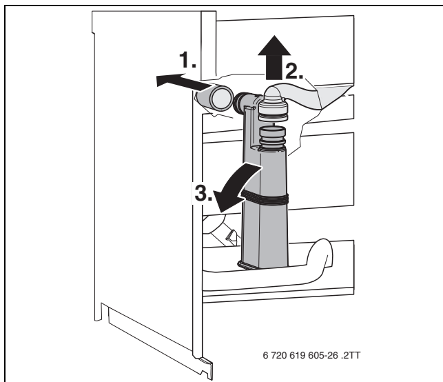
Rys. 66 Demontaż syfonu kondensatu
