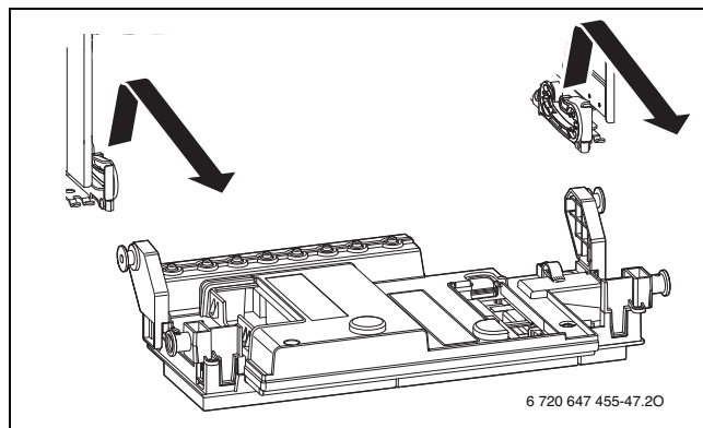
Rys. 80 Wyczepienie sterownika
