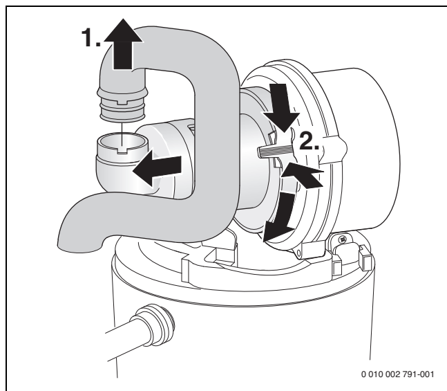
Rys. 58 Demontaż rury ssącej i zespołu mieszającego
