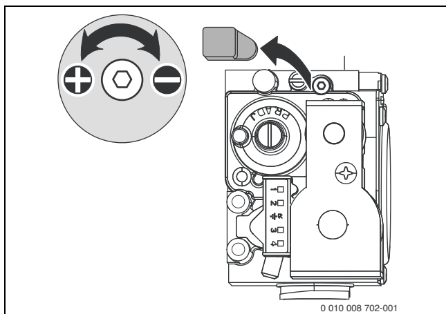
Rys. 52 Zdjęcie plomby
