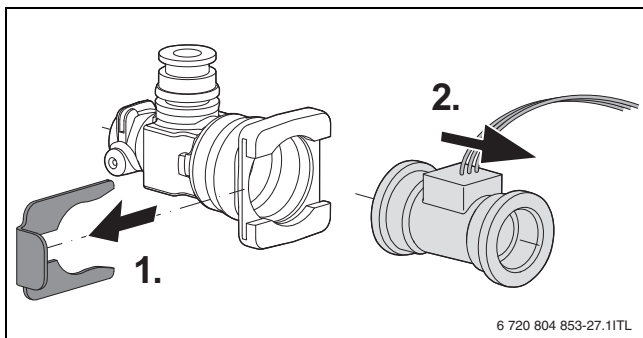
Rys. 70 Demontaż turbiny z rury wody zimnej
