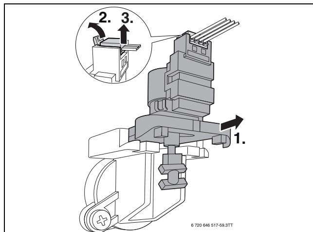
Rys. 72 Zdemontować napęd zaworu 3-drogowego
