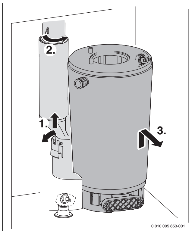
Rys. 83 Demontaż wymiennika ciepła
