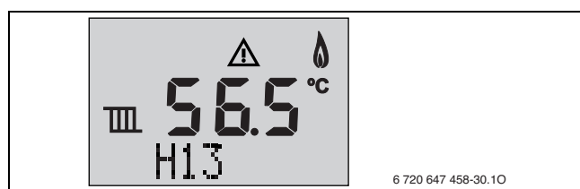
Rys. 84 Przykład: usterka niepowodująca zablokowania
