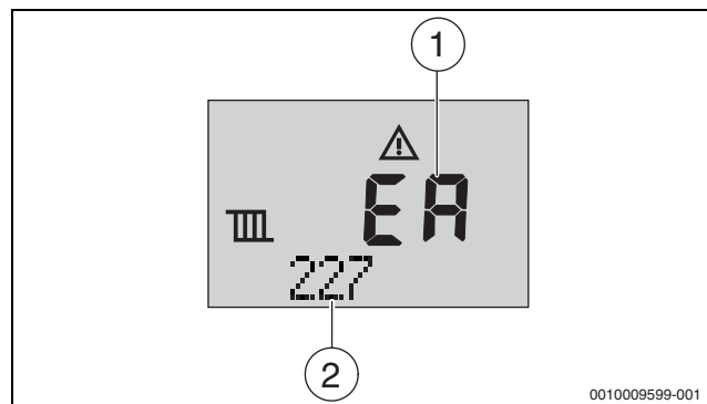
Rys. 85 Przykład: wskazanie usterki nieprzemijającej
