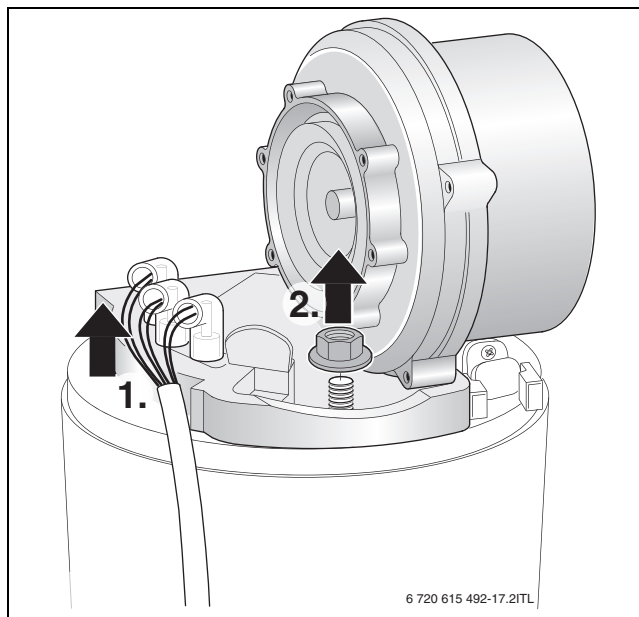
Rys. 59 Wyjmowanie wentylatora
