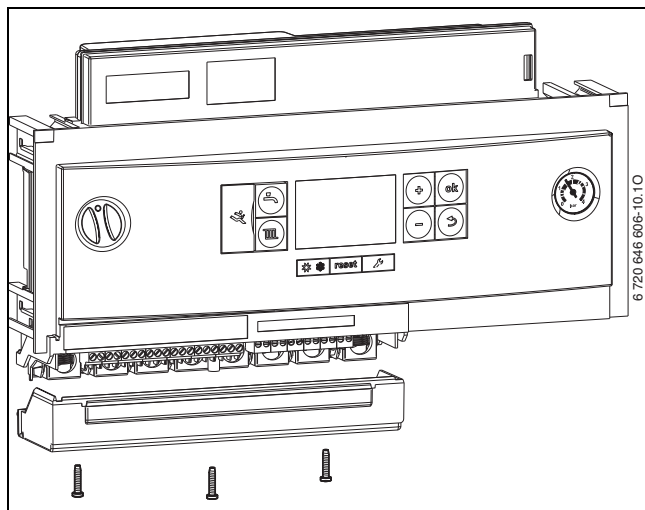
Rys. 77 Zdjęcie pokrywy
