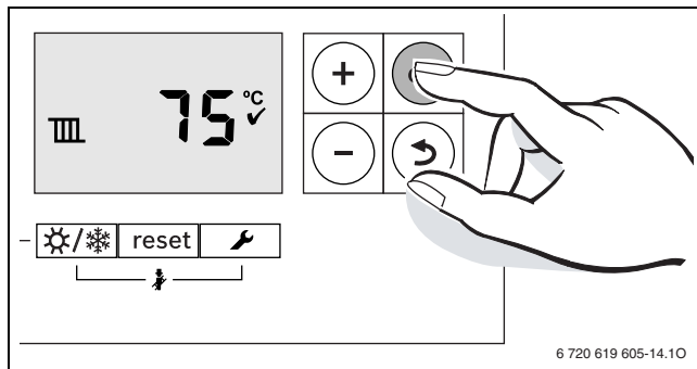
Rys. 40 Potwierdzenie wskazania temperatury zasilania
