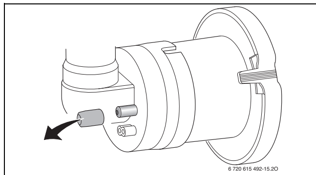
Rys. 57 Króciec pomiarowy na zespole mieszającym
