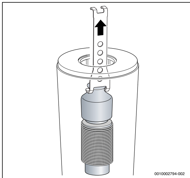
Rys. 61 Wyjmowanie górnego elementu wyporowego
