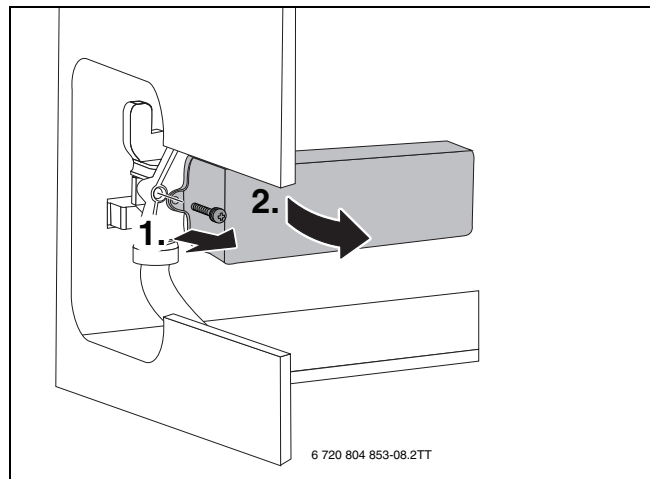
Rys. 68 Demontaż płytowego wymiennika ciepła
