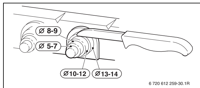
Rys. 35 Dopasować uchwyt odciążający do średnicy kabla
