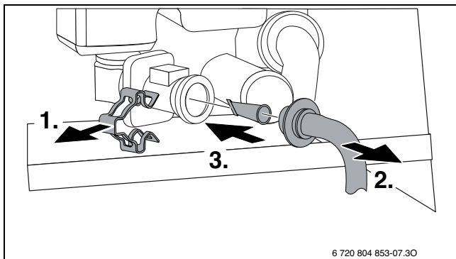
Rys. 69 Demontaż sitka z rury wody zimnej
