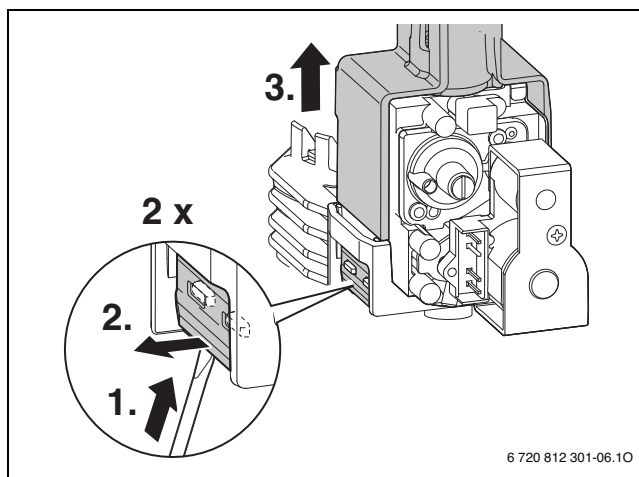
Rys. 76 Demontaż armatury gazowej
