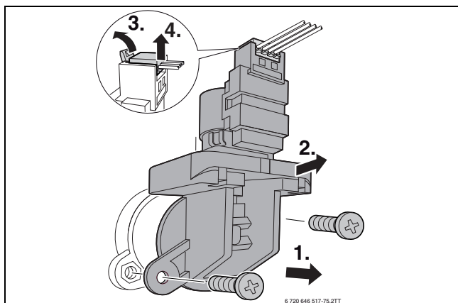
Rys. 73 Demontaż zaworu 3-drogowego
