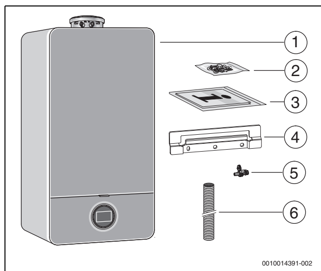
Rys. 1 Zakres dostawy
