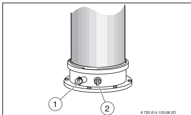
Rys. 56 Króćce pomiarowe spalin oraz powietrza do spalania
