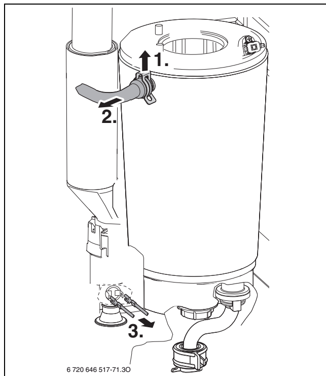
Rys. 81 Uwalnianie rury zasilającej i odłączanie kabla
