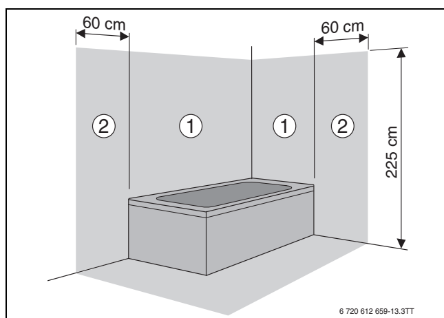
Rys. 33 Strefy ochronne
