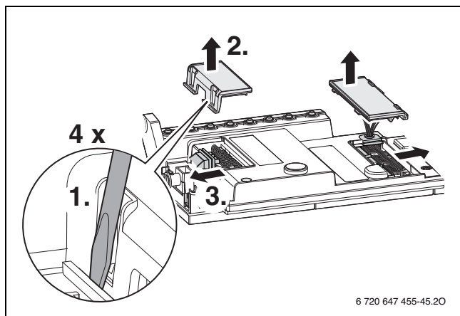
Rys. 79 Zdjęcie pokrywy
