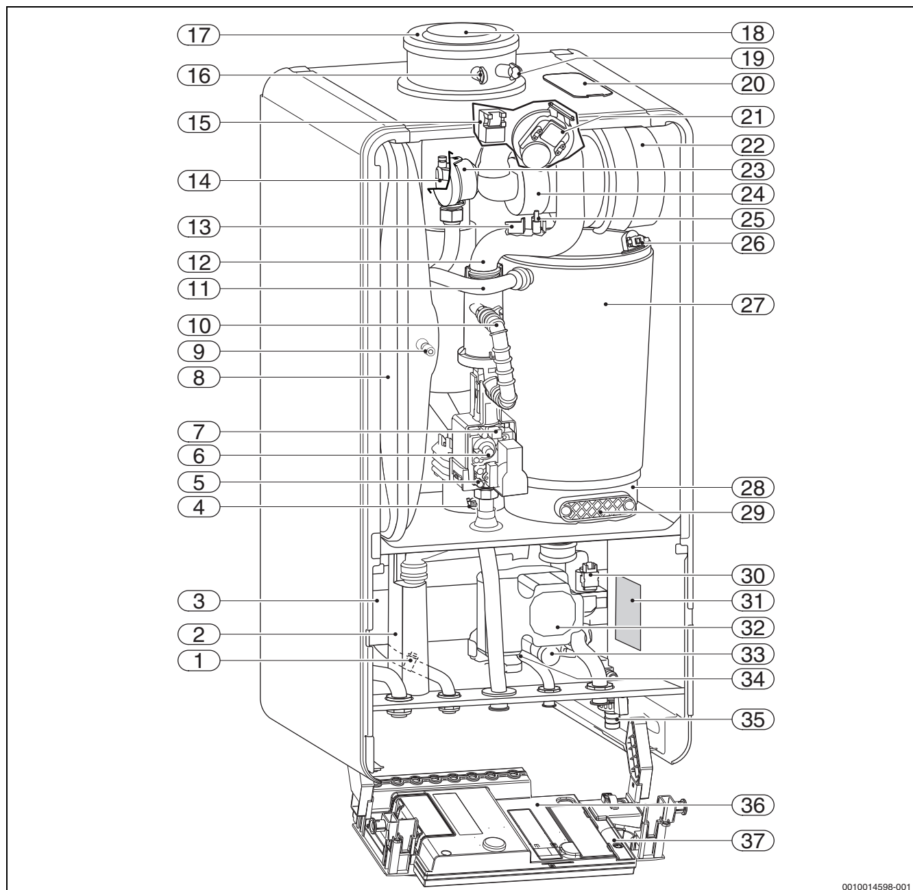
Rys. 3 Przegląd produktu
