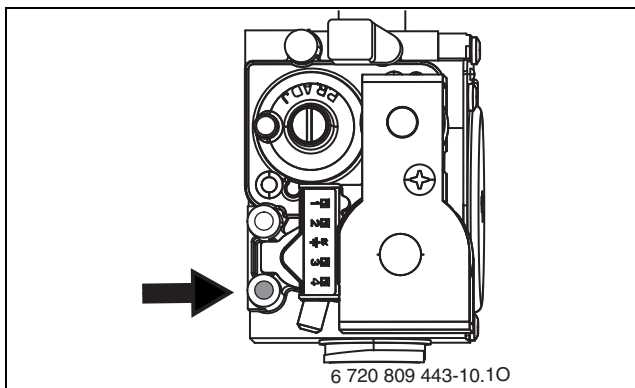
Rys. 54 Króciec pomiarowy ciśnienia gazu na przyłączy
