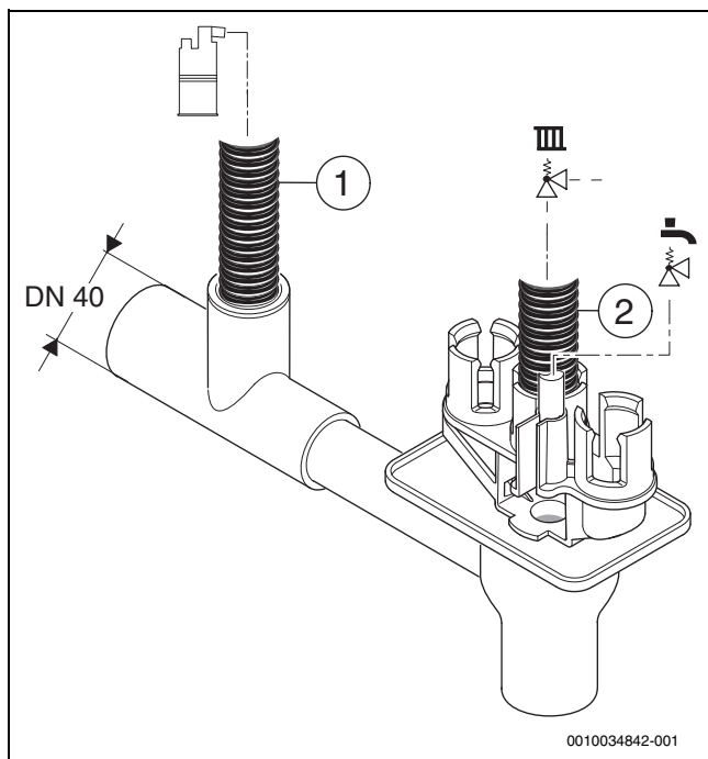
Rys. 31 Montaż węży kondensatu i węży zaworu bezpieczeństwa na syfonie
