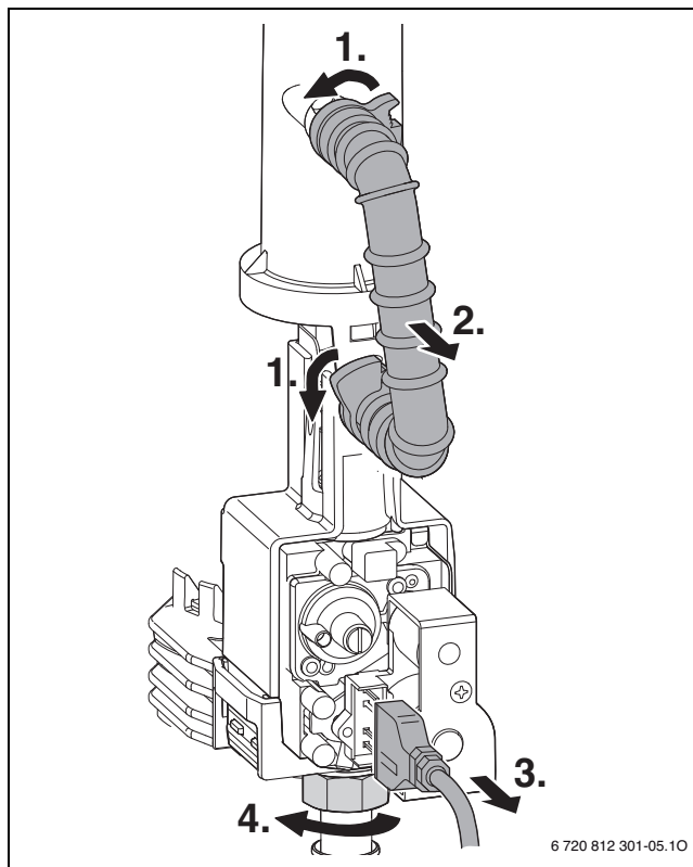
Rys. 75 Demontaż armatury gazowej
