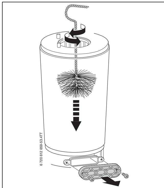
Rys. 63 Czyszczenie wymiennika ciepła
