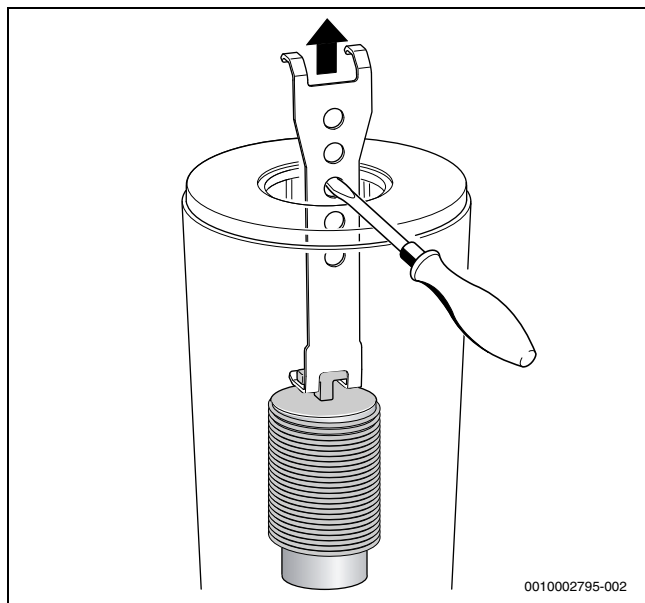
Rys. 62 Wyjmowanie dolnego elementu wyporowego
