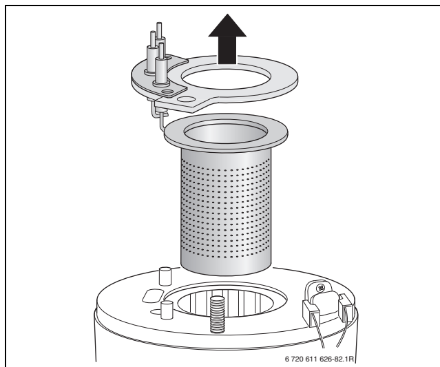
Rys. 60 Wyjmowanie palnika
