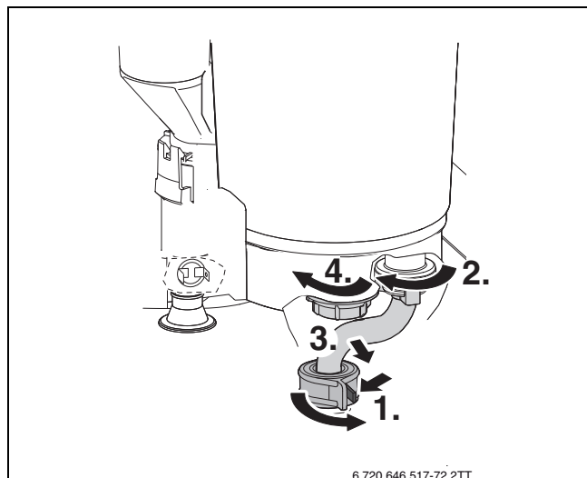
Rys. 82 Wykręcanie nakrętki i uwolnienie rury powrotu
