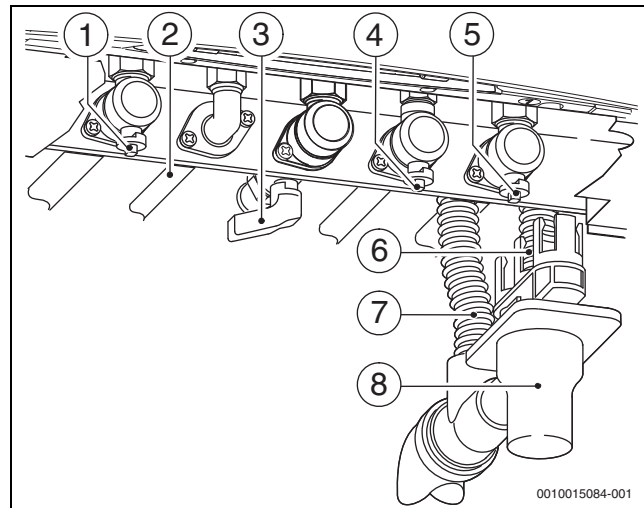
Rys. 32 Przyłącza po stronie gazowej oraz wodnej (osprzęt dodatkowy)
