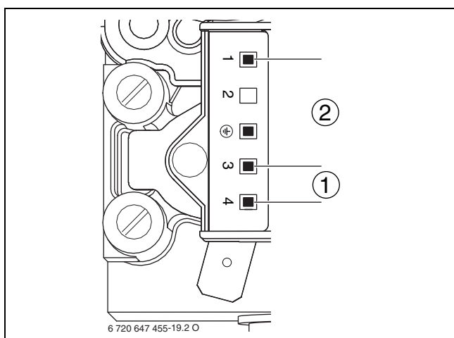
Rys. 74 Punkty pomiarowe na armaturze gazowej
