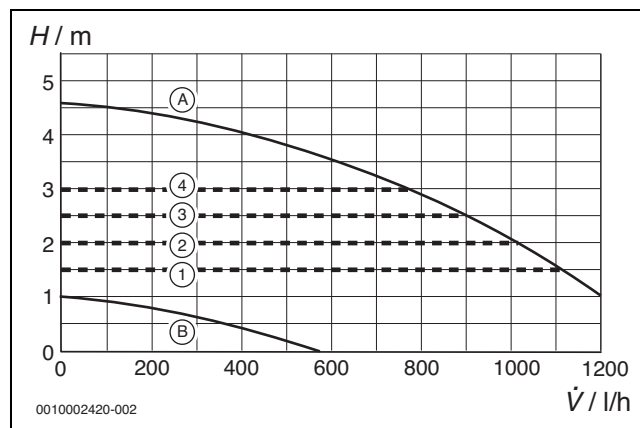
Rys. 88 Charakterystyki wykreślnie pompy i charakterystyki pompy
