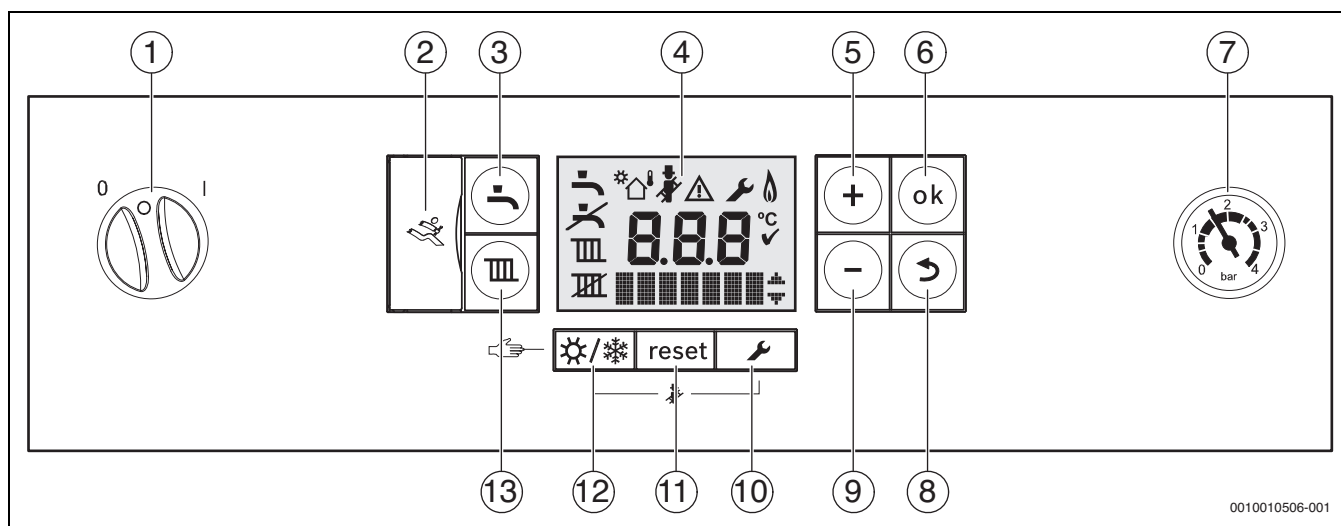
Rys. 36 Panel obsługi ze zdjętą osłoną
