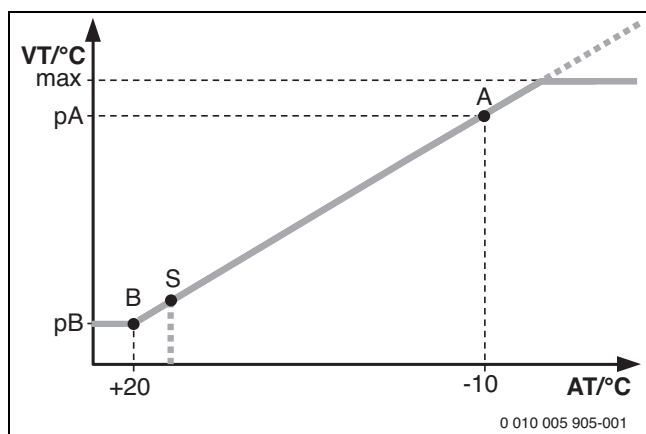
Rys. 87 Krzywa grzewcza
