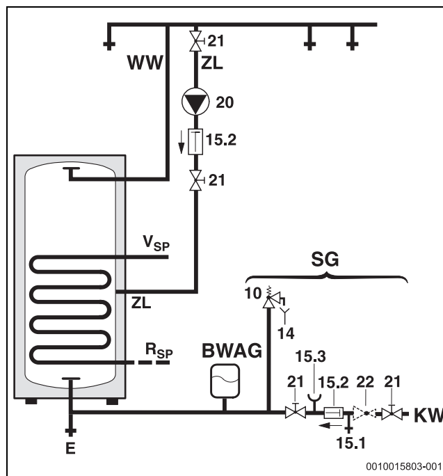
Fig. 2 Schema di collegamento dell'acqua potabile
