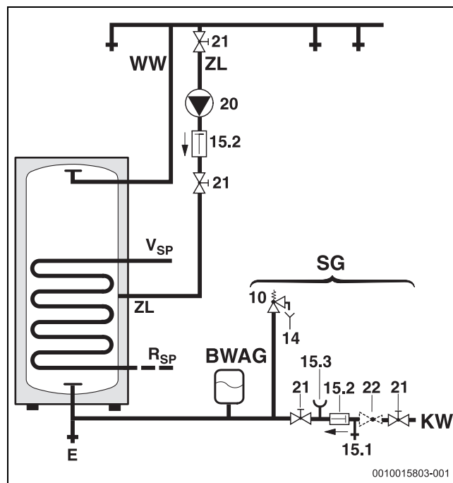
Afb. 5 Aansluitschema drinkwaterzijde
