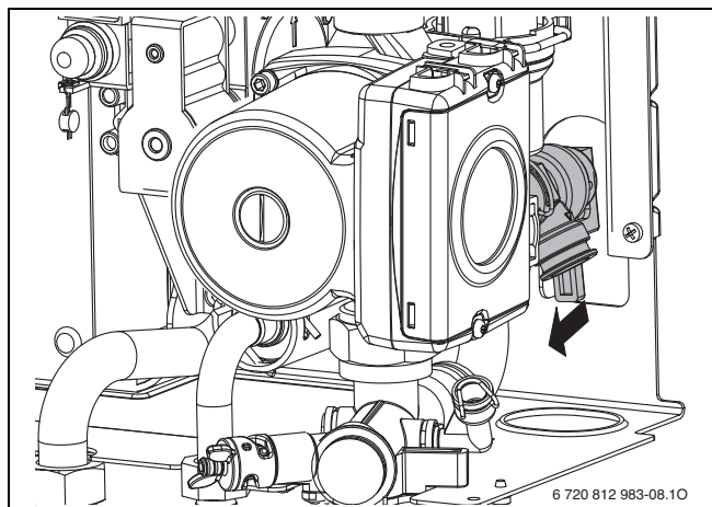
Rys. 53 Zawór bezpieczeństwa (instalacja grzewcza)
