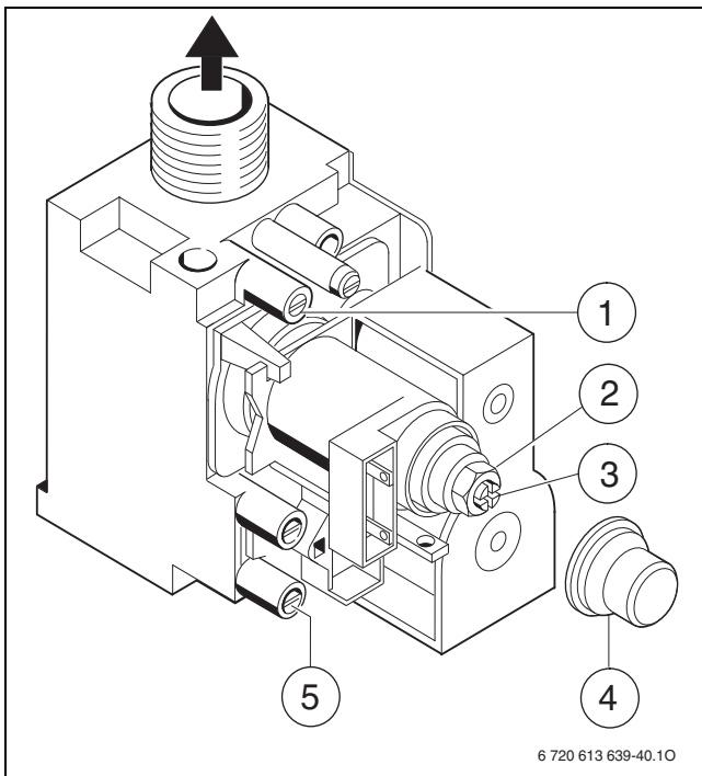
Rys. 35 Armatura gazowa
