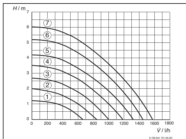
Rys. 29 Charakterystyki pomp
