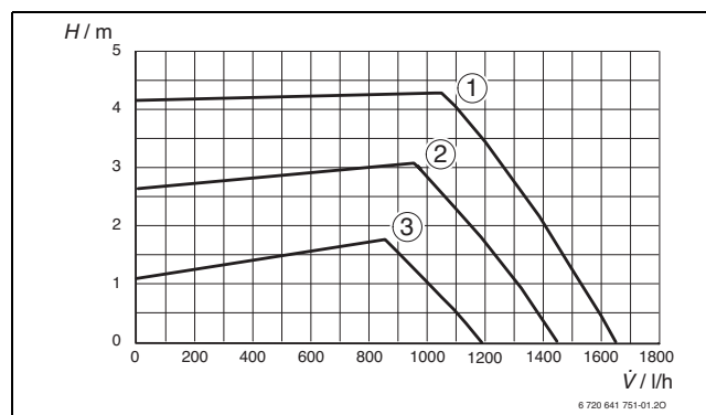
Rys. 27 Ciśnienie stałe
