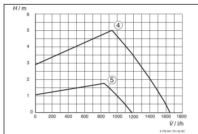
Rys. 28 Ciśnienie proporcjonalne
