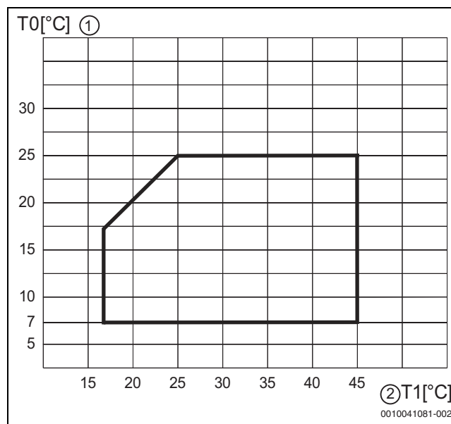
Rys. 5 Pompa ciepła w trybie chłodzenia
