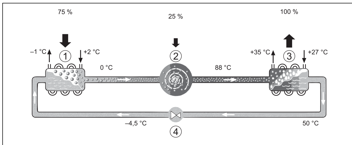
Rys. 6 Zasada działania obiegu czynnika chłodniczego w pompie ciepła
