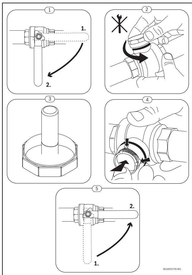
Rys. 14 Czyszczenie filtra magnetycznego
