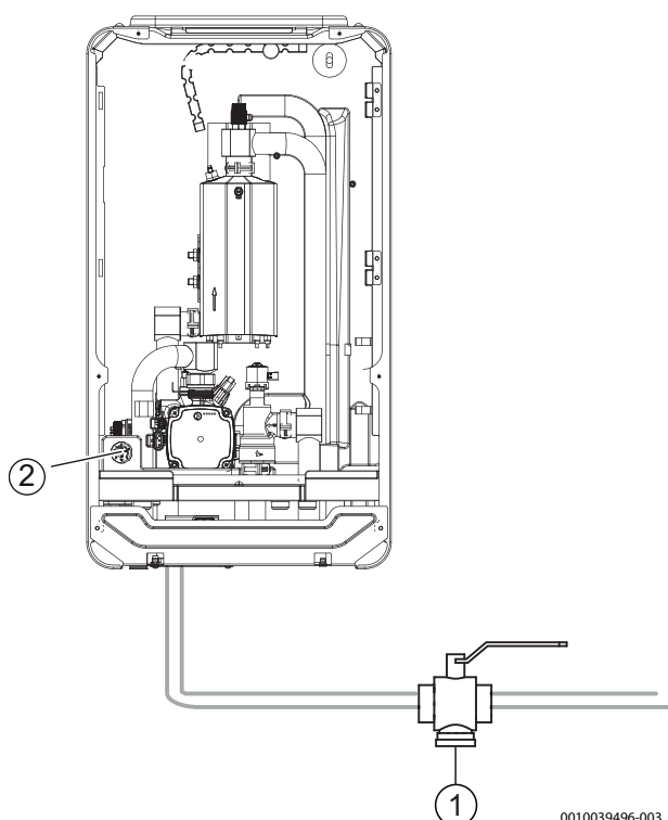
Rys. 11 Jednostka wewnętrzna Compress 5800/6800i 12 E
