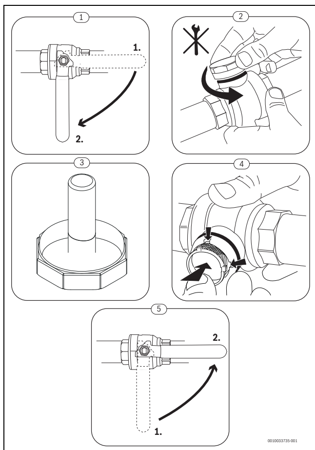
Rys. 12 Czyszczenie filtra magnetycznego
