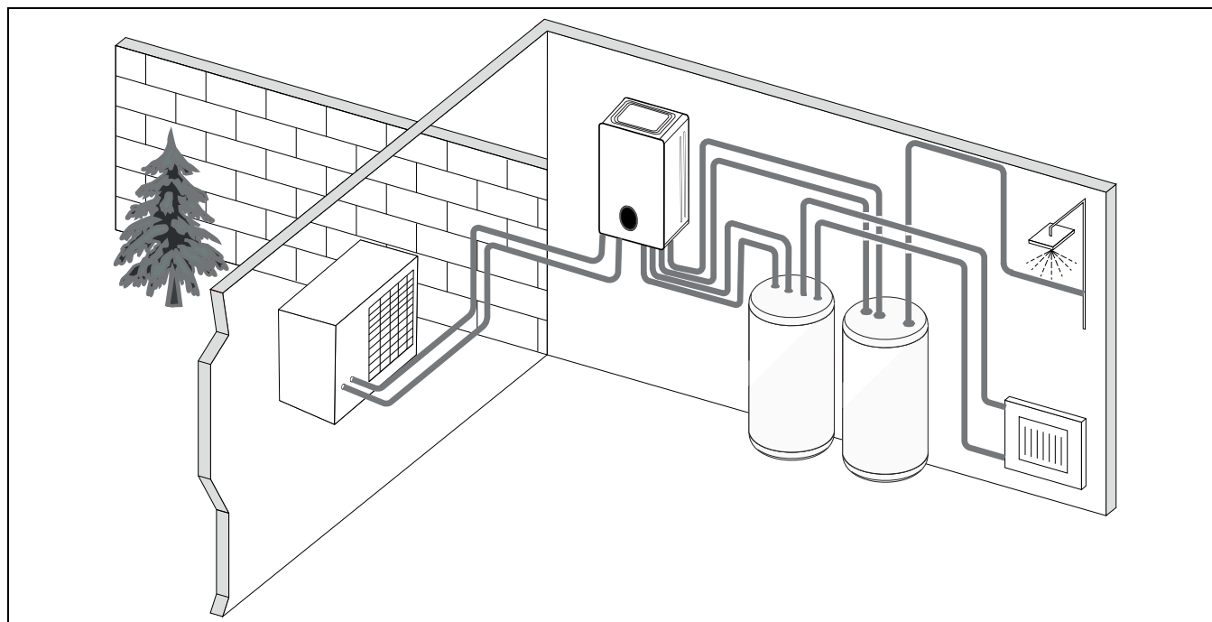
Rys. 5 Pompa ciepła AW OR, jednostka wewnętrzna Compress 5800/6800i 12 E z grzałką zanurzeniową i zewnętrznym podgrzewaczem pojemnościowym c.w.u.
