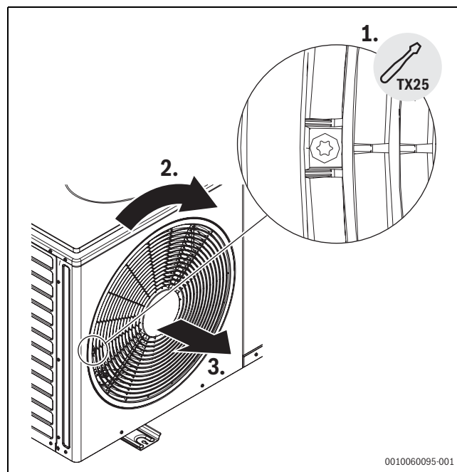
Rys. 37 Instrukcje demontażu ramki wentylatora
