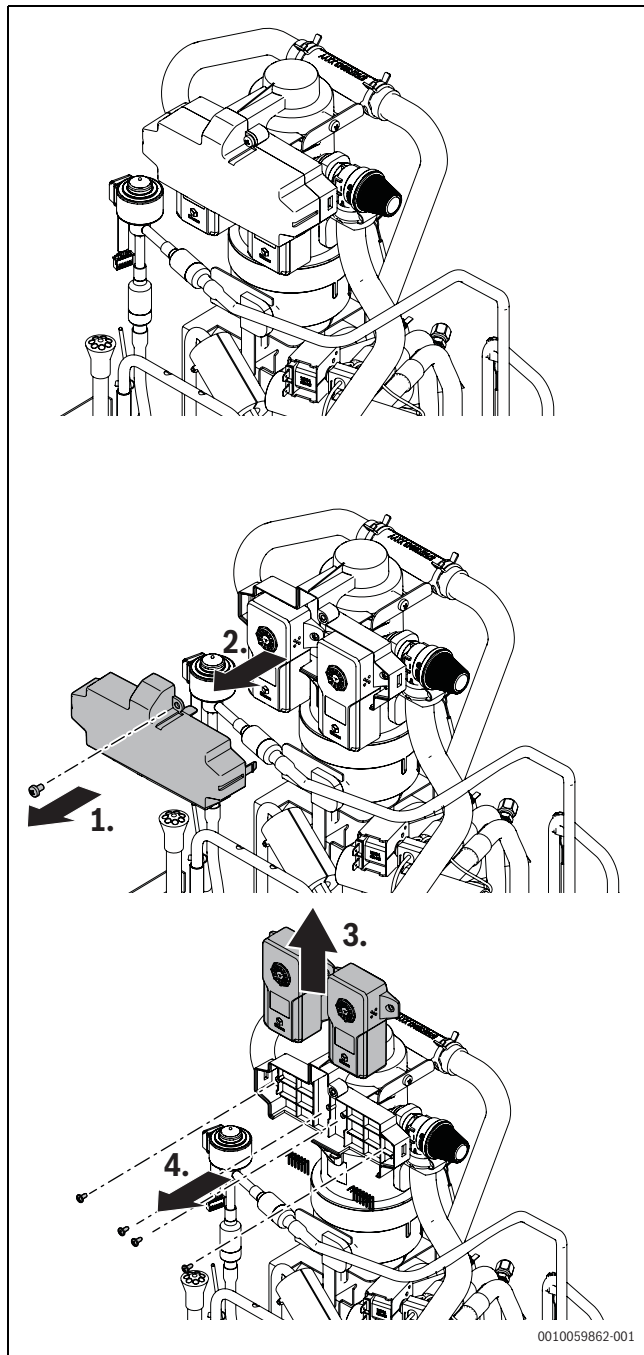
Rys. 42 Wymiana czujników R290
