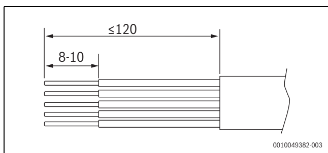
Rys. 34 Usuwanie izolacji z żył do przyłącza prądu (mm)
