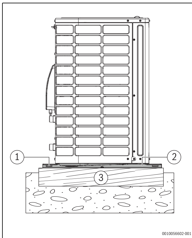
Rys. 24 Przymocowanie pompy ciepła
