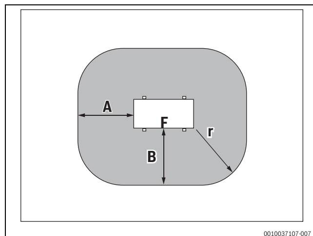
Rys. 9 Obszar bezpieczeństwa, ustawienie na ziemi na wydzielonym terenie lub na dachu, widok z góry
