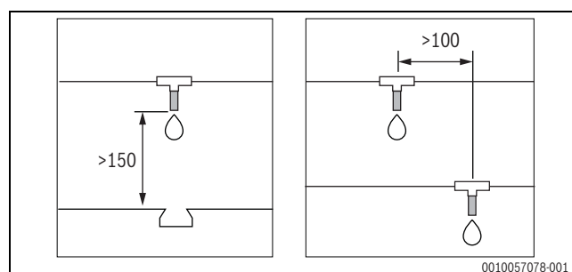
Rys. 23 Odległości instalacji zaworu środka przeciw zamarzaniu w milimetrach (mm)
