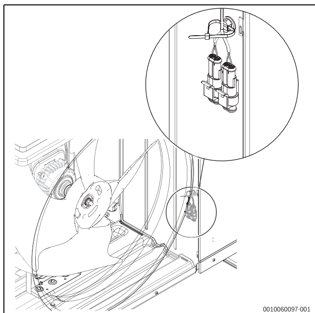
Rys. 39 Połączenie podgrzewacza tacy ociekowej i przewodu grzewczego
