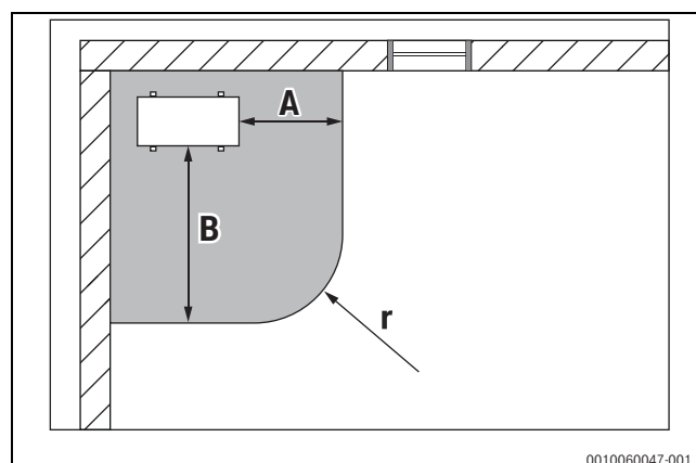
Rys. 11 Obszar bezpieczeństwa, ustawienie na ziemi w narożniku, widok z góry
