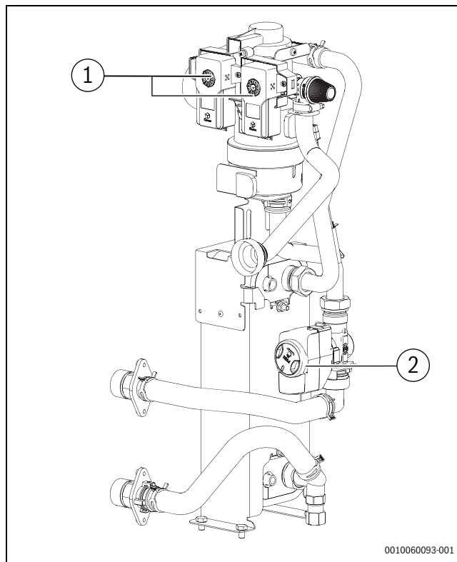
Rys. 41 Zestaw bezpieczeństwa propanu
