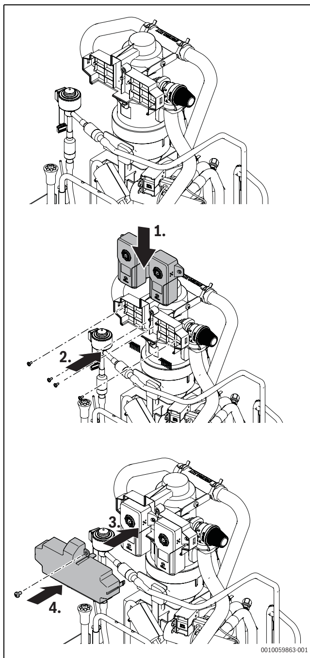
Rys. 43 Wymiana czujników R290
