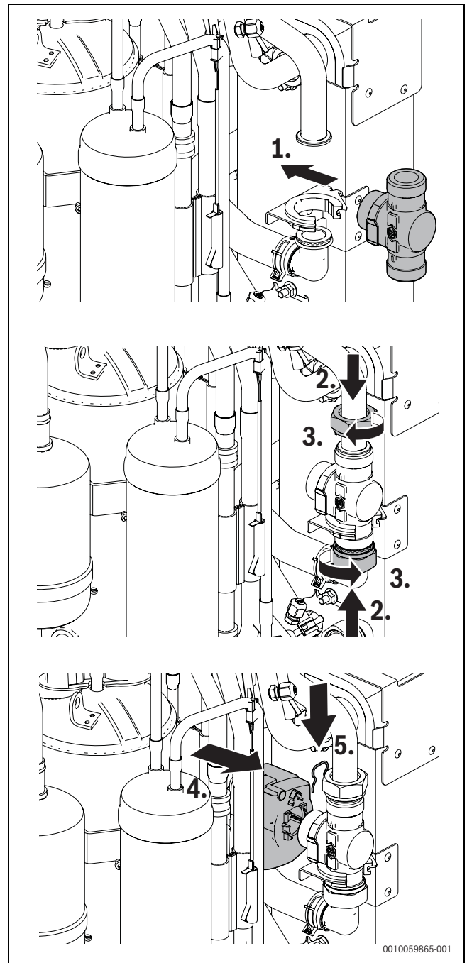
Rys. 45 Wymiana NCV
