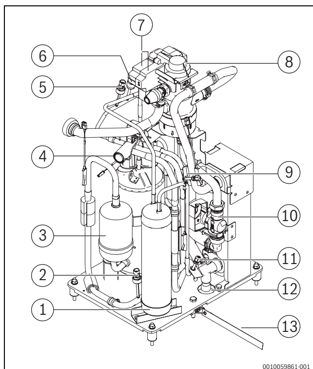
Rys. 2 Przegląd obiegu czynnika chłodniczego
