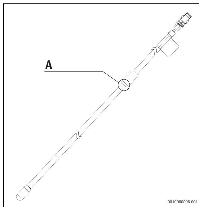
Rys. 38 Przewód grzewczy do rury odpływowej
