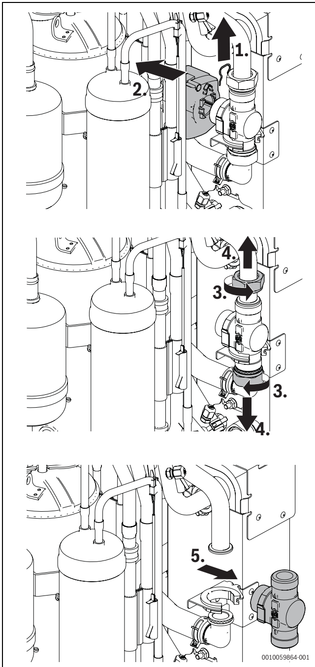
Rys. 44 Wymiana NCV
