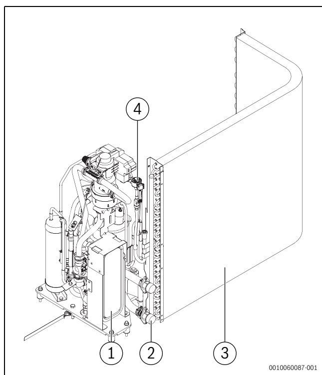
Rys. 3 Przegląd produktu, widok z tyłu
