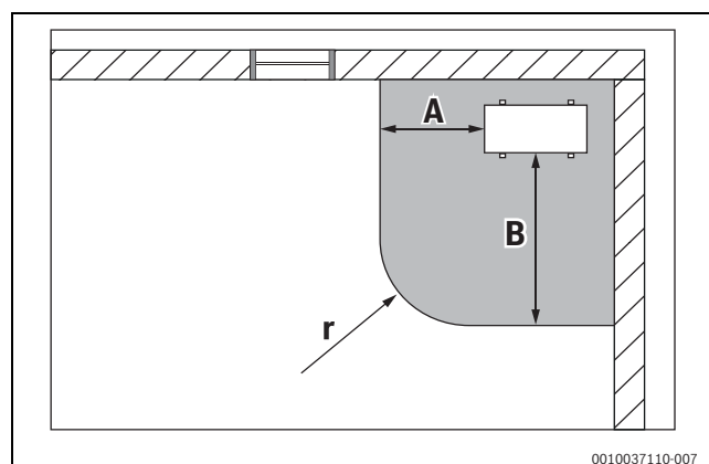
Rys. 10 Obszar bezpieczeństwa, ustawienie na ziemi w narożniku, widok z góry
