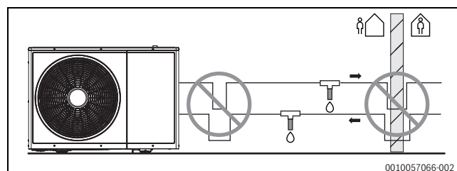
Rys. 22 Instalacja zaworu środka przeciw zamarzaniu
