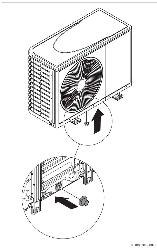
Rys. 25 Montaż przyłącza spustowego
