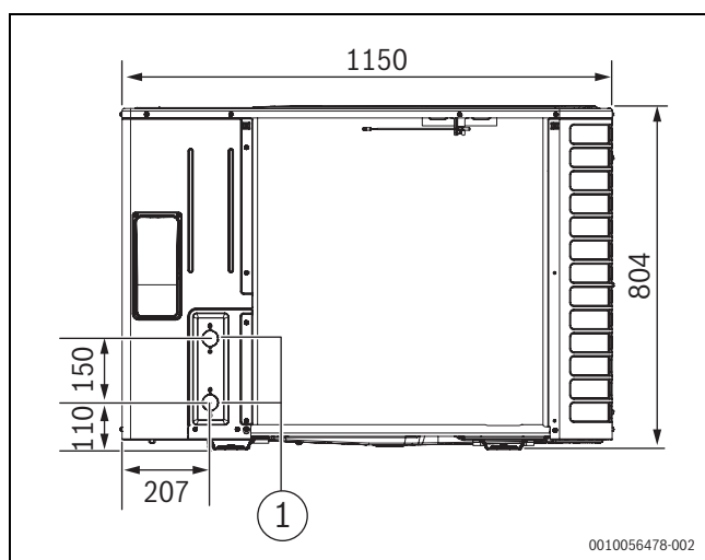
Rys. 4 Wymiary pompy ciepła i podłączenia hydrauliczne, widok z tyłu
