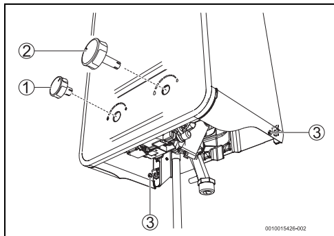
Rys. 15 Zdjąć obudowę
