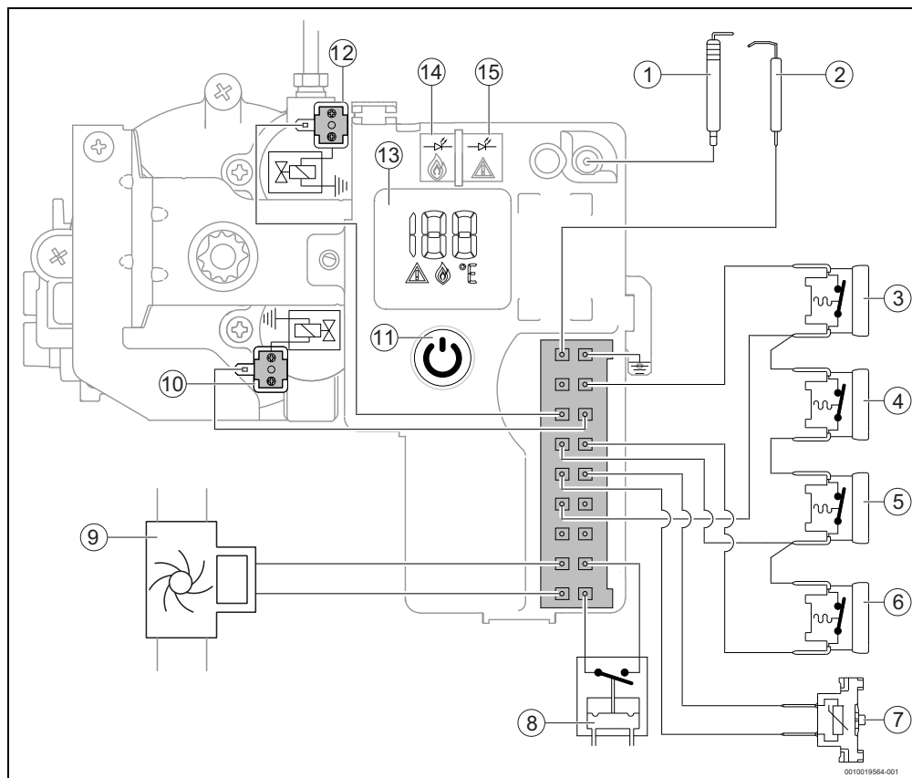
Rys. 30 Schemat elektryczny
