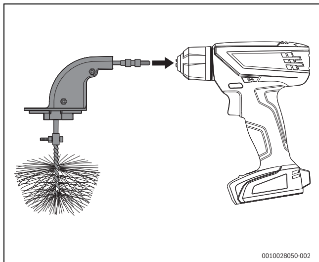
Rys. 66 Łączenie szczotki z wkrętkarką akumulatorową
