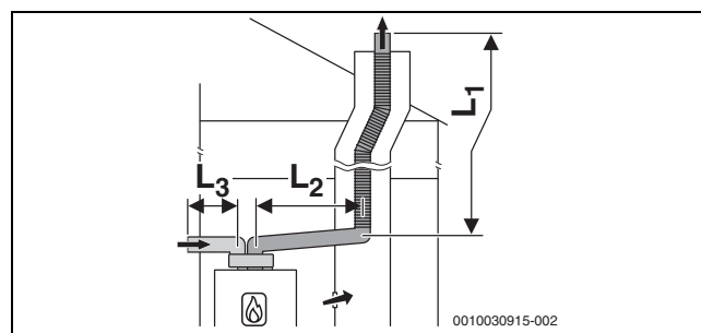
Rys. 16 Elastyczne odprowadzenie spalin wg C 53 w szachcie i instalacja powietrzno-spalinowa z odseparowanymi rurami dla dopływu powietrza i odprowadzenia spalin w pomieszczeniu zainstalowania
