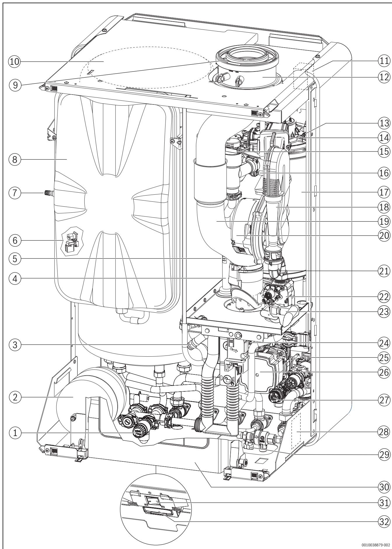
Rys. 5 Przegląd produktu
