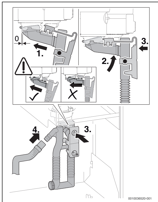
Rys. 75 Zakładanie syfonu kondensatu
