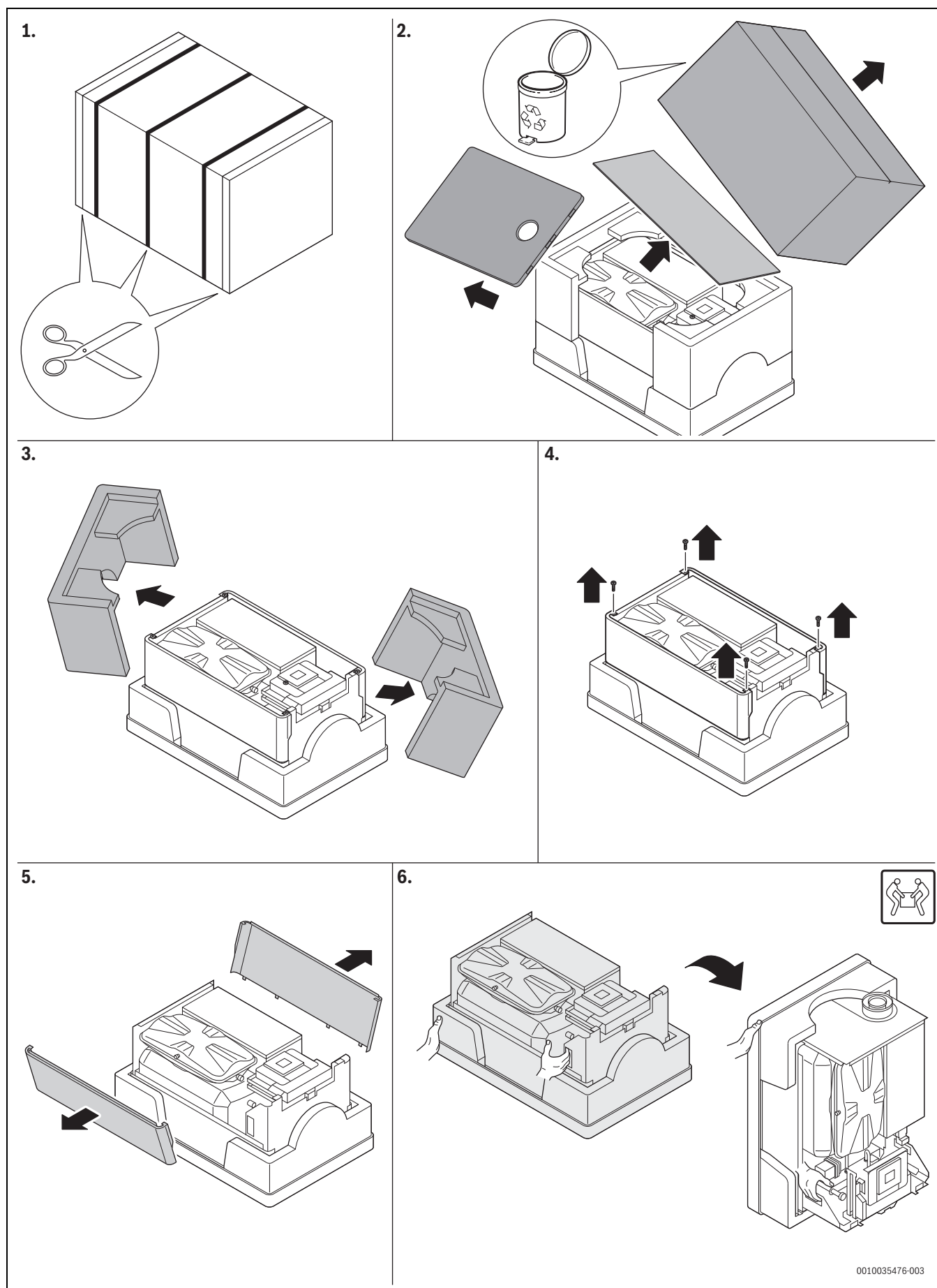
Rys. 32 Instrukcja rozpakowywania
