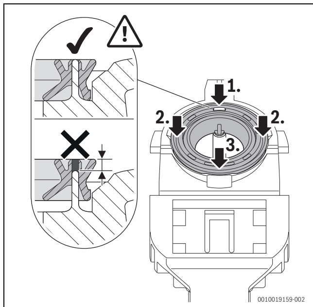
Rys. 74 Dociśnięcie uszczelki
