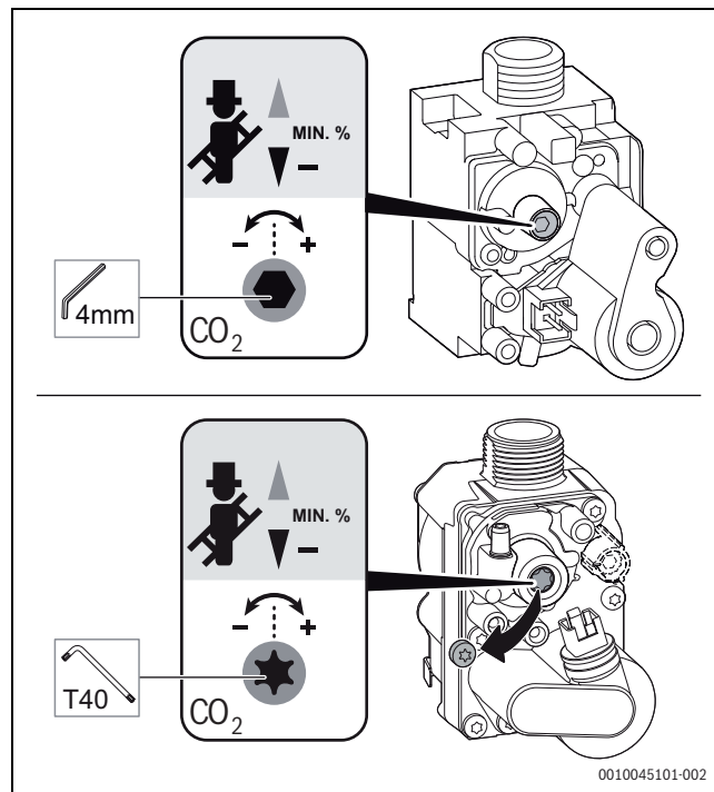
Rys. 55 Ustawianie stężenia CO 2 /O 2 dla minimalnej znamionowej mocy cieplnej
