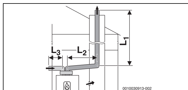
Rys. 15 Sztywne odprowadzenie spalin wg C 53 w szachcie i instalacja powietrzno-spalinowa z odseparowanymi rurami dla dopływu powietrza i odprowadzenia spalin w pomieszczeniu zainstalowania
