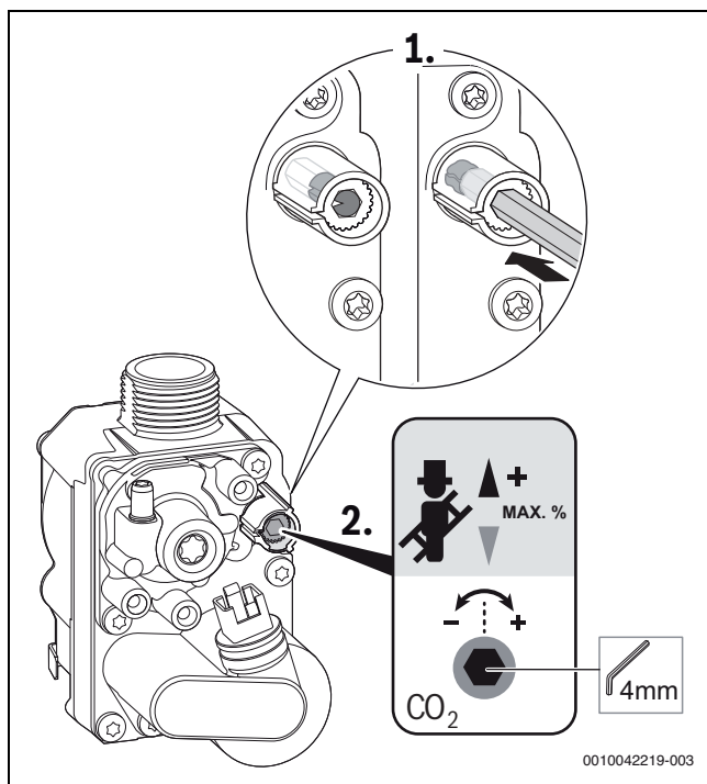
Rys. 54 Ustawianie stężenia CO 2 /O 2 dla maksymalnej znamionowej mocy cieplnej, armatura gazowa z możliwością ustawienia
