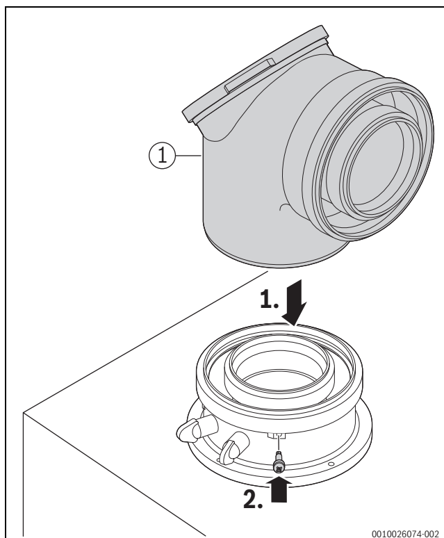
Rys. 41 Wkładanie osprzętu spalinowego i zabezpieczanie go śrubą
