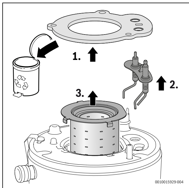
Rys. 62 Wyjmowanie palnika
