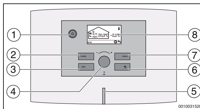
Rys. 2 Panel sterowania
