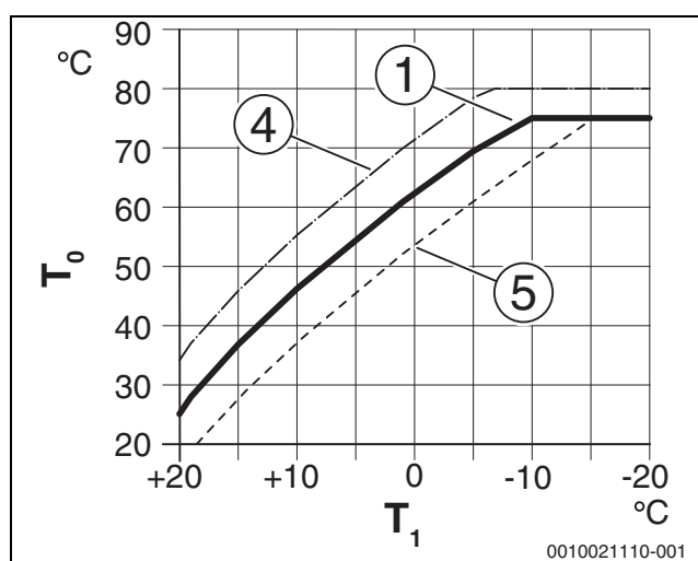
Rys. 5 Ustawienie krzywej grzania dla grzejników Przesunięcie równoległe powyżej Korekta temp.pomiesz. lub zadanej temperatury pomieszczenia
