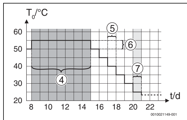
Rys. 7 Proces suszenia jastrychu z ustawieniami podstawowymi w fazie chłodzenia
