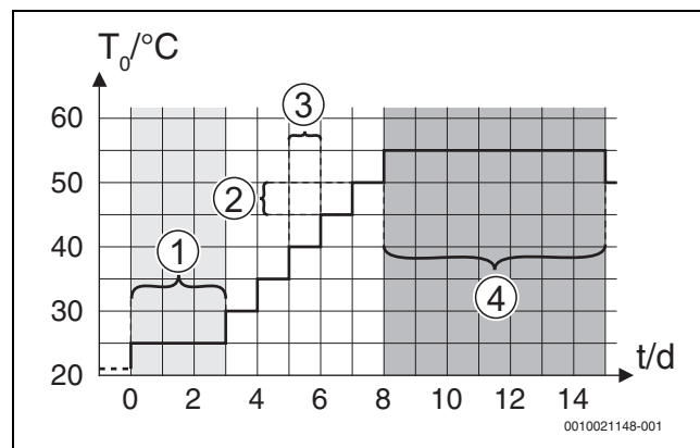
Rys. 6 Proces suszenia jastrychu z ustawieniami podstawowymi w fazie nagrzewania
