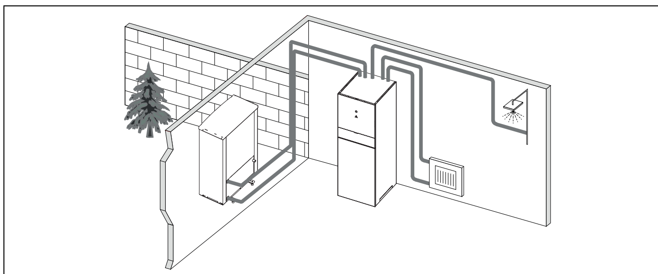
Rys. 3 Pompa ciepła Compress 7000i AW, jednostka wewnętrzna AWM/ AWMS ze zintegrowanym podgrzewaczem pojemnościowym c.w.u. i dogrzewaczem elektrycznym
