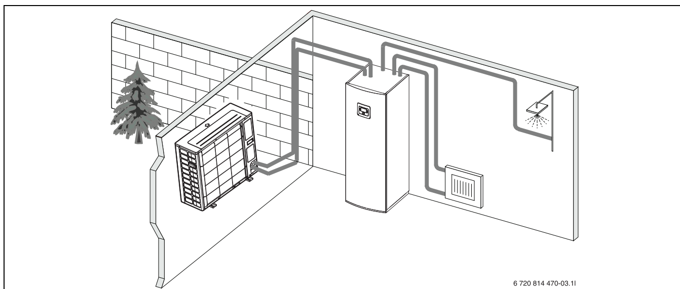
Rys. 2 Pompa ciepła (jednostka zewnętrzna), jednostka wewnętrzna AWMS/AWMSS ze zintegrowanym podgrzewaczem pojemnościowym c.w.u. i dogrzewaczem elektrycznym
