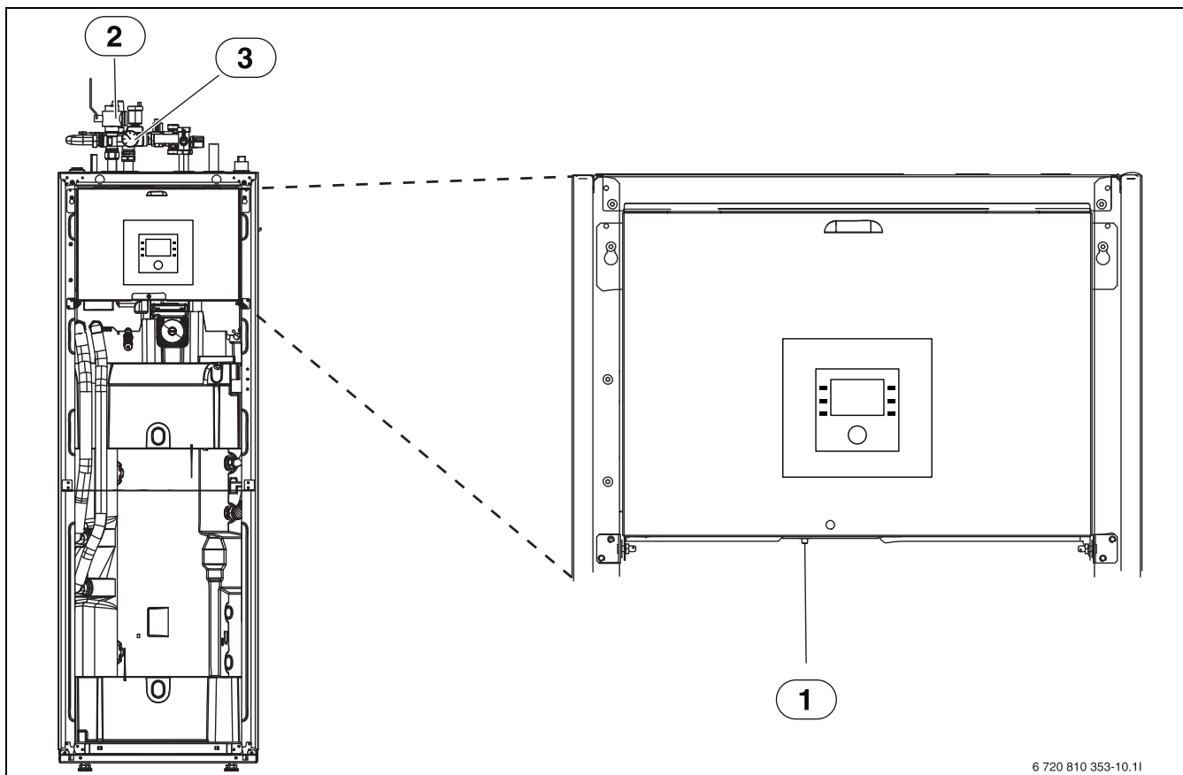
Rys. 5 Jednostka wewnętrzna AWMS / AWMSS
