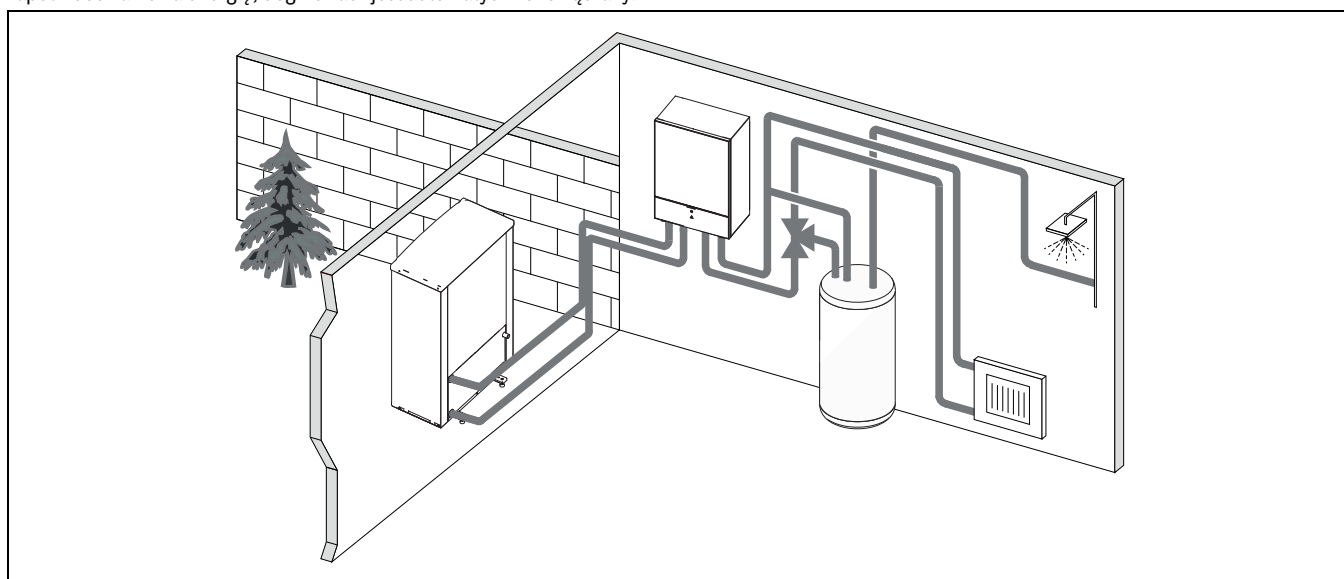
Rys. 3 Pompa ciepła Compress 7000i AW, jednostka wewnętrzna AWE z dogrzewaczem elektrycznym i zewnętrznym podgrzewaczem pojemnościowym c.w.u.
