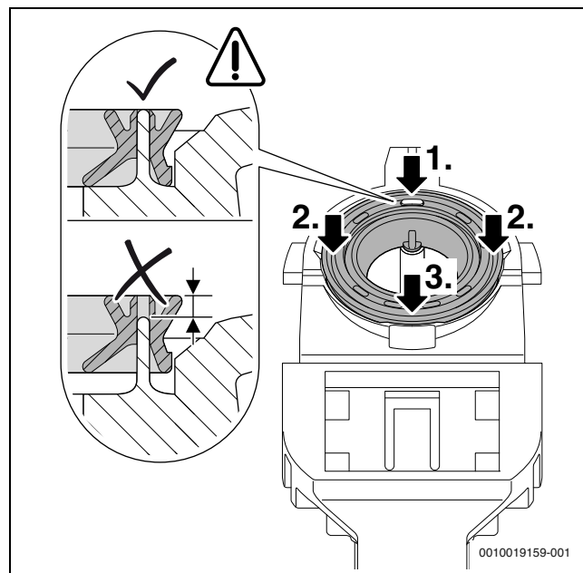
Rys. 59 Docisnięcie uszczelki
