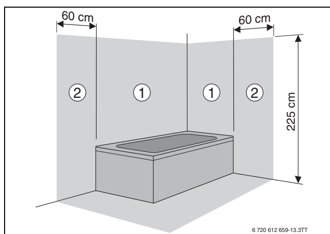
Rys. 30 Strefy ochronne
