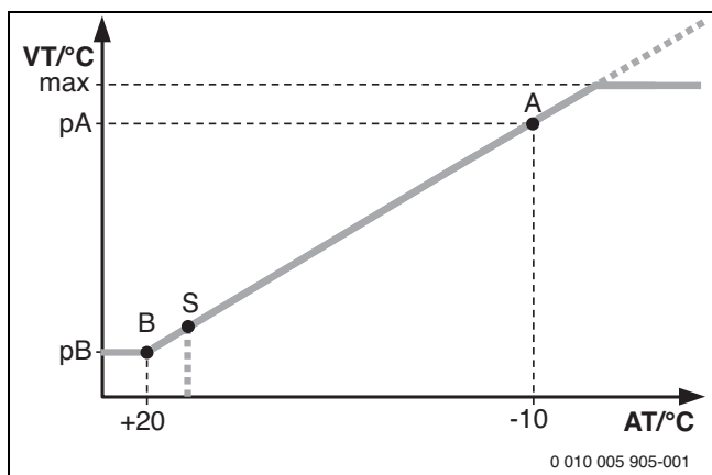
Rys. 77 Krzywa grzewcza
