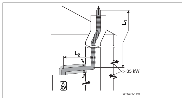
Rys. 19 Elastyczne odprowadzenie spalin w szachcie wg B 33 z zależnym od powietrza w pomieszczeniu doprowadzeniem powietrza przez koncentryczną instalację powietrzno-spalinową w pomieszczeniu zainstalowania
