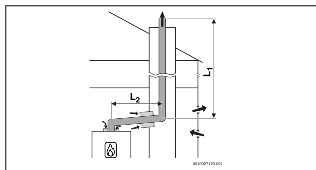
Rys. 16 Sztywne odprowadzenie spalin w szachcie wg B 23p /B 53p z zależnym od powietrza w pomieszczeniu doprowadzeniem powietrza do urządzenia i koncentryczną złączką między pomieszczeniem zainstalowania a szachtem
