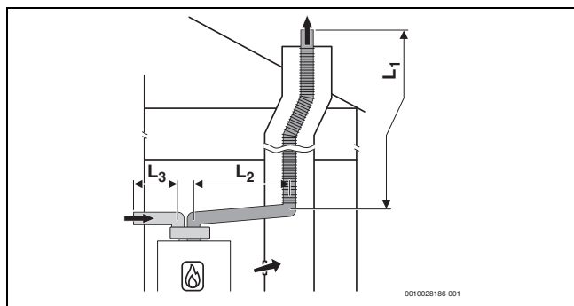
Rys. 12 Elastyczne odprowadzenie spalin wg C 53 w szachcie i instalacja powietrzno-spalinowa z odesparowanymi rurami dla dopływu powietrza i odprowadzenia spalin w pomieszczeniu zainstalowania
