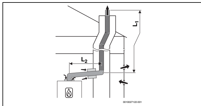
Rys. 17 Elastyczne odprowadzenie spalin w szachcie wg B 23p /B 53p z zależnym od powietrza w pomieszczeniu doprowadzeniem powietrza do urządzenia i koncentryczną złązką między pomieszczeniem zainstalowania a szachtem
