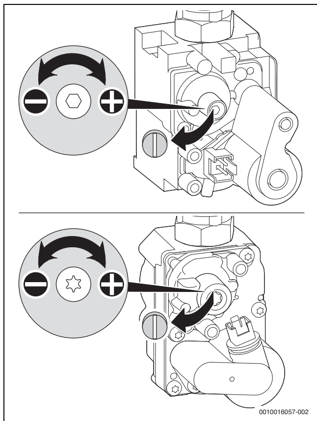
Rys. 42 Zdejmowanie plomb z śruby nastawczej
