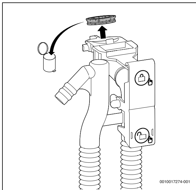
Rys. 57 Zdejmowanie uszczelki u góry na syfonie kondensatu
