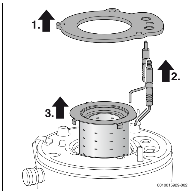
Rys. 49 Wymywanie palnika
