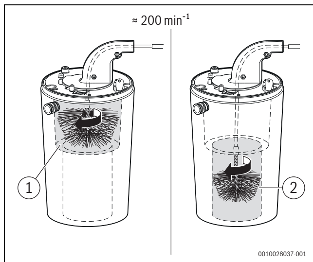
Rys. 135 Czyszczenie bloku cieplnego (ok. 200 min -1 , tylko ruch w prawo)
