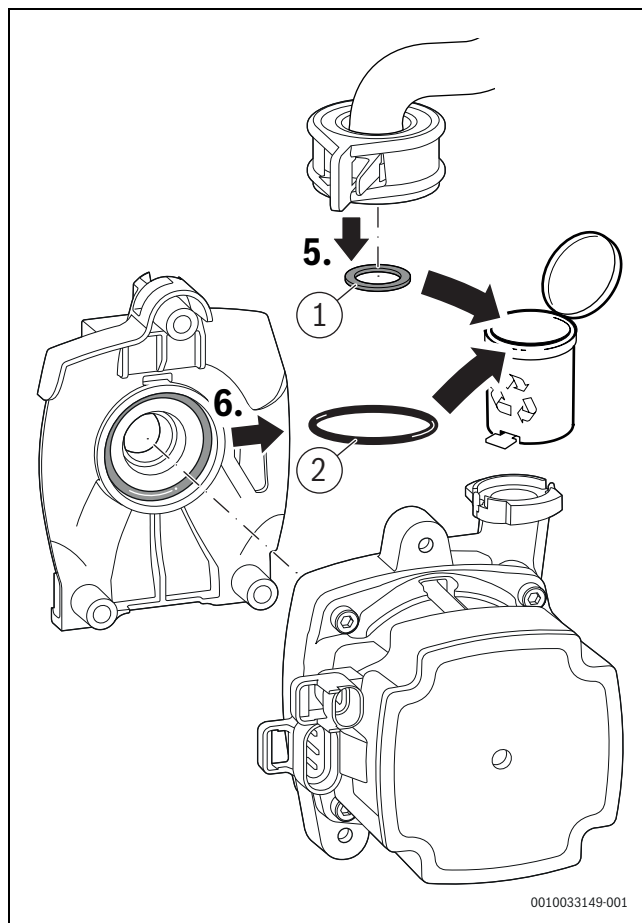
Rys. 144 Utylizacja uszczelki
