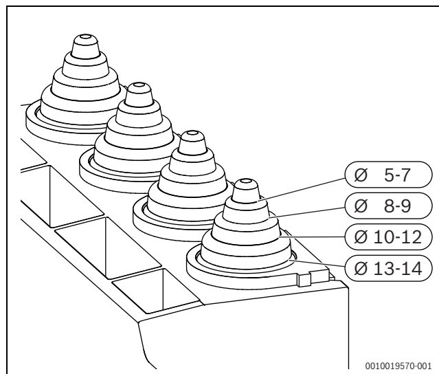
Rys. 91 Dopasowywanie uchwytu odciążającego do średnicy kabla
