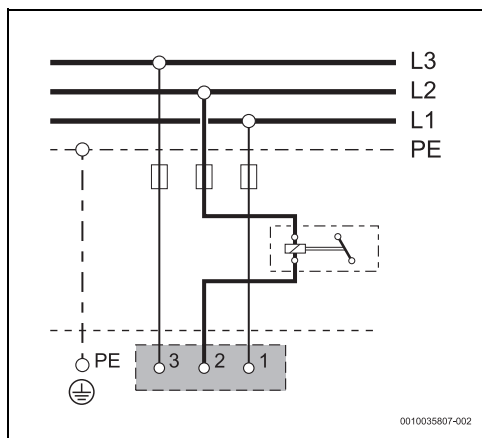
Rys. 42 Schemat elektryczny
