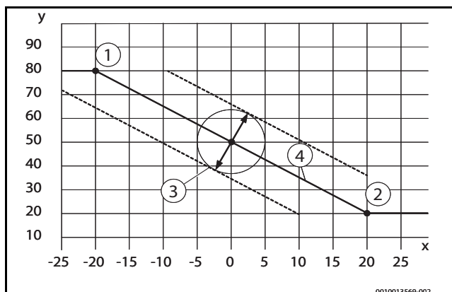
Rys. 4 Krzywa grzania przy regulacji wg temperatury zewnętrznej
