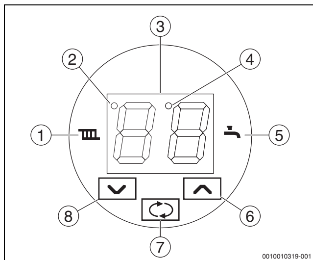
Rys. 3 Panel obsługi
