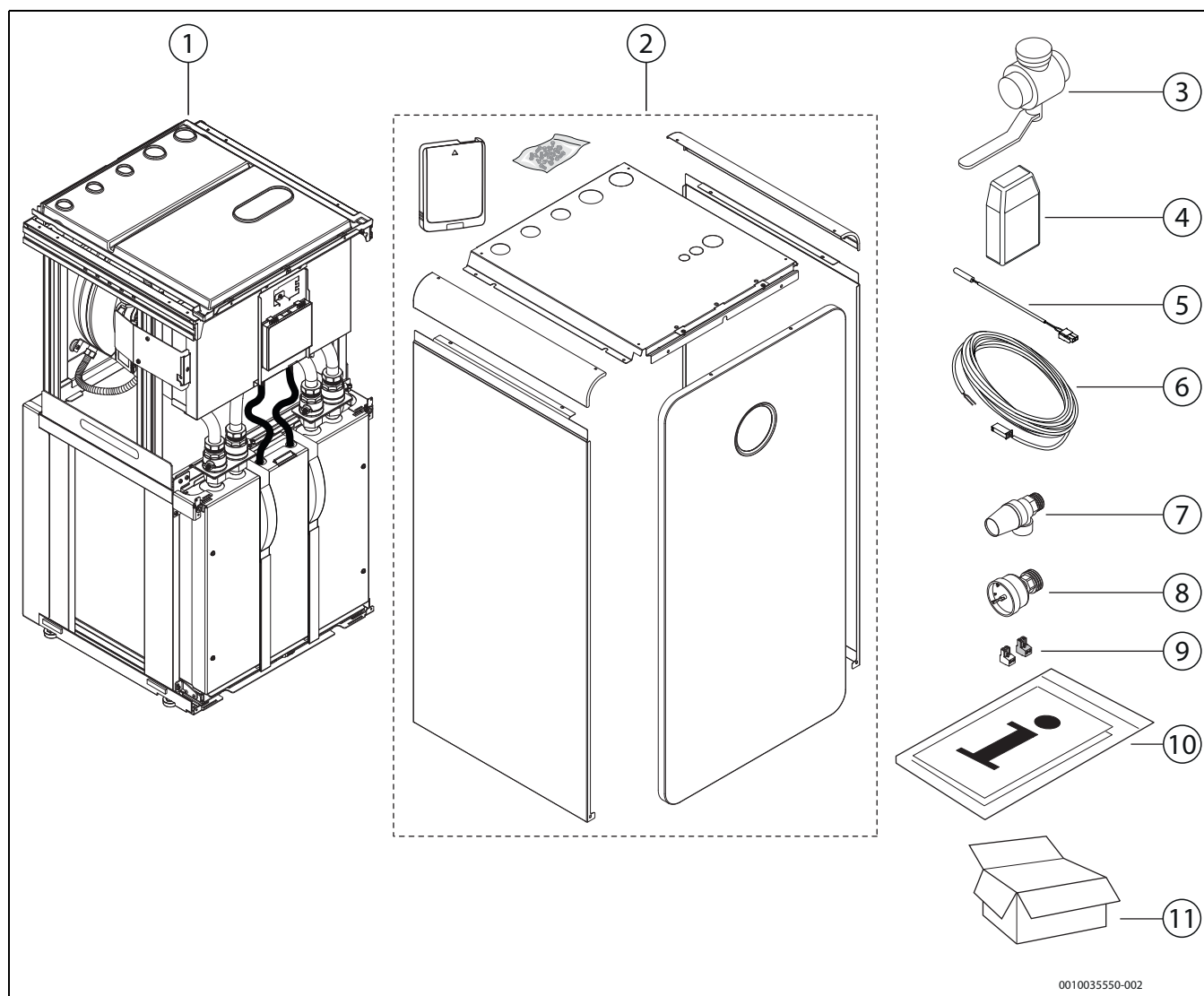
Rys. 2 Zakres dostawy
