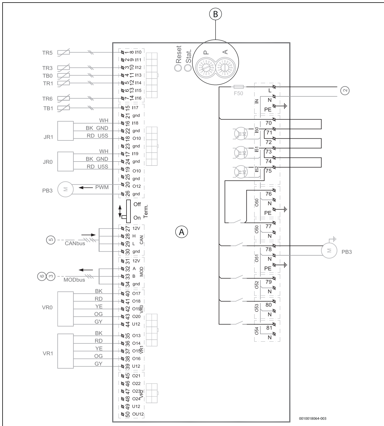
Rys. 53 Schemat elektryczny modułu I/O
