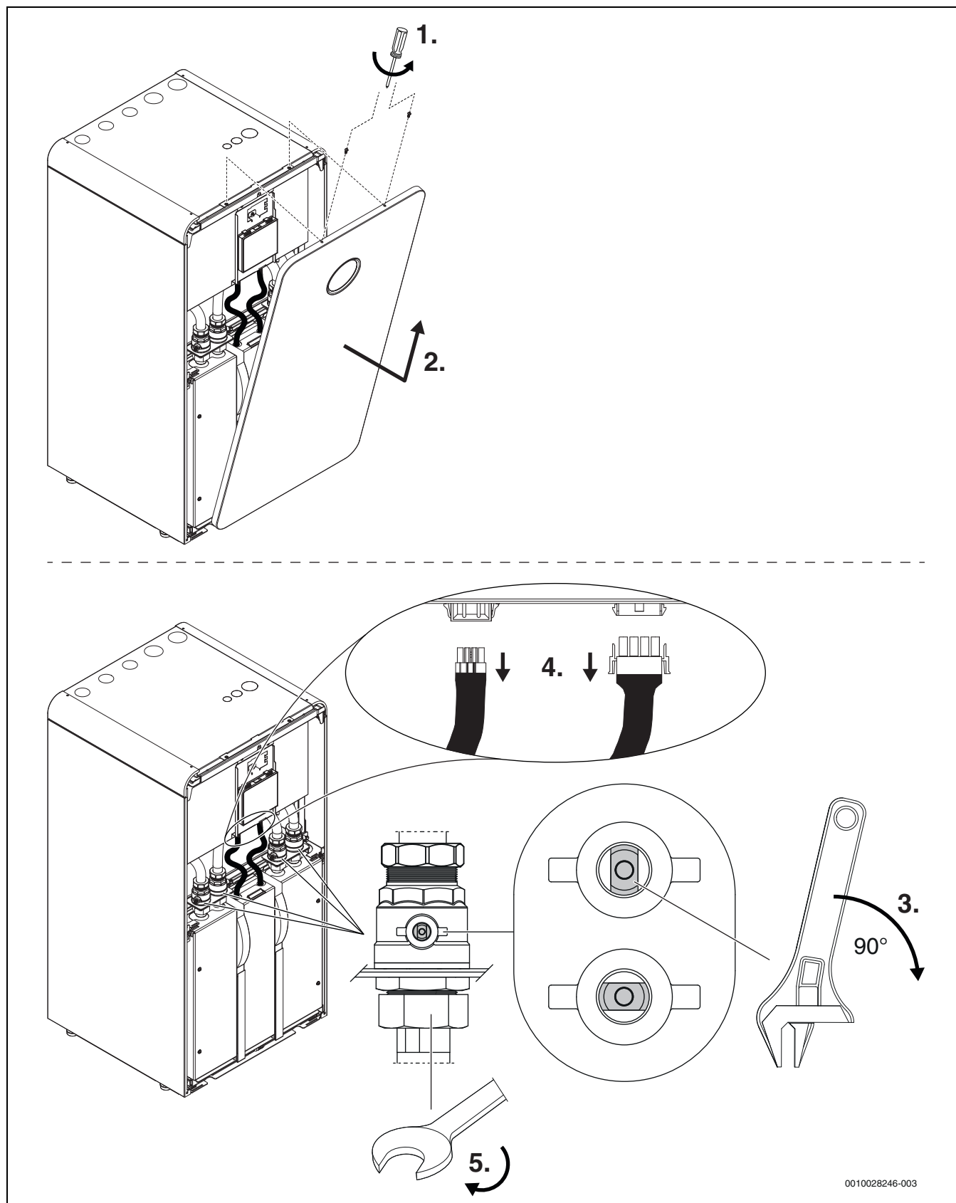
Rys. 39 Dostępność obiegu chłodniczego do zaawansowanych prac montażowych i konserwacyjnych, krok 1–5
