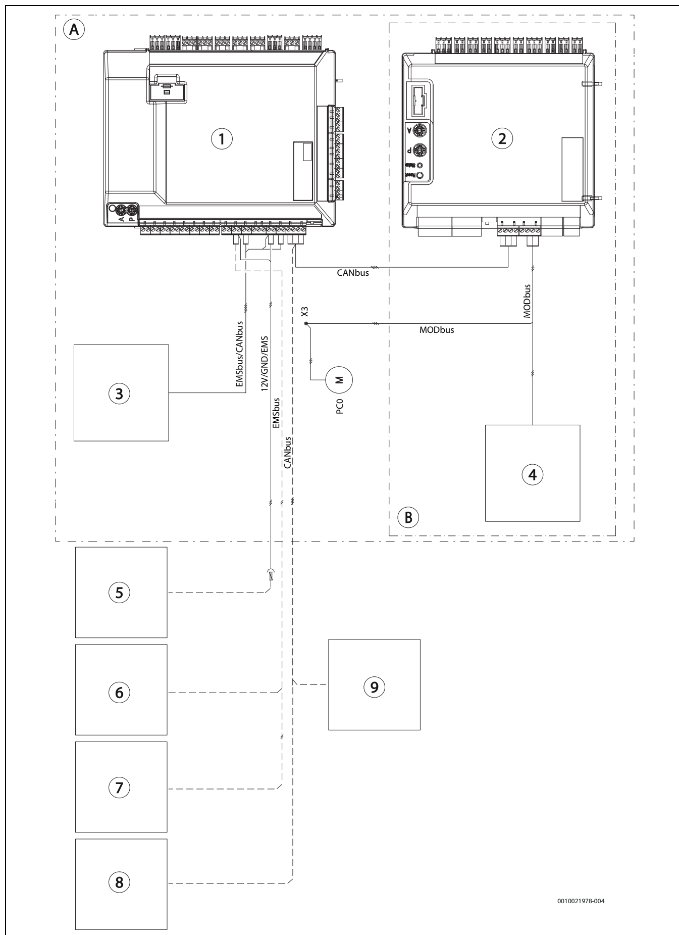
Rys. 54 Przegląd CAN-, EMS-, MOD-BUS
