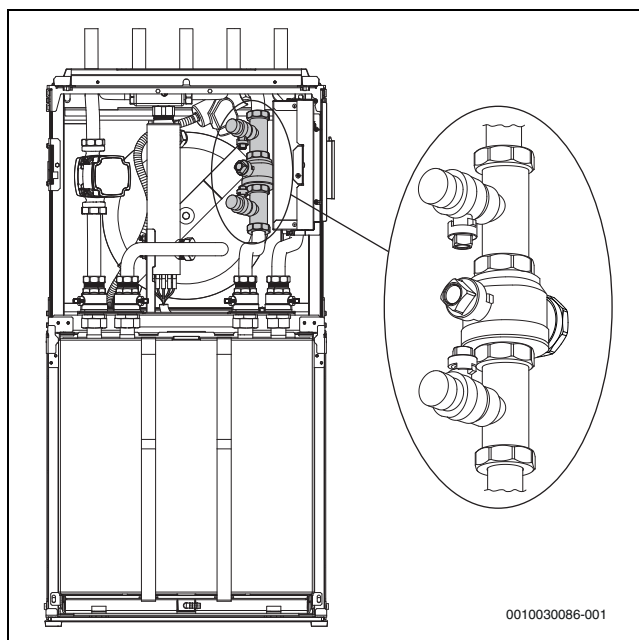
Rys. 27 Urządzenie napełniające
