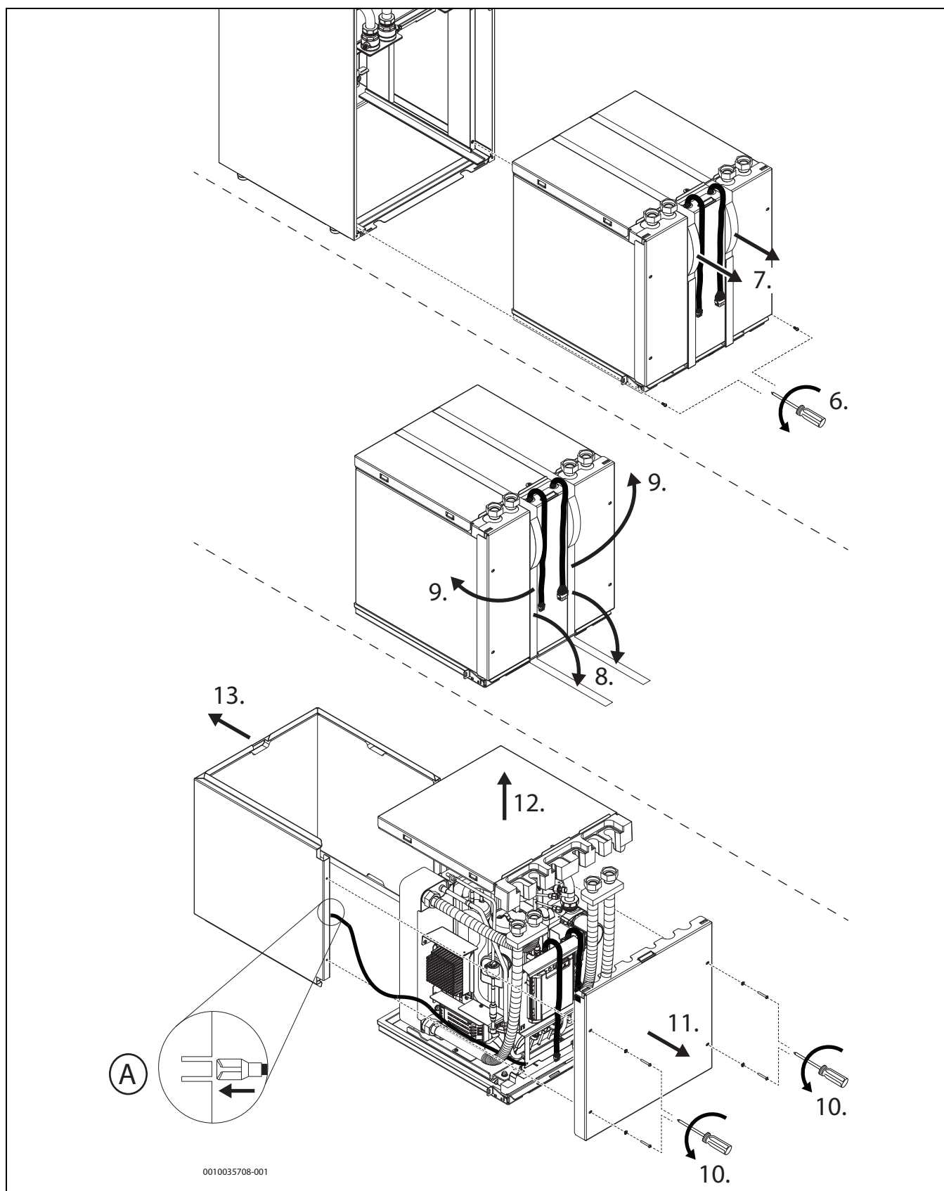
Rys. 40 Dostępność obiegu chłodniczego do zaawansowanych prac montażowych i konserwacyjnych, krok 6–13
