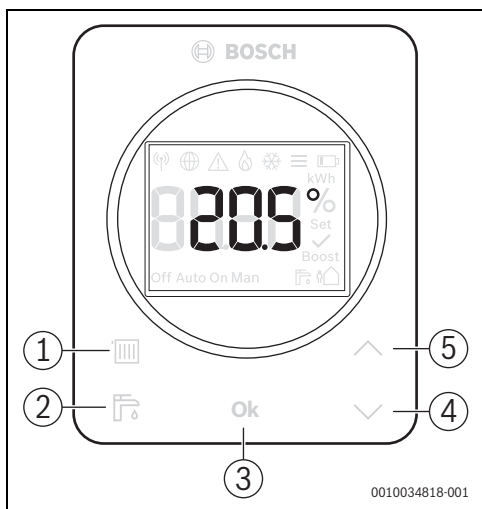
Rys. 1 Elementy obsługowe
