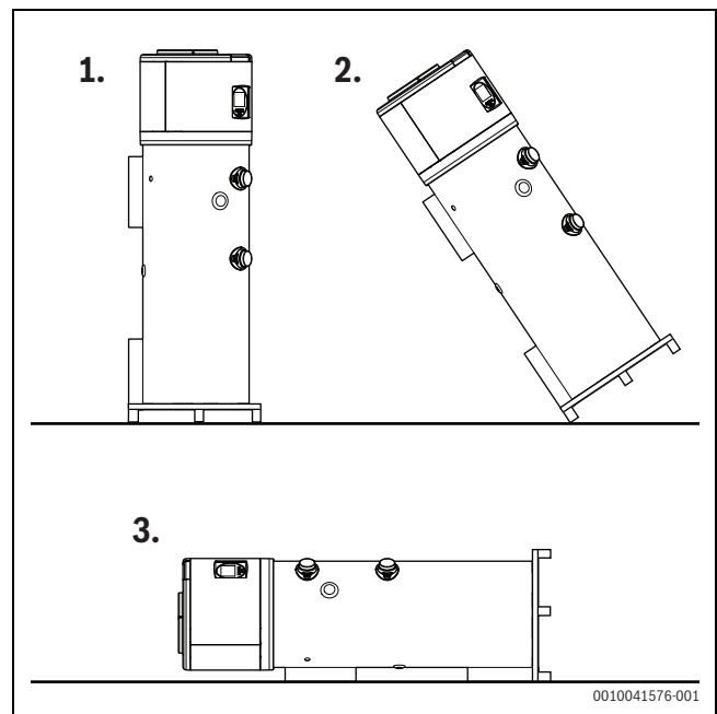
Rys. 5 Pochylenie urządzenia
