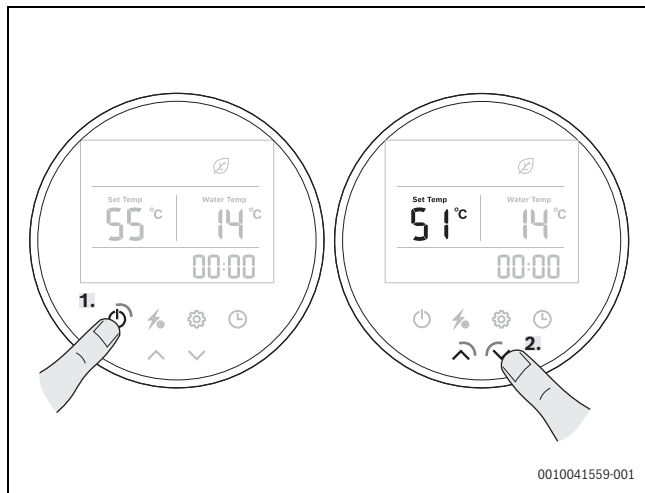
Rys. 18 Ustawienie temperatury
