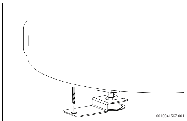
Rys. 8 Wspornik mocujący
