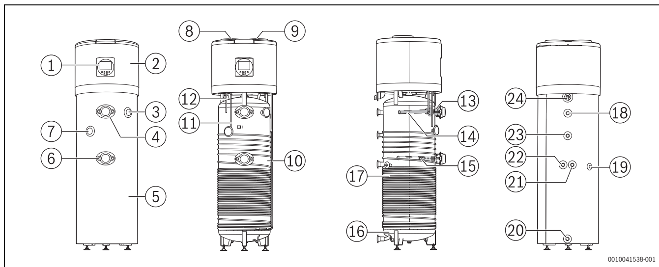
Rys. 3 Przegląd produktu
