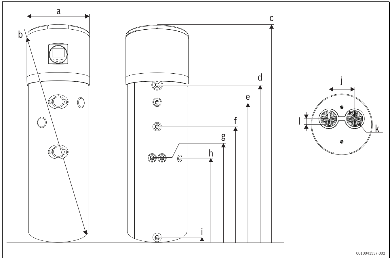
Rys. 2 Wymiary urządzenia
