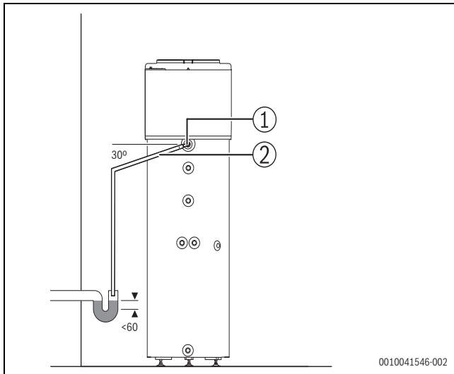
Rys. 12 Podłączenie odprowadzenia kondensatu
