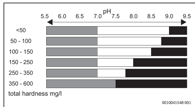
Rys. 13 Jakość wody
