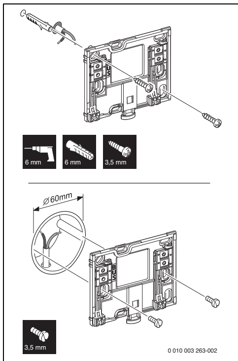
Rys. 4 Instalacja cokołu
