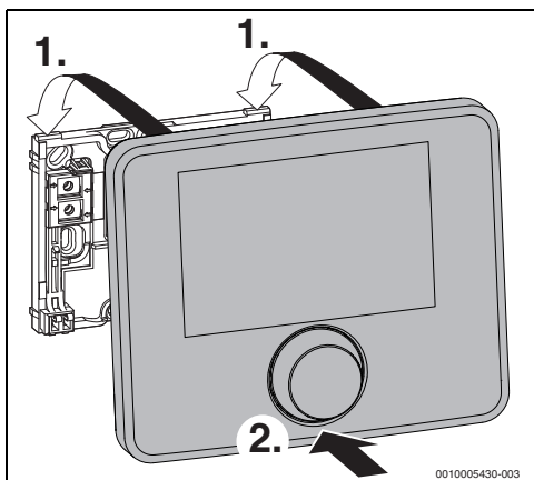
Rys. 5 Zawieszenie sterownika
