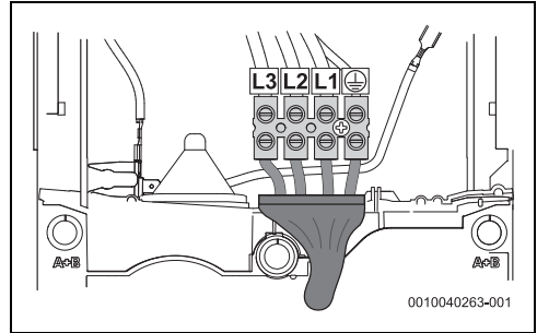
Rys. 50 Przyłącze od dołu na krótkie kable
