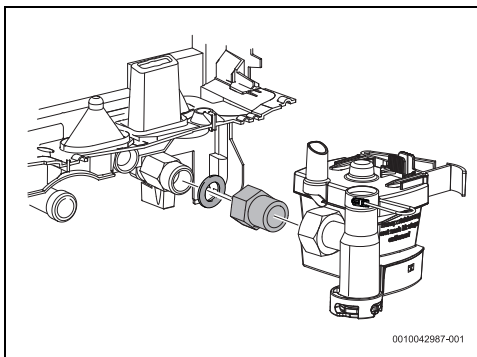
Rys. 27 Dodatkowa tuleja
