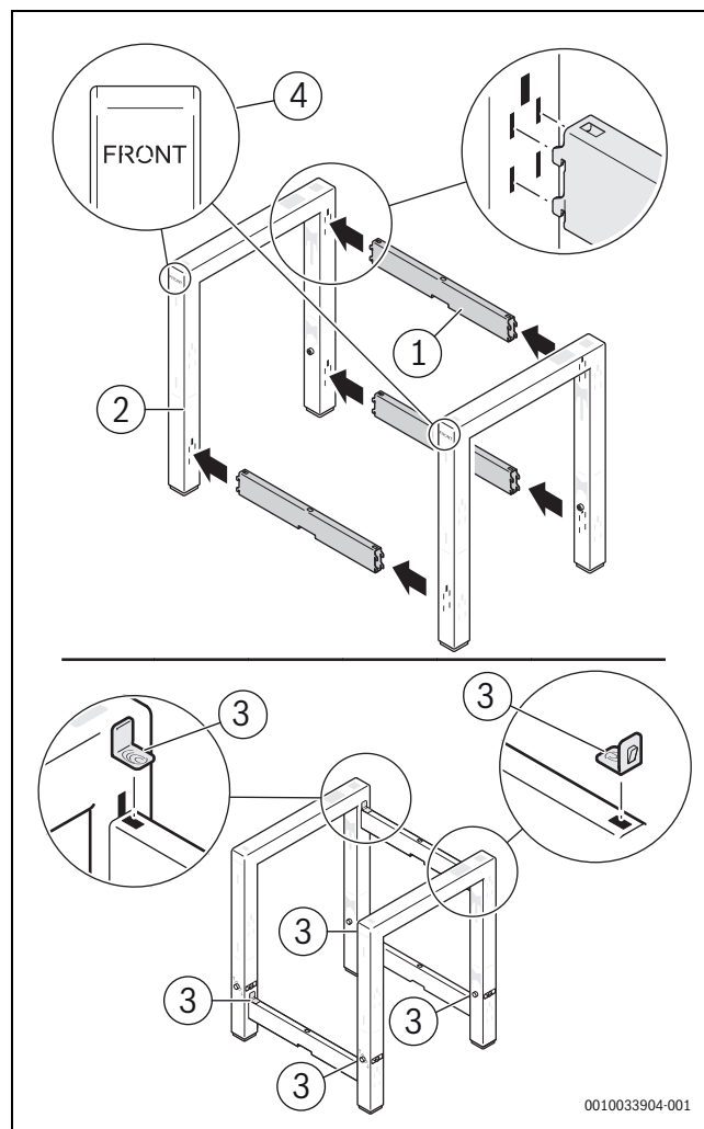
Rys. 8 Montaż ramy
