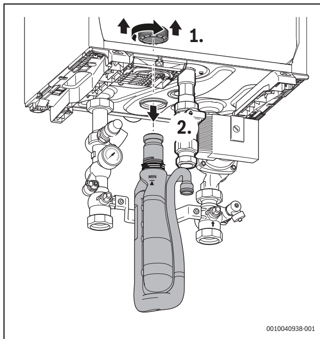
Rys. 43 Wymontować syfon kotła
