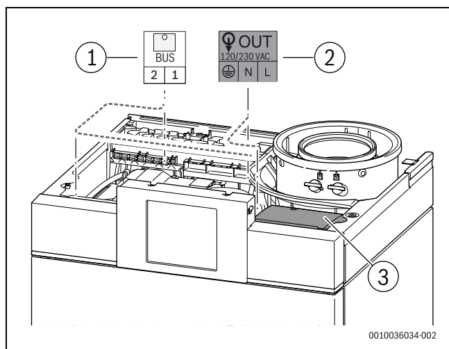
Rys. 29 Montaż modułu funkcyjnego
