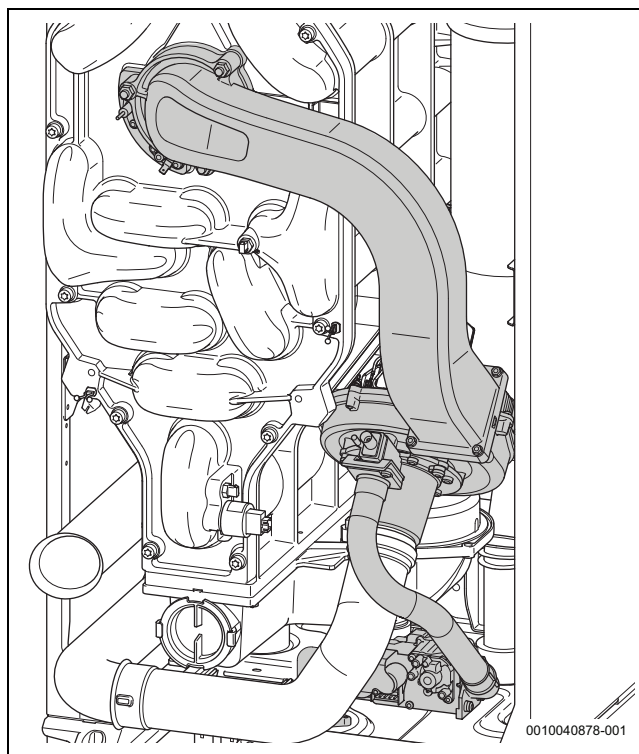
Rys. 34 Kontrola drogi gazowej
