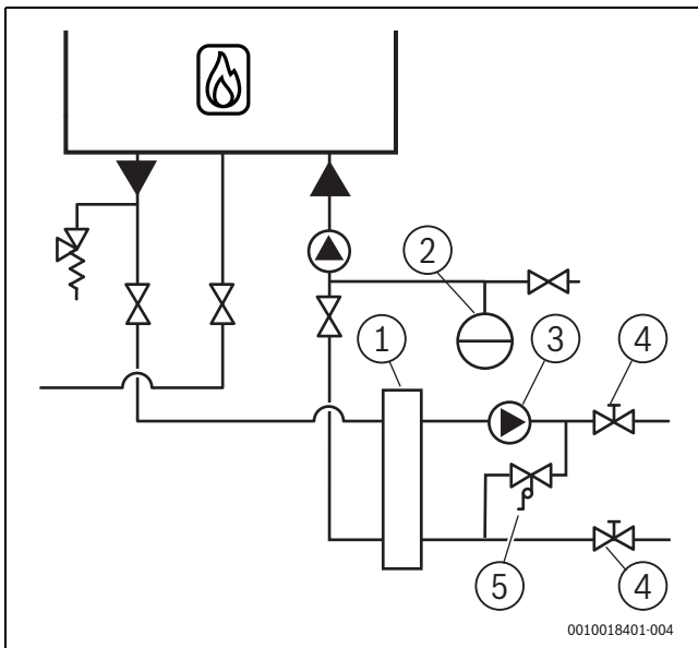
Rys. 19 Konfiguracja ze sprzęgłem hydraulicznym
