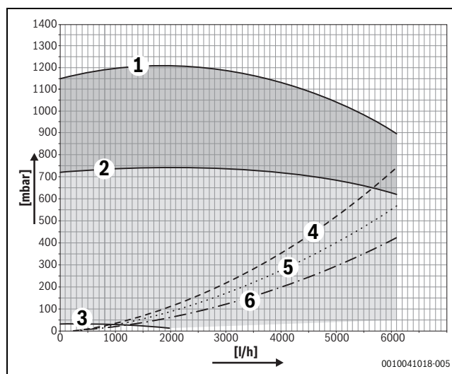
Rys. 52 Ciśnienie dyspozycyjne pompy 100kW-150kW
