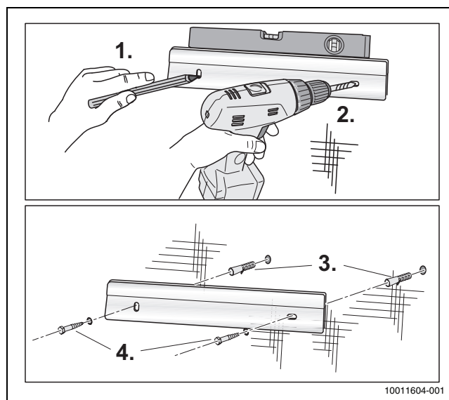
Rys. 11 Instalowanie szyny montażowej w ścianie betonowej
