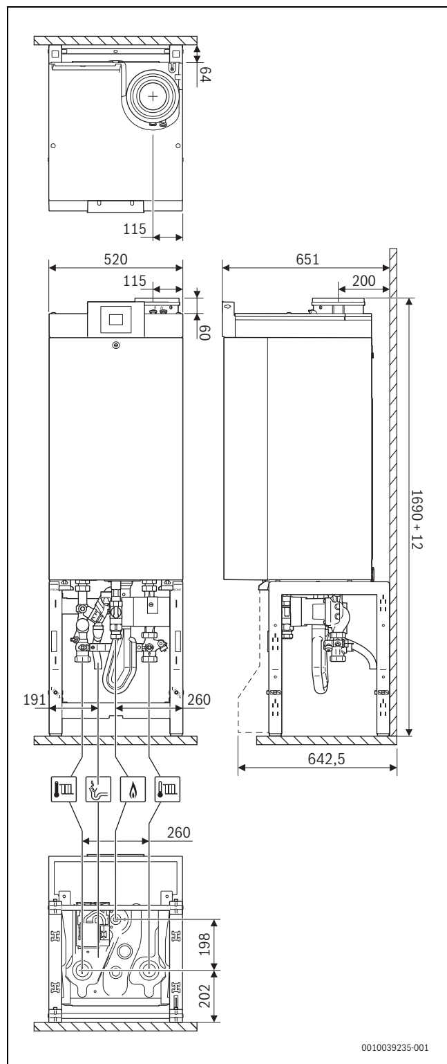
Rys. 4 Wymiary kotła stojącego na ramie podstawy [mm]
