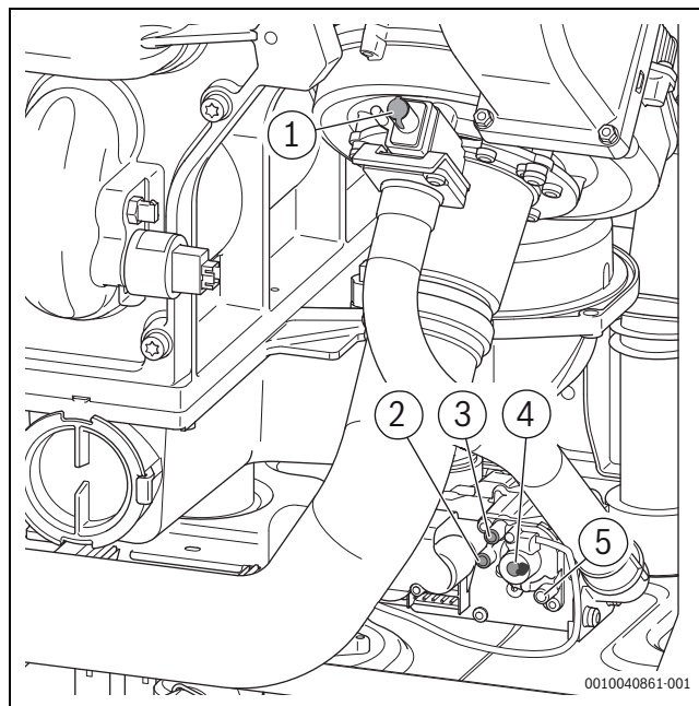
Rys. 31 Omówienie króćca pomiarowego i śruby nastawczej
