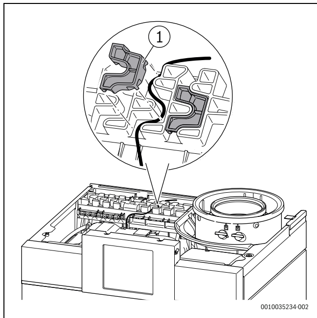
Rys. 24 Ustawianie przewodu łączącego i kanału kablowego
