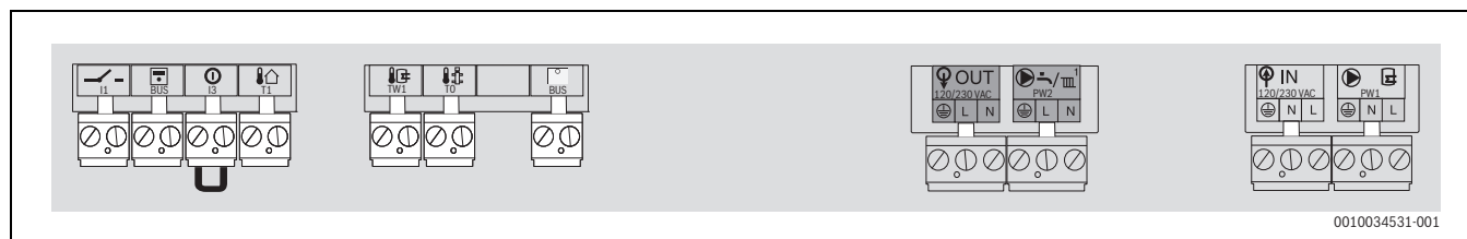
Rys. 23 Omówienie listwy wtykowej
