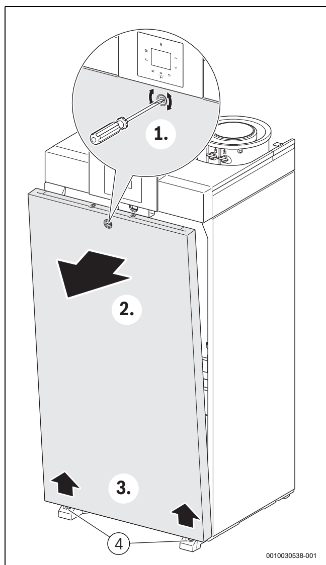
Rys. 6 Otwieranie ścianki przedniej
