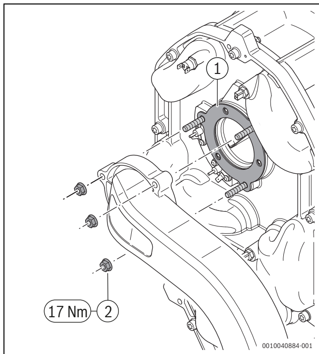
Rys. 45 Montaż rury mieszania gazu z powietrzem
