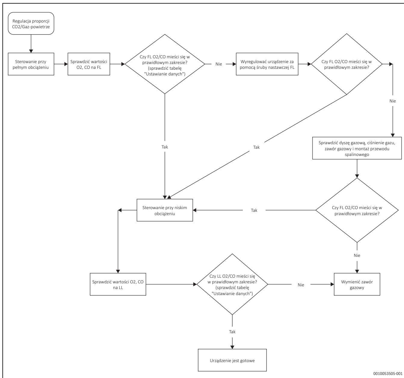
Rys. 33 Schemat blokowy instrukcji nastawy
