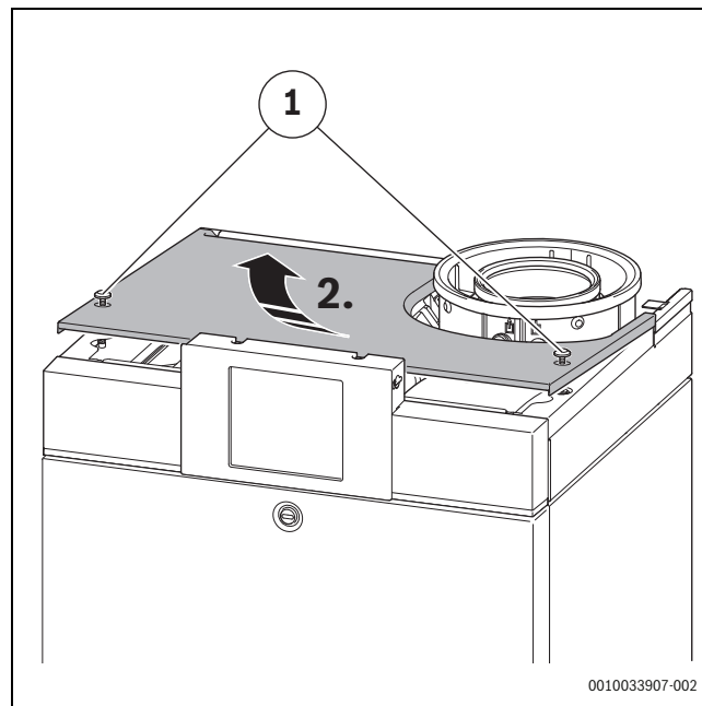
Rys. 22 Otwieranie pokrywy
