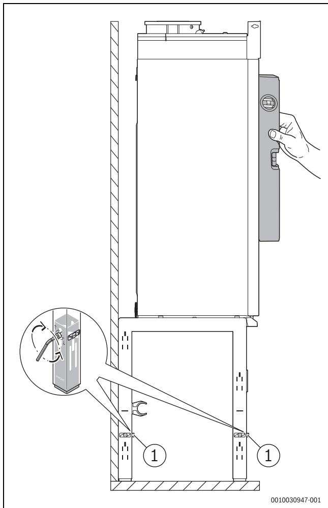
Rys. 10 Wyrównać położenie kotła na ramie.
