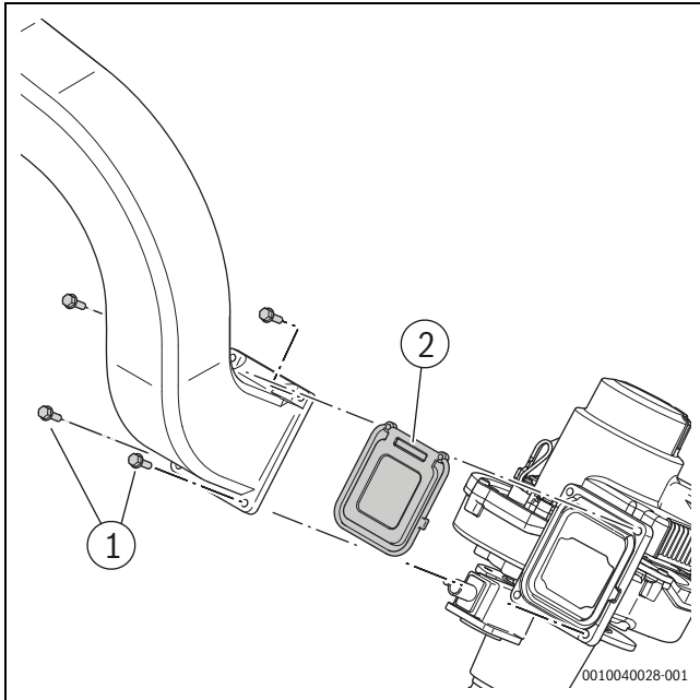
Rys. 49 Wymiana zaworu zwrotnego spalin
