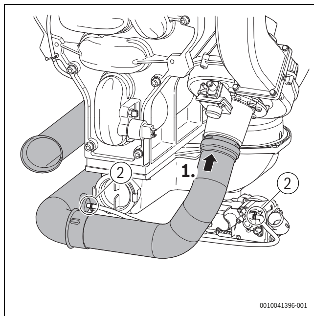
Rys. 46 Sprawdzić połączenia węża kompensacji ciśnienia.
