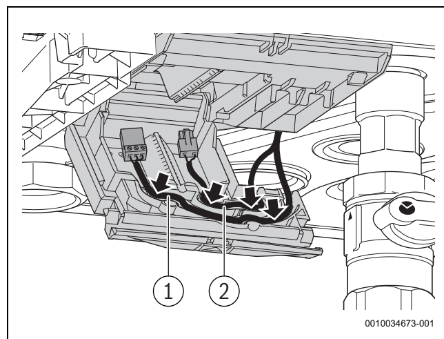
Rys. 26 Podłączanie pompy
