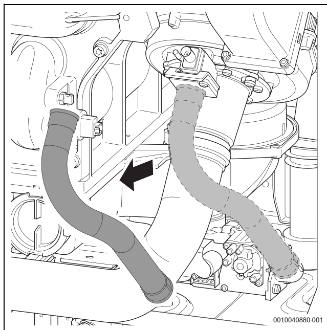
Rys. 36 Wymontować wąż gazu
