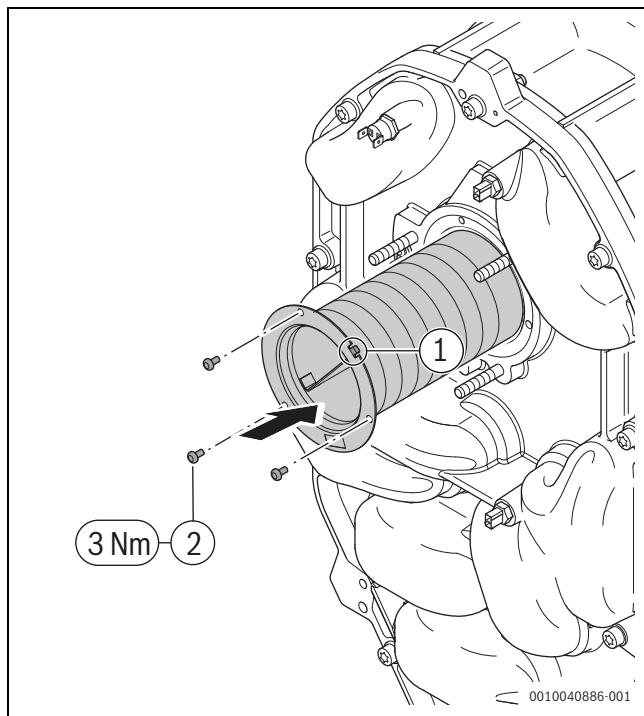
Rys. 44 Montaż palnika
