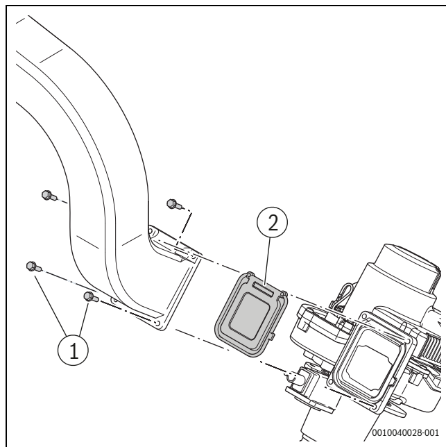
Rys. 39 Czyszczenie zaworu zwrotnego gazu/powietrza
