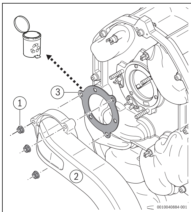
Rys. 38 Zdemontować rurę mieszania gazu z powietrzem
