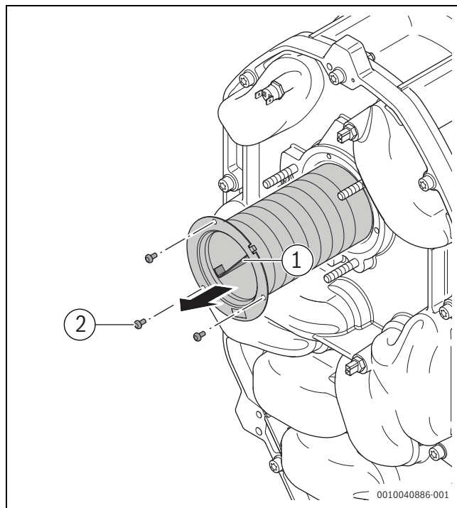
Rys. 40 Demontaż palnika
