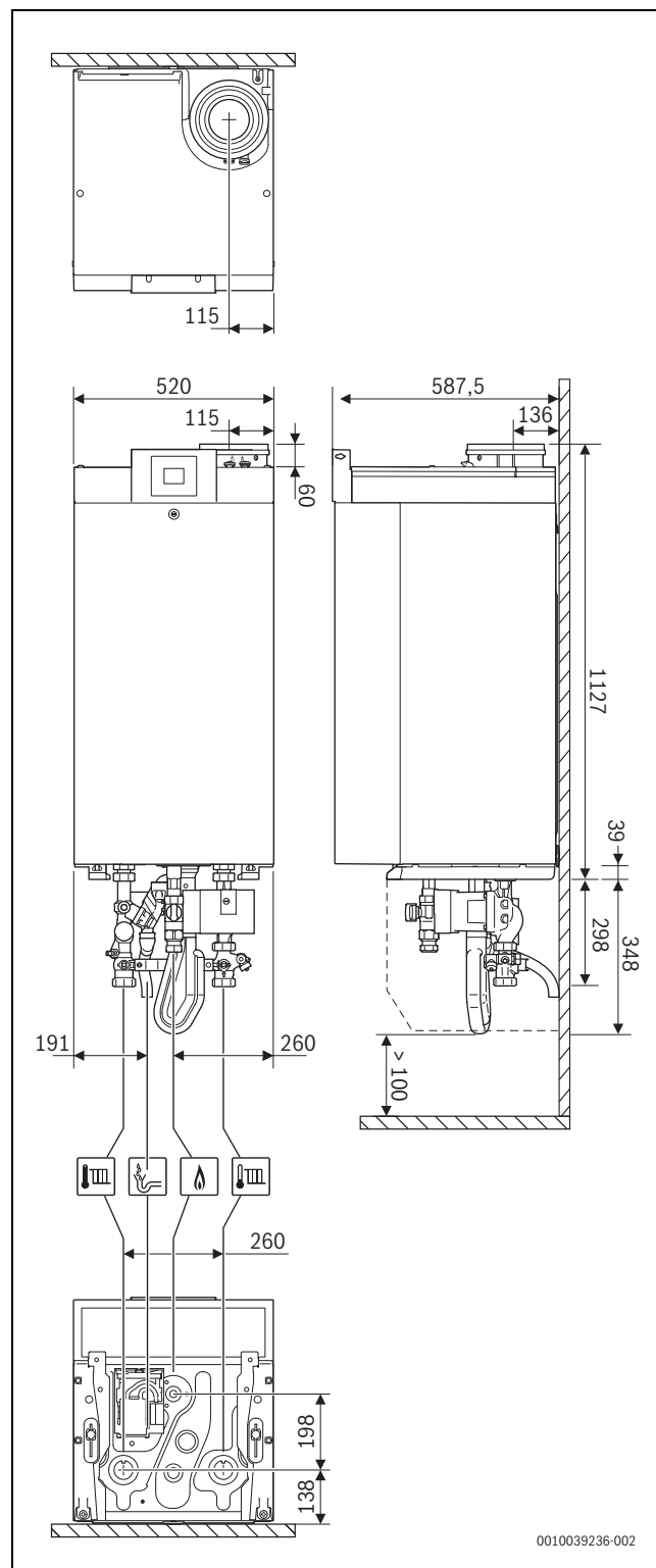
Rys. 5 Wymiary kotła wiszącego na ścianie [mm]
