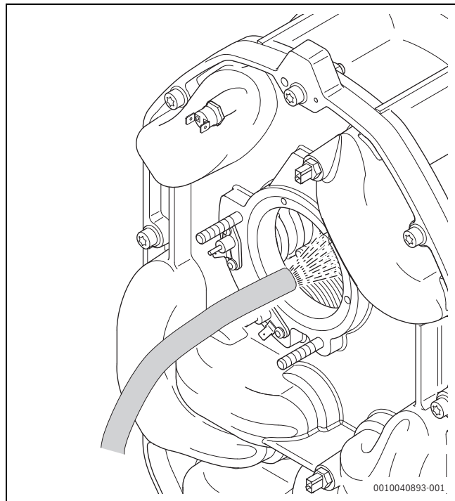
Rys. 41 Przepłukiwanie wymiennika ciepła
