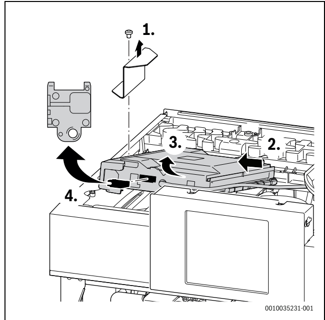
Rys. 50 Wymiana wtyczki kodującej
