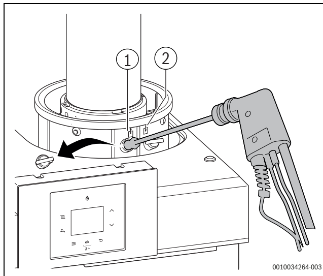
Rys. 32 Wyjąć korek z wylotu spalin
