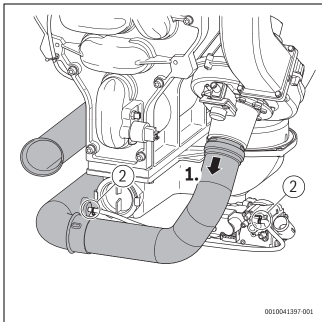
Rys. 37 Wymontowywanie kolektora powietrza
