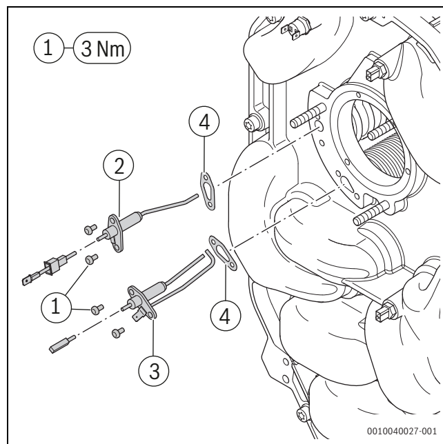
Rys. 48 Wymiana elektrody jonizacyjnej i zapłonowej
