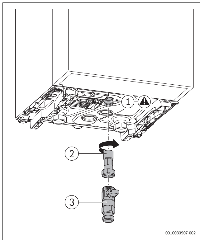
Rys. 13 Montaż zaworu gazowego
