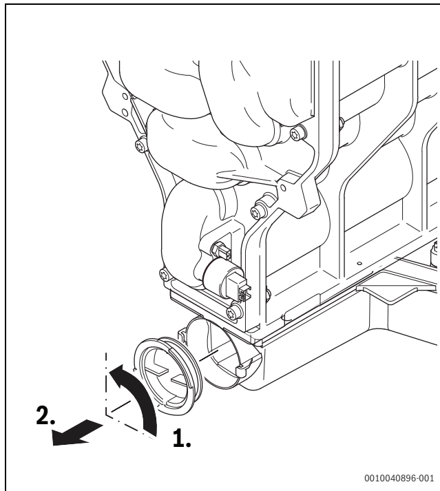
Rys. 42 Otworzyć pokrywę tacy skroplin.
