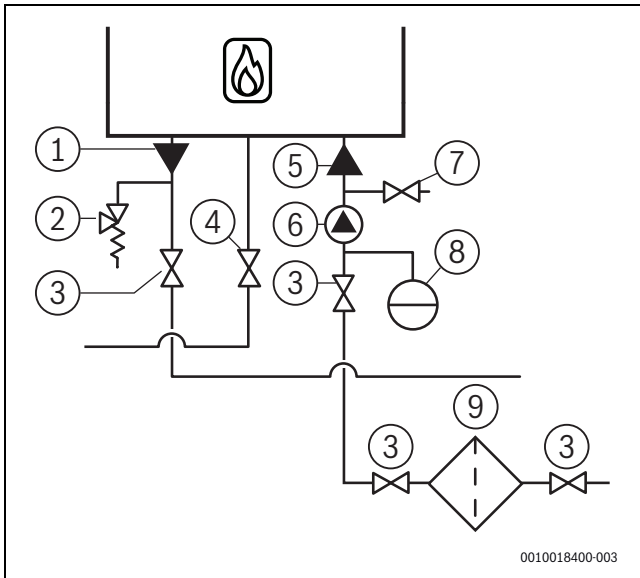
Rys. 18 Podłączenie rur wody grzejnej
