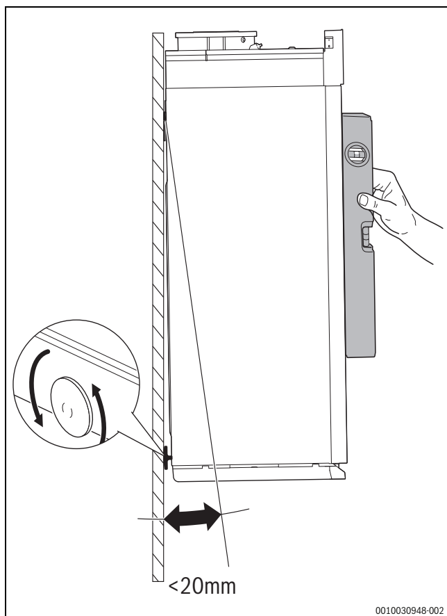
Rys. 12 Wyrównywanie położenia kotła na ścianie
