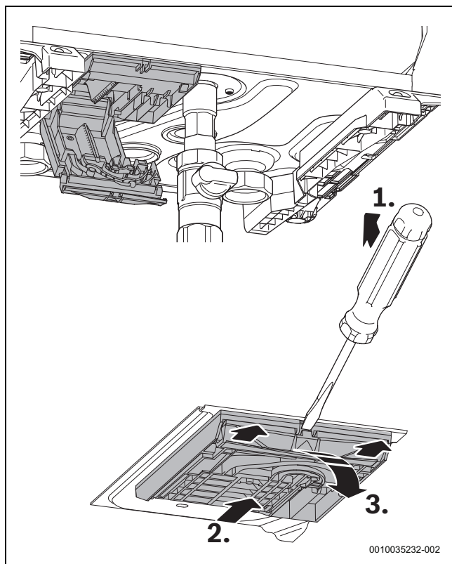
Rys. 25 Otwieranie skrzynki pompy.
