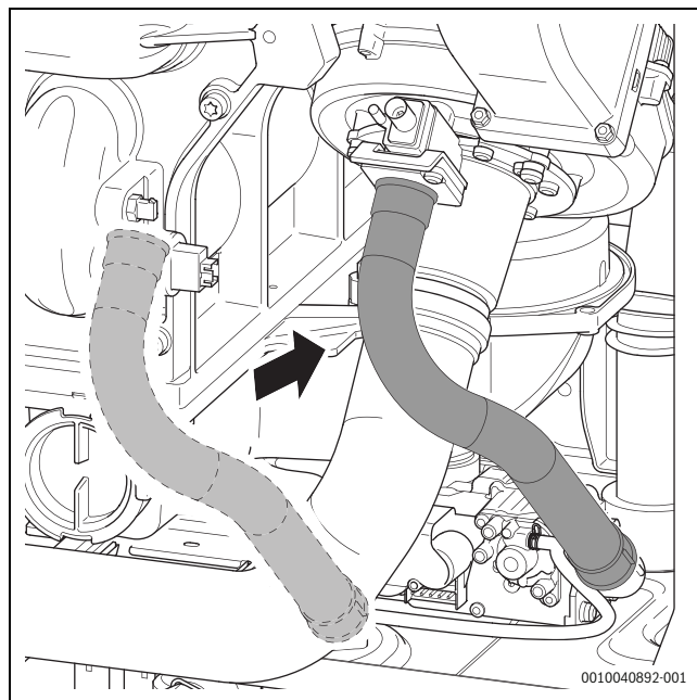
Rys. 47 Montaż węża gazu
