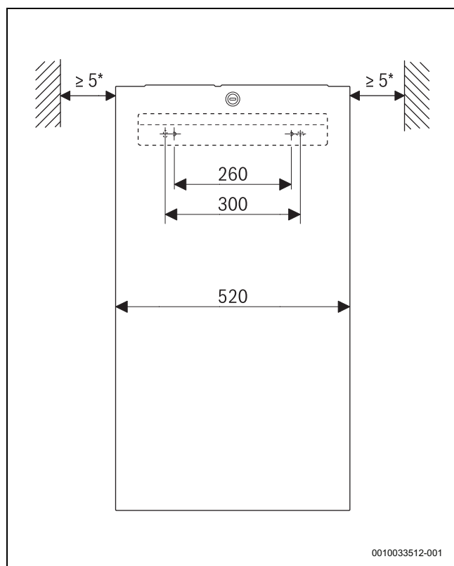
Rys. 3 Widok z przodu [mm]
