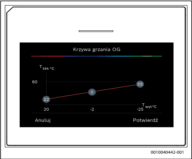
Rys. 1 Ekran startowy do ustawiania krzywej grzewczej dla rodzaju regulacji według temperatury zewnętrznej z punktem początkowym (i punktem komfortu)
