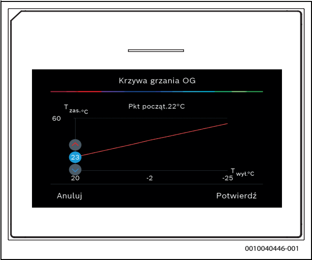
Rys. 3 Dostosowanie punktu początkowego
