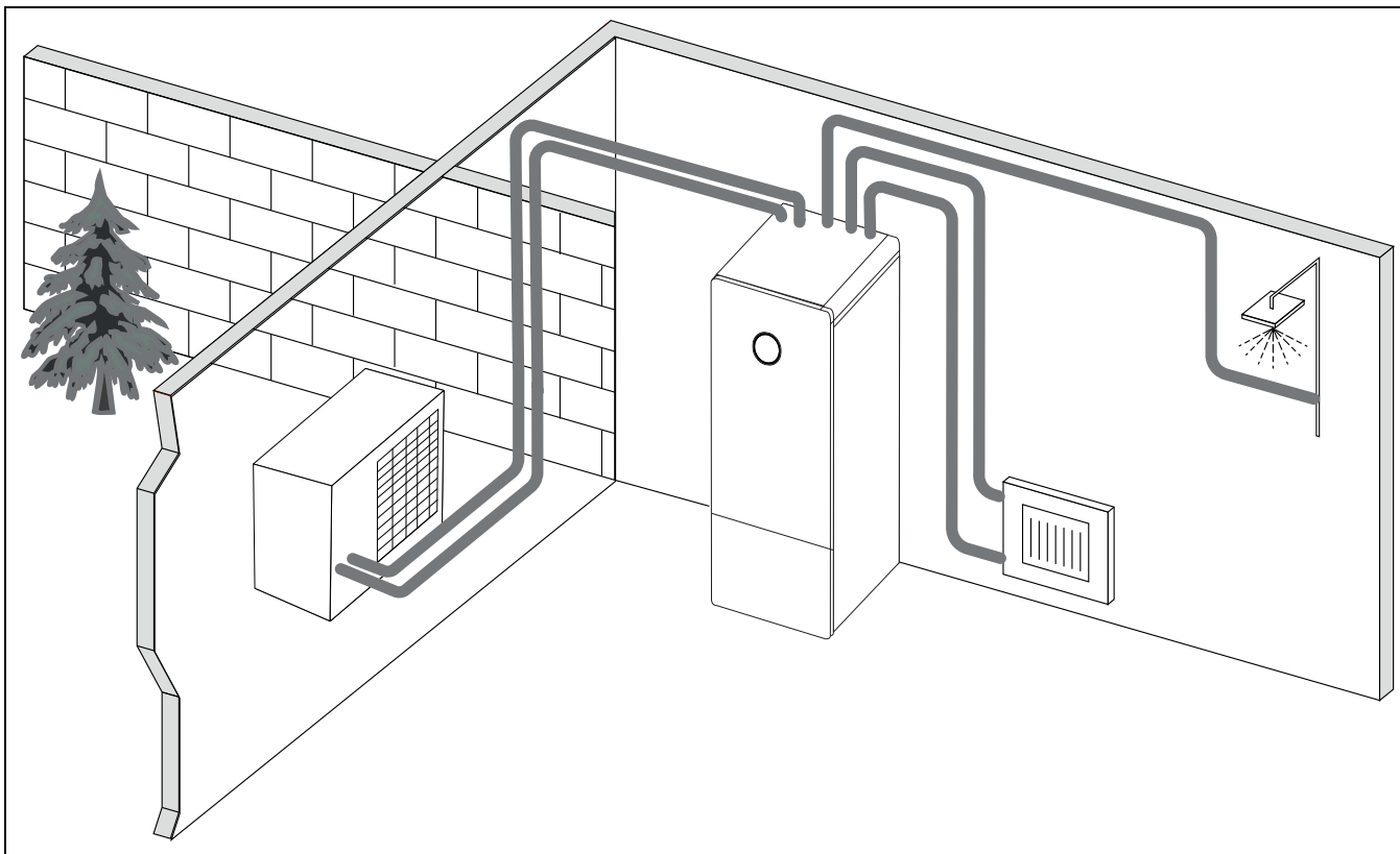
Rys. 7 Pompa ciepła AW OR, jednostka wewnętrzna Compress 5800i 12 M ze zintegrowanym podgrzewaczem pojemnościowym c.w.u. oraz grzałką zanurzeniową
