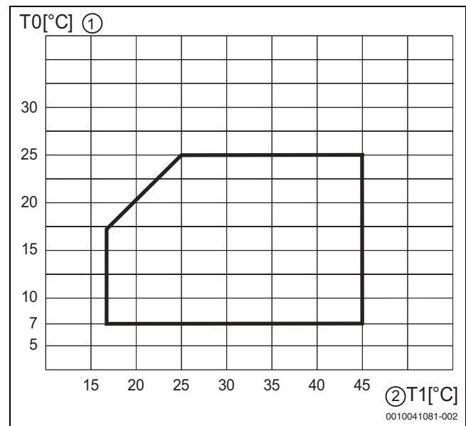
Rys. 5 Pompa ciepła w trybie chłodzenia
