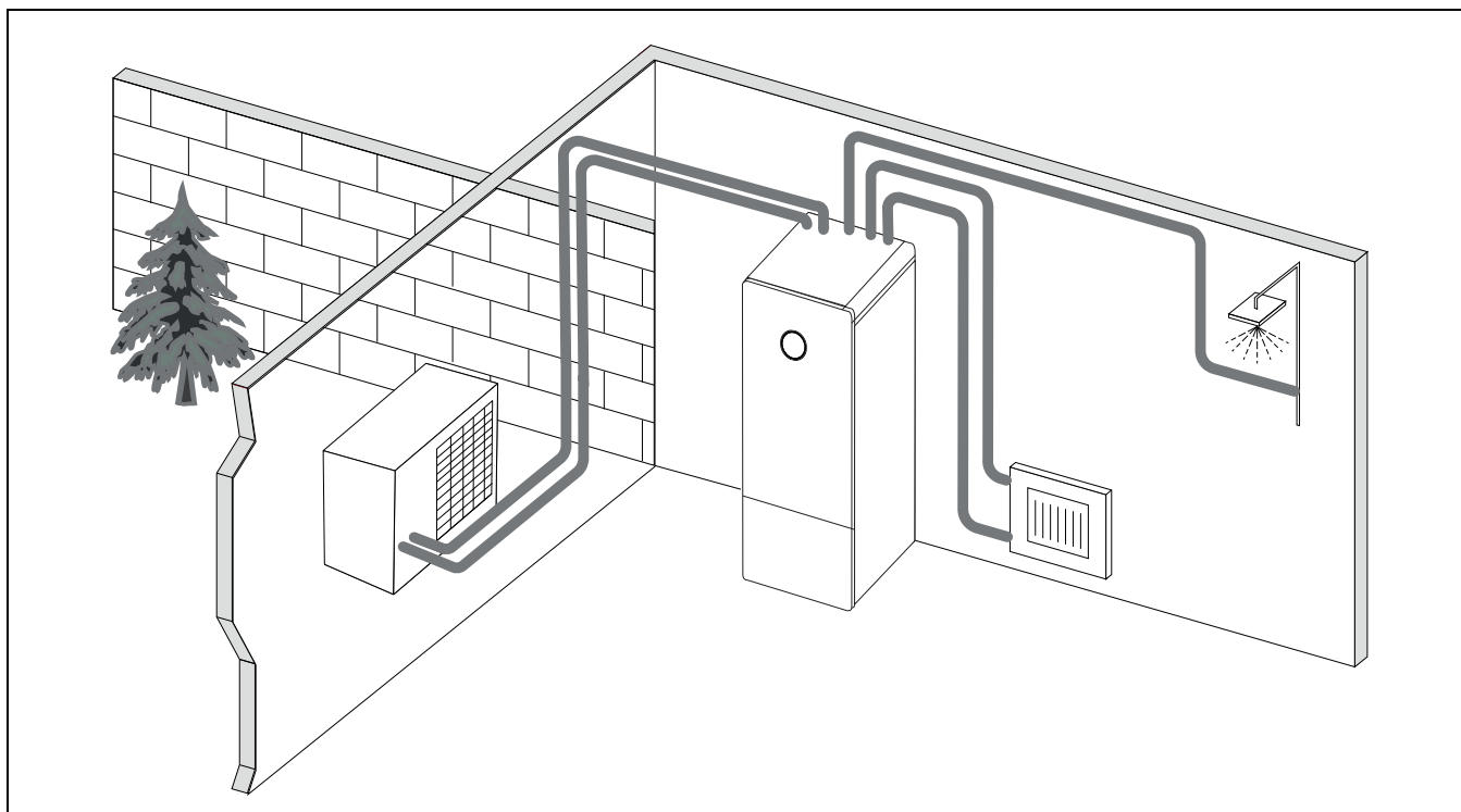
Rys. 5 Pompa ciepła AW OR, jednostka wewnętrzna Compress 5800/6800i 12 M ze zintegrowanym podgrzewaczem pojemnościowym c.w.u. oraz grzałką zanurzeniową
