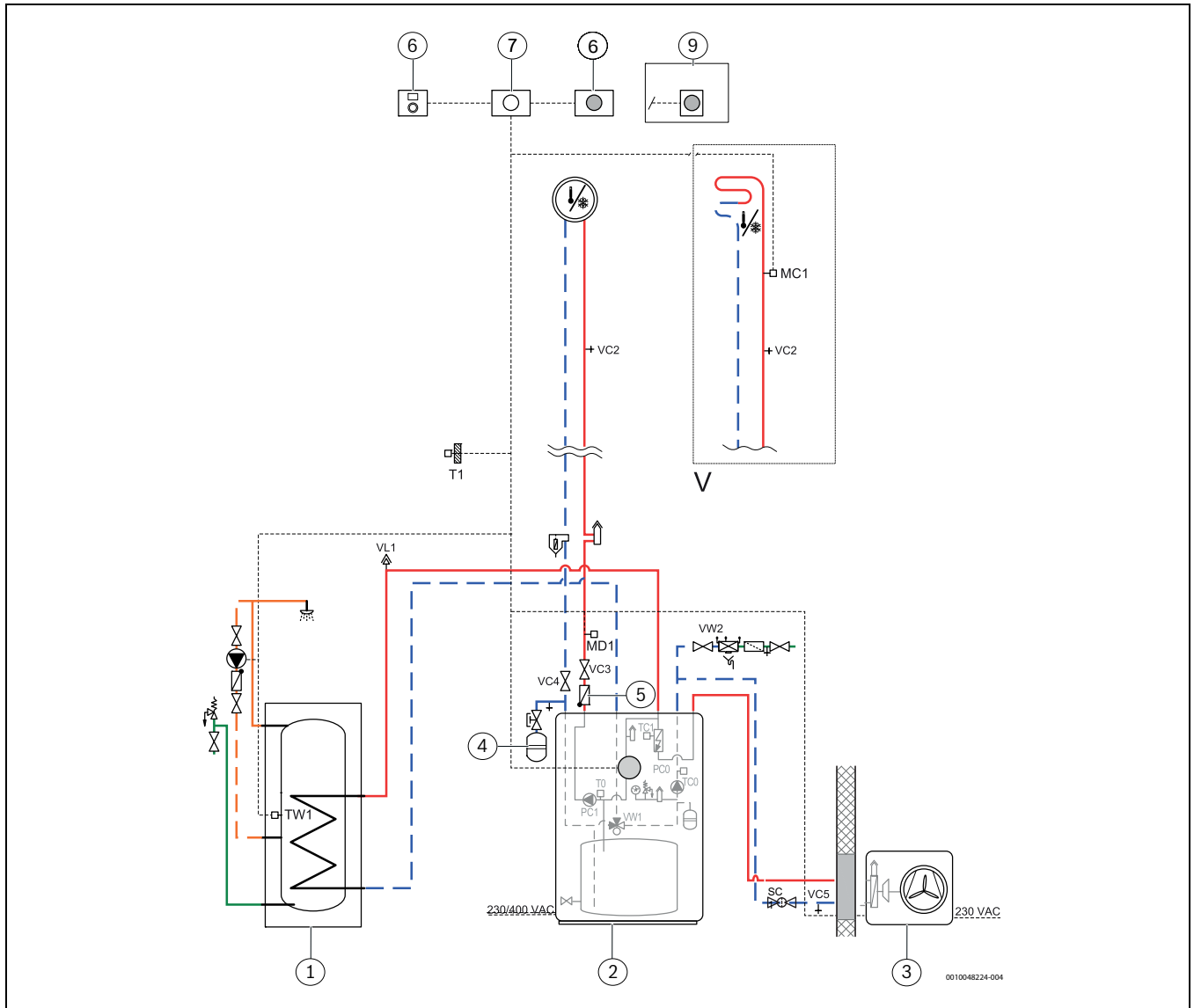
Rys. 24 Wariant instalacji z jednostką zewnętrzną, jednostką wewnętrzną ze zintegrowanym dogrzewaczem, zasobnikiem buforowym i obiegiem grzewczym bez zmieszania
