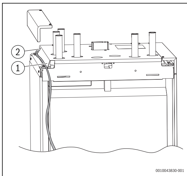
Rys. 29 Przepust kablowy w urządzeniu
