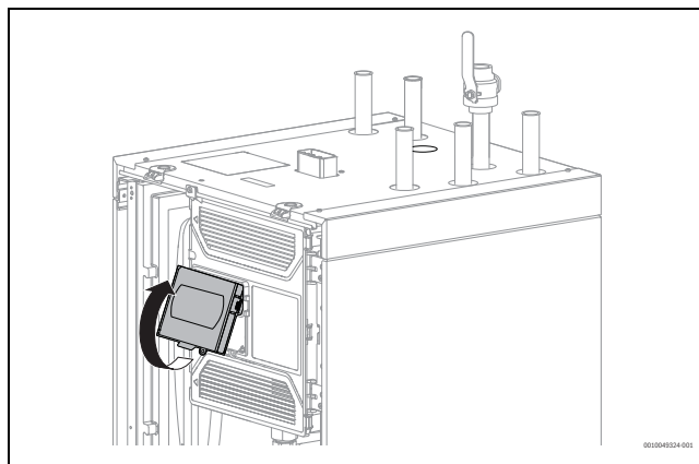
Rys. 47 Widok z przodu: skrzynka elektroniczna ze śrubą zabezpieczającą
