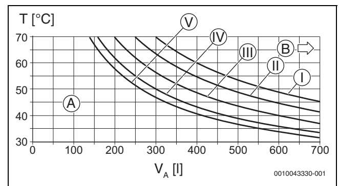
Rys. 7 Krzywe dla naczynia wzbiórczego (17 l)
