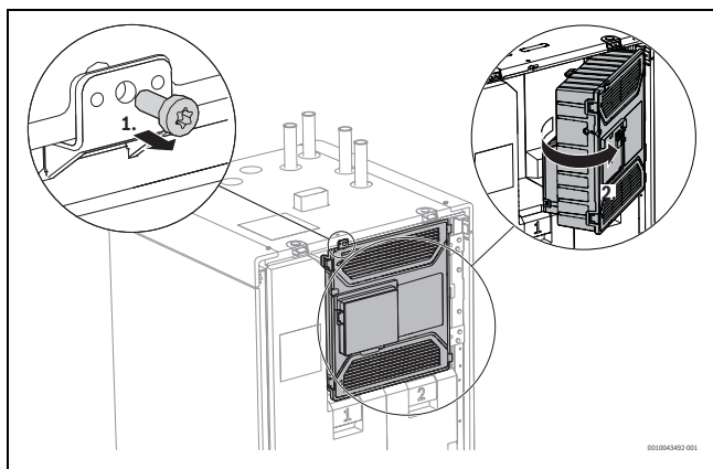
Rys. 49 Skrzynka elektroniczna
