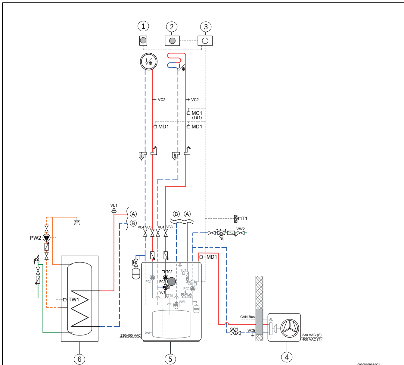
Rys. 57 Rozwiązanie systemowe z dodatkowym wewnętrznym zestawem rozszerzającym 2HK
