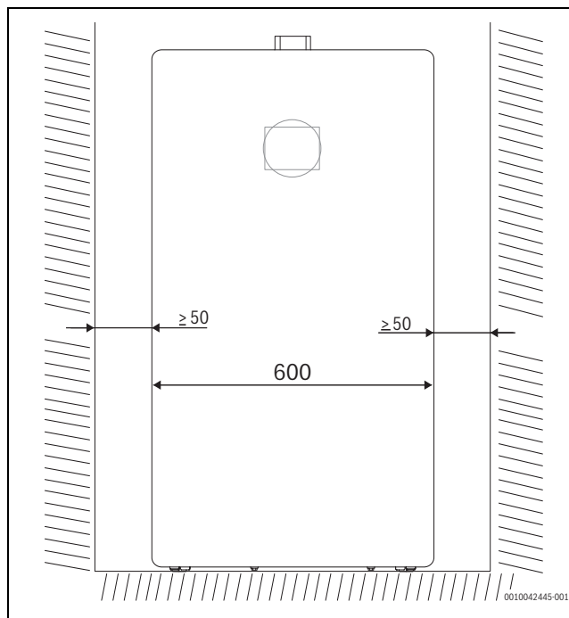
Rys. 2 Widok z przodu: minimalna odległość od krawędzi bocznej do ściany. Odległość od innych jednostek wynosi 0 mm.
