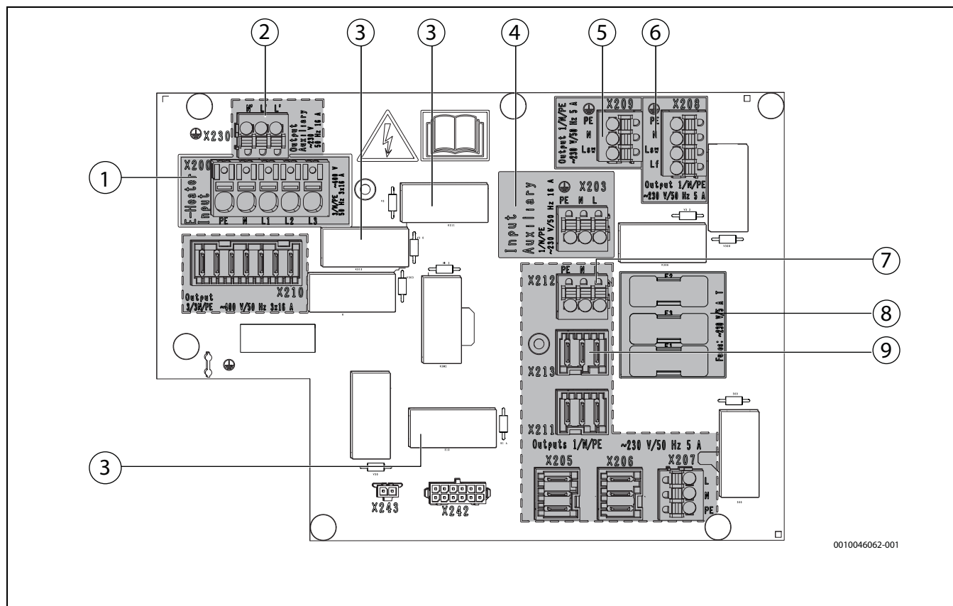
Rys. 39 Przyłącza na płycie głównej
