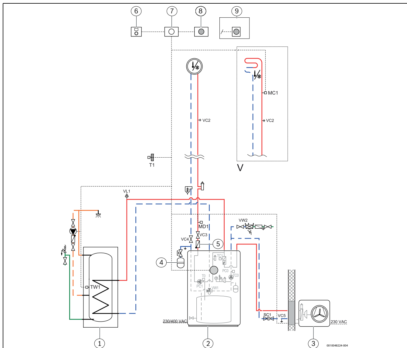
Rys. 58 System z jednostką zewnętrzną, jednostką wewnętrzną ze zintegrowanym dogrzewaczem i zasobnikiem buforowym oraz jednym obiegiem grzewczym bez zaworu mieszającego
