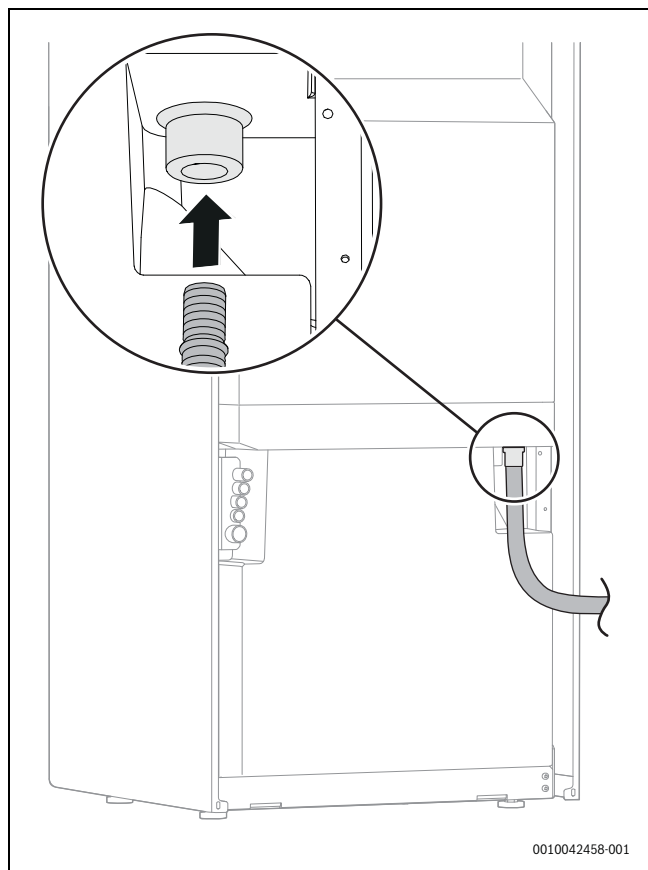
Rys. 23 Podłączanie węża odpływowego do urządzenia
