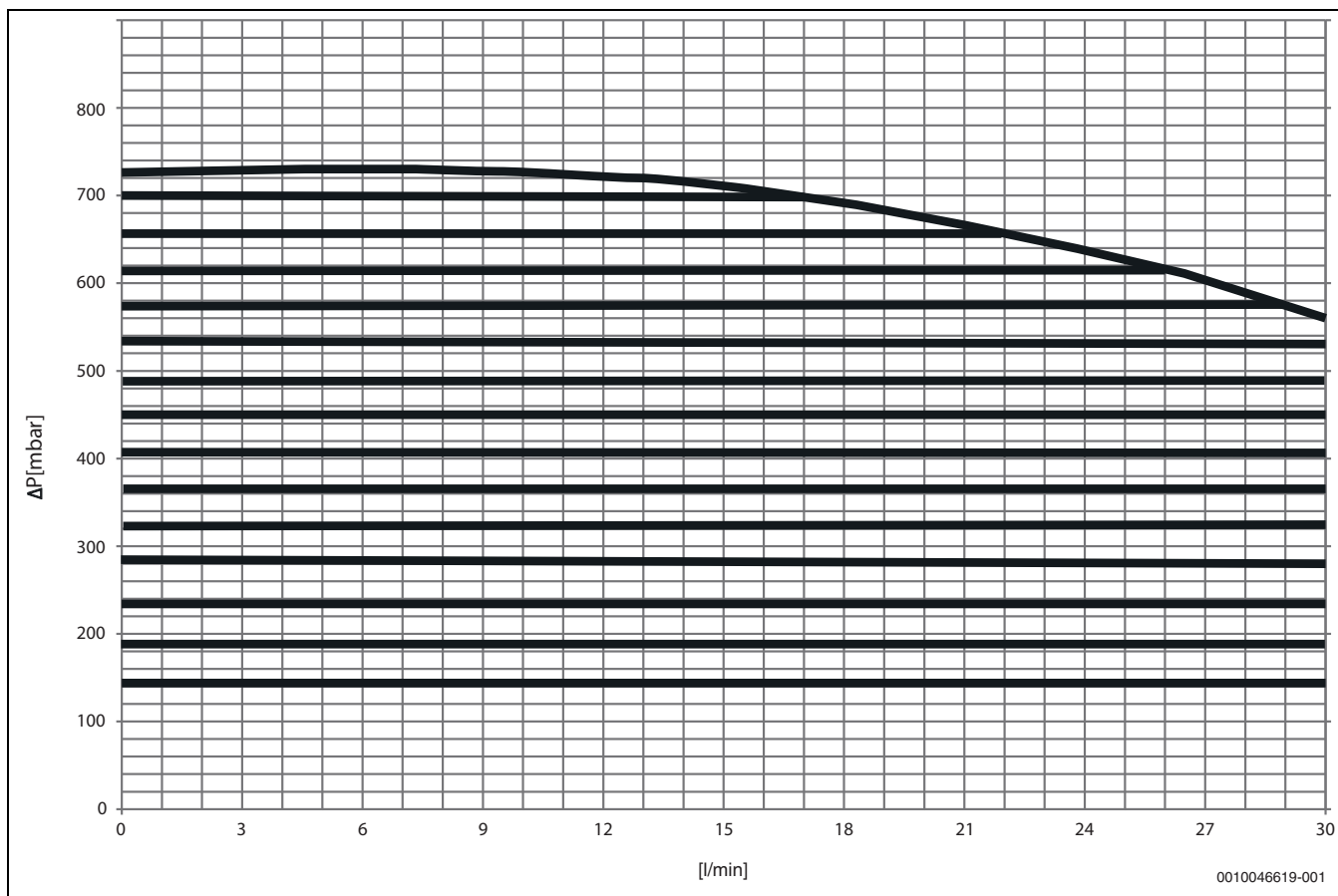
Rys. 53 Wykres mocy dla pompy PC1 w obiegu grzewczym ze zmieszaniem ze stałym ciśnieniem
