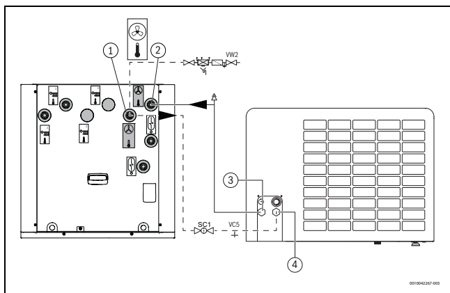
Rys. 19 Podłączenie jednostki zewnętrznej
