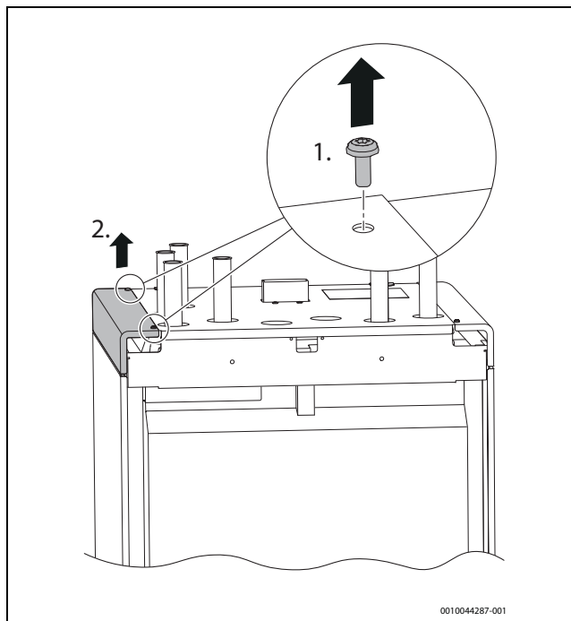
Rys. 28 Widok z tyłu: narożniki ze śrubami mocującymi
