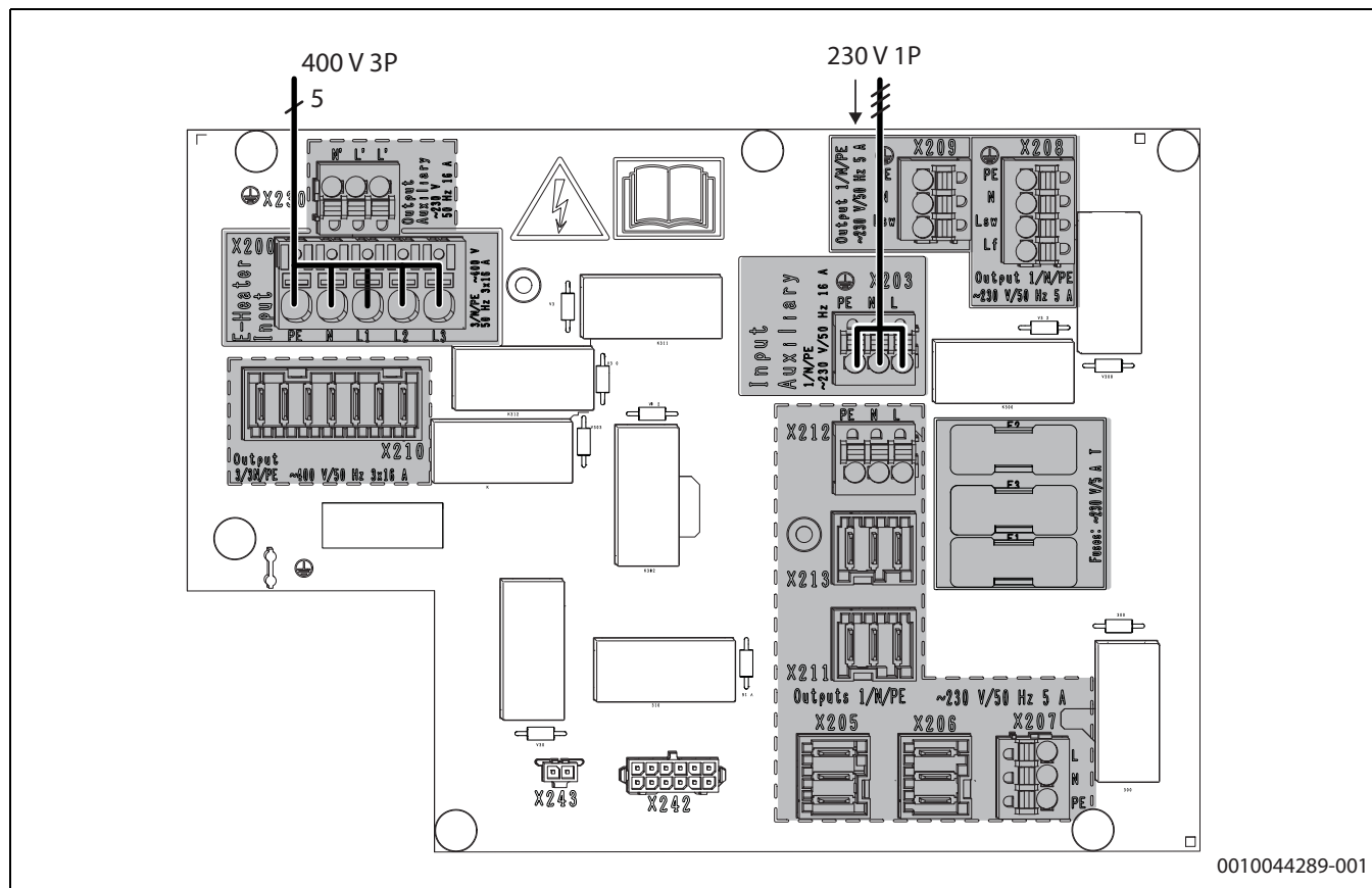
Rys. 37 Przyłącze 400 V ogrzewacza elektrycznego, przyłącze 230 V sterownika i pomp
