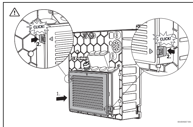
Rys. 50 Prawidłowe położenie pokrywy
