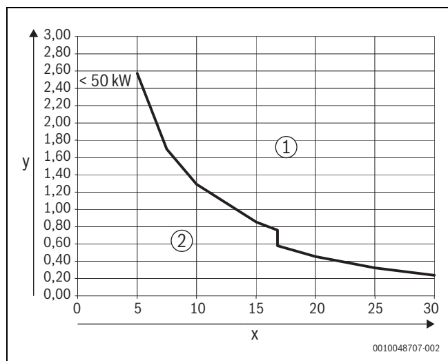
Rys. 6 Urządzenia grzewcze < 50–100 kW
