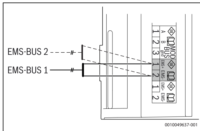
Rys. 43 Podłączanie kilku przewodów EMS-BUS w obszarze przyłączy XCU-THH dla przewodów sterowania i czujników
