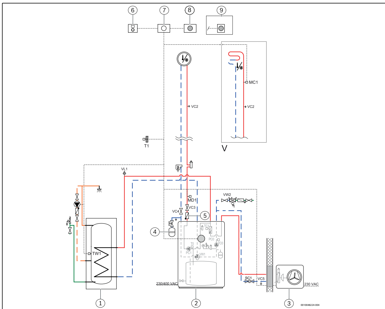
Rys. 58 System z jednostką zewnętrzną, jednostką wewnętrzną ze zintegrowanym dogrzewaczem i zasobnikiem buforowym oraz jednym obiegiem grzewczym bez zaworu mieszającego
