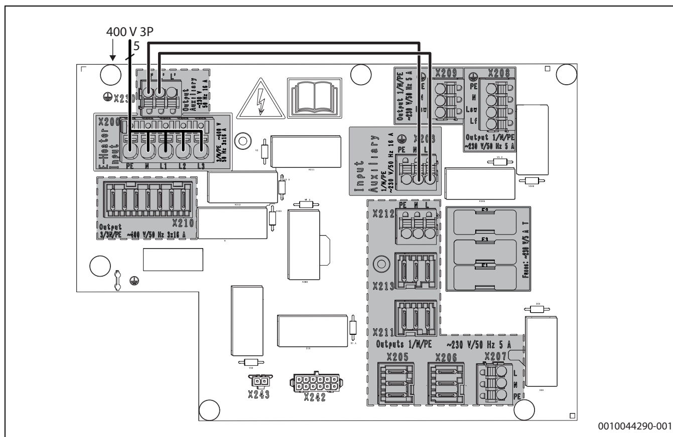
Rys. 38 Przyłącze 400 V dogrzewacza elektrycznego ze zmostkowanym przyłączem 230 V sterownika i pomp
