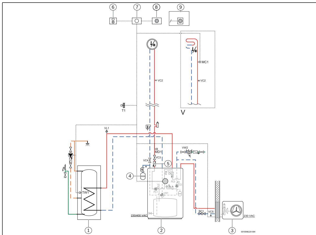
Rys. 59 Systemy z jednostką zewnętrzną, jednostką wewnętrzną ze zintegrowanym dogrzewaczem i zasobnikiem buforowym oraz jednym obiegiem grzewczym bez zaworu mieszającego i jednym obiegiem grzewczym z zaworem mieszającym
