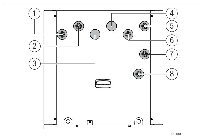
Rys. 18 Obszar przyłączy hydraulicznych
