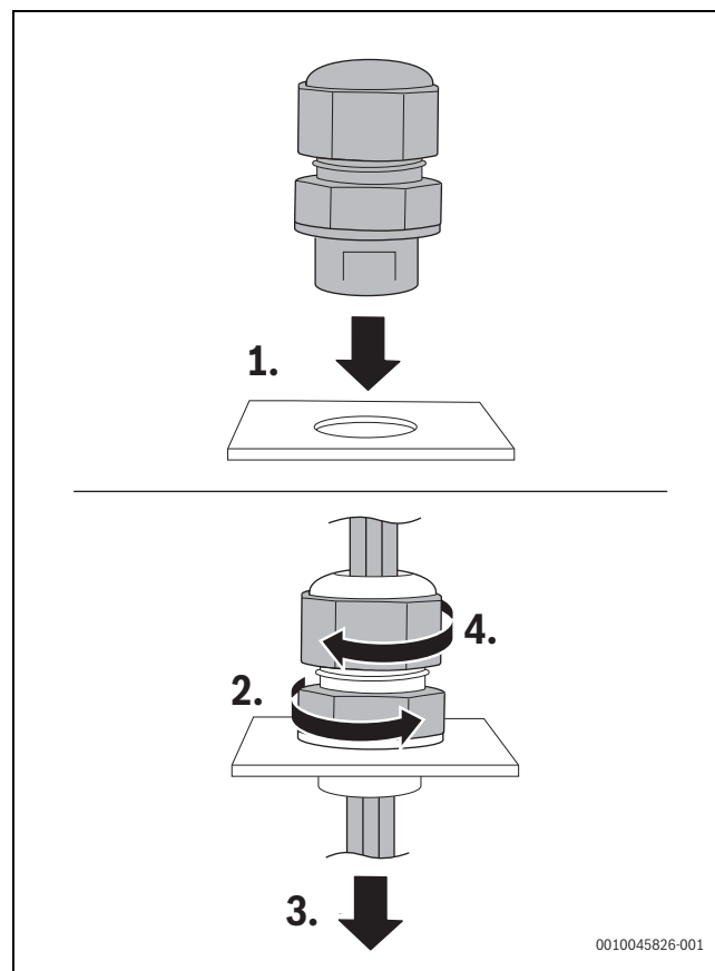
Rys. 31 Wkładanie dławików kablowych
