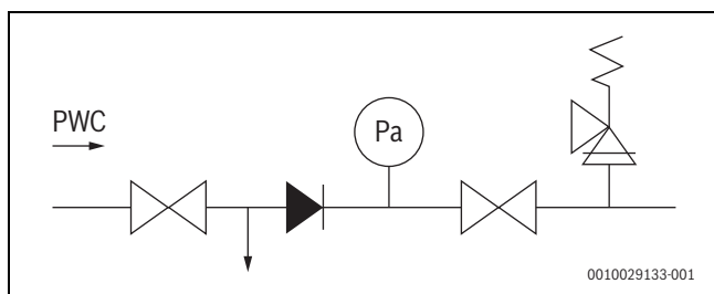
Rys. 20 Przykład: grupa bezpieczeństwa w wodzie w zespole rozprężnym wg EN 1488
