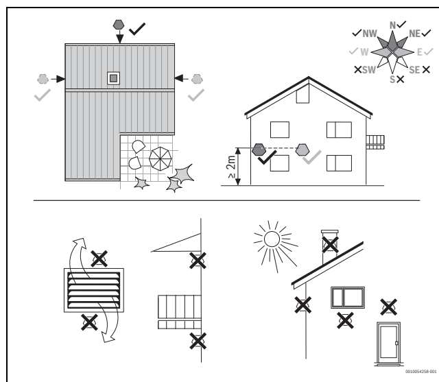
Rys. 44 Położenie czujnika temperatury zewnętrznej
