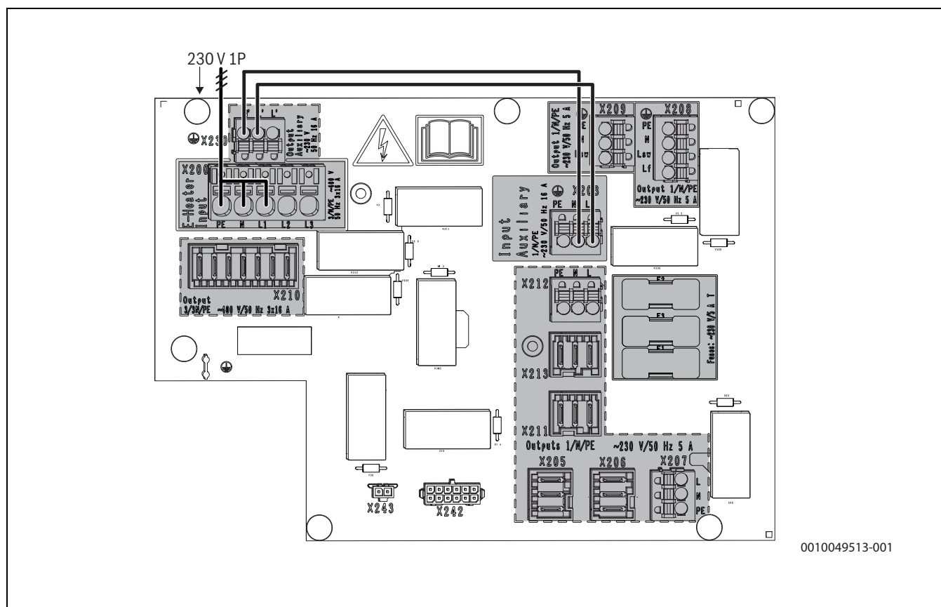
Rys. 36 Przyłącze 230 V ogrzewacza elektrycznego ze zmostkowanym przyłączem 230 V sterownika i pomp
