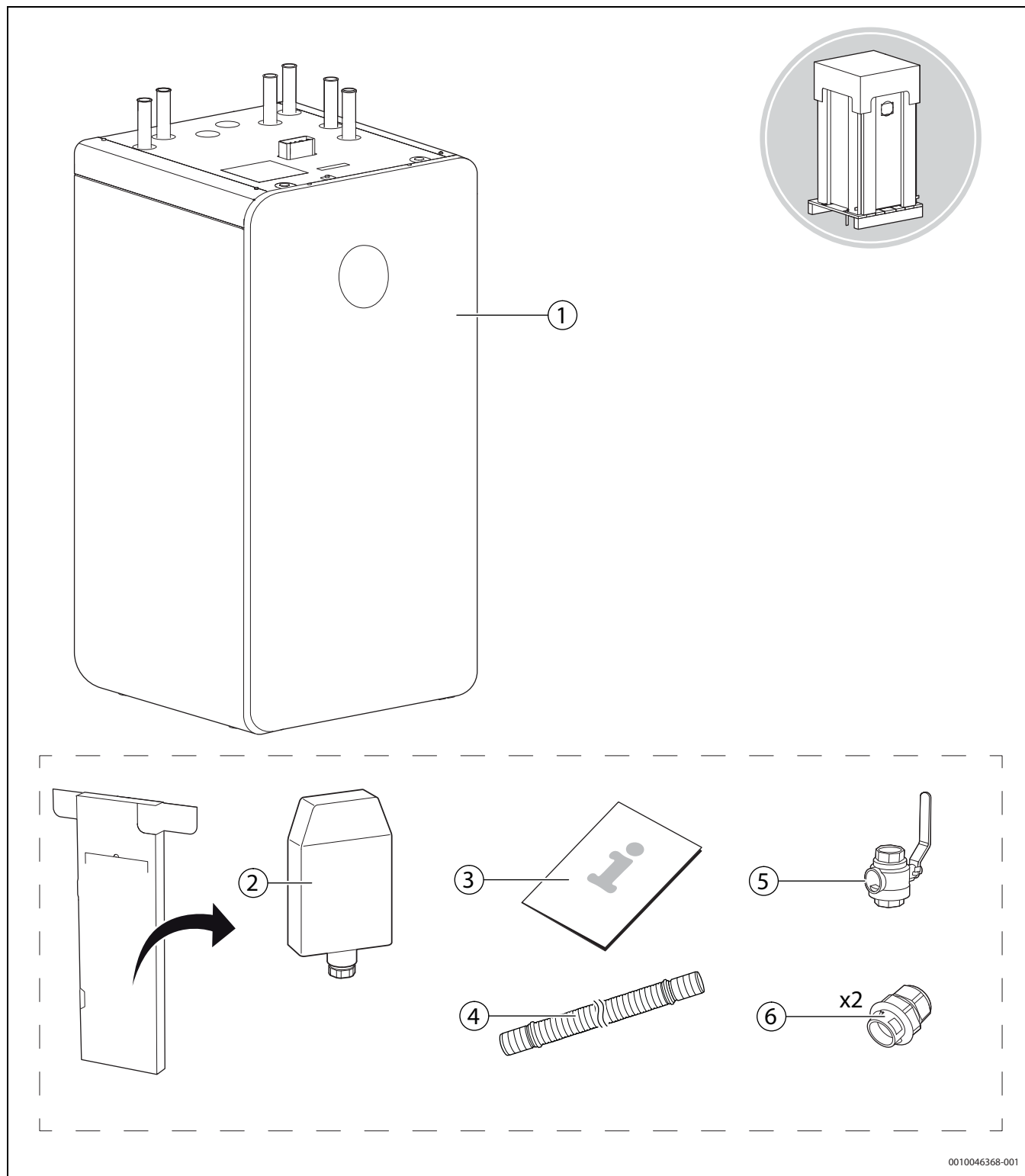
Rys. 1 Zakres dostawy
