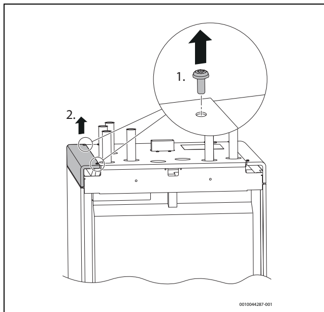
Rys. 28 Widok z tyłu: narożniki ze śrubami mocującymi
