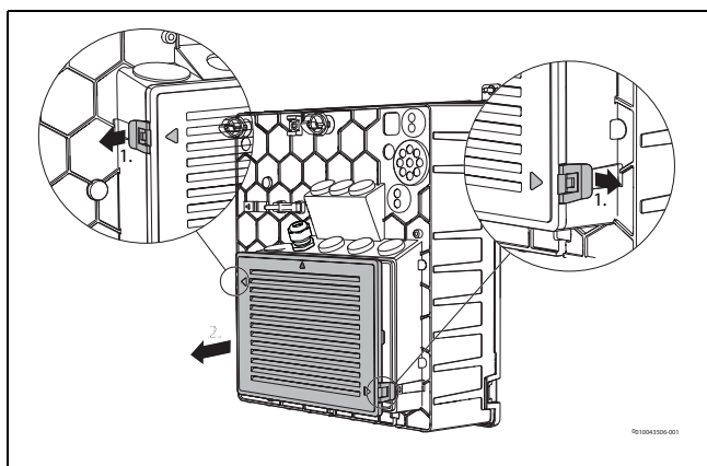
Rys. 33 Zdejmowanie pokrywy
