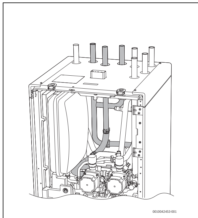
Rys. 13 Osprzęt dodatkowy zamontowany w urządzeniu
