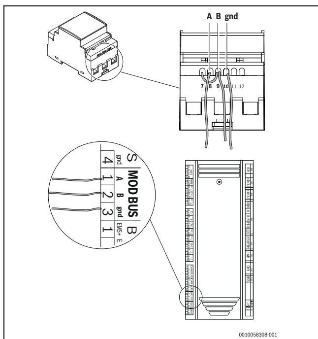
Rys. 14 Połączenie licznika Power Meter 5000 z jednostką wewnętrzną
