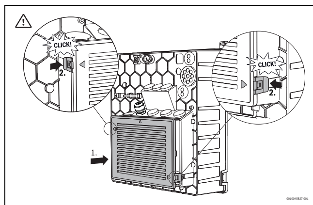
Rys. 40 Prawidłowe położenie pokrywy
