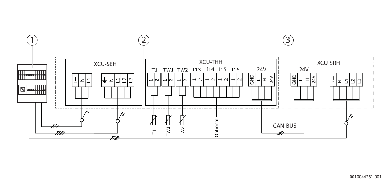
Rys. 55 Uproszczony schemat elektryczny 3 N~
