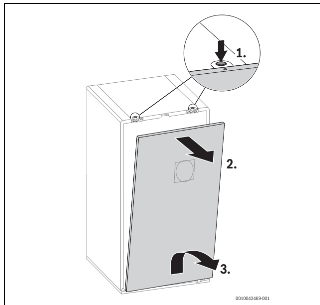
Rys. 12 Zdjąć przednią część obudowy
