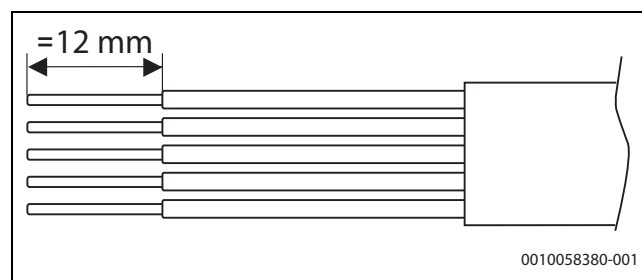
Rys. 32 Usuwanie izolacji z przewodu zasilania sieciowego
