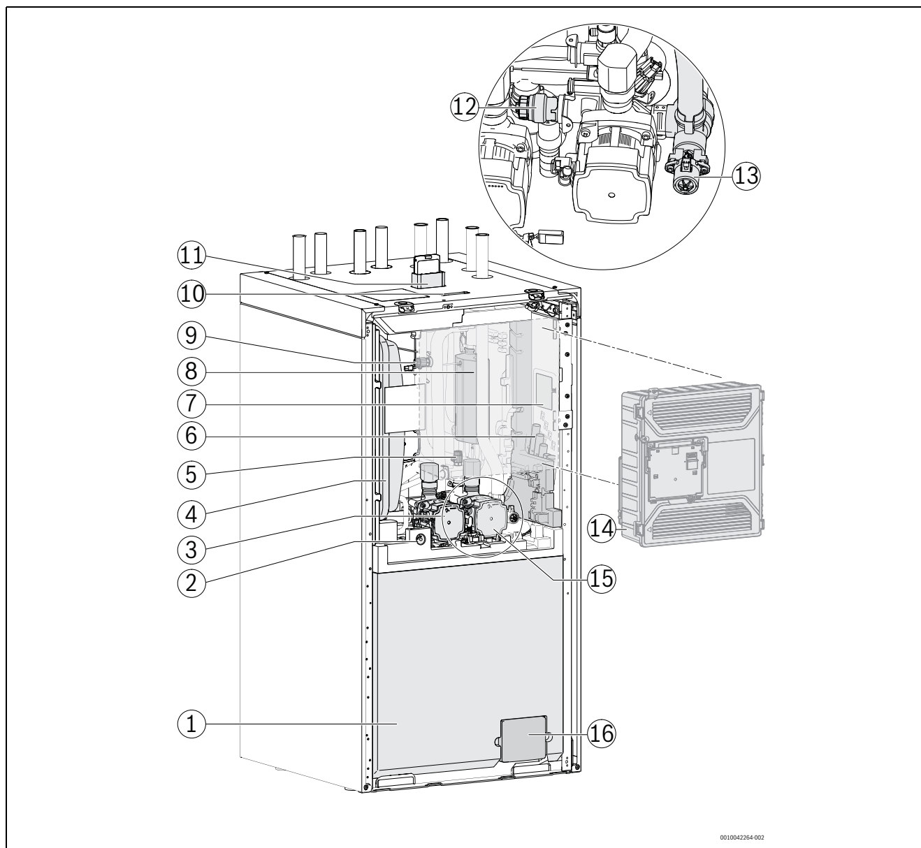
Rys. 5 Jednostka wewnętrzna dodatkowym zestawem rozszerzającym 2HK zewnętrznym i Connect-Key
