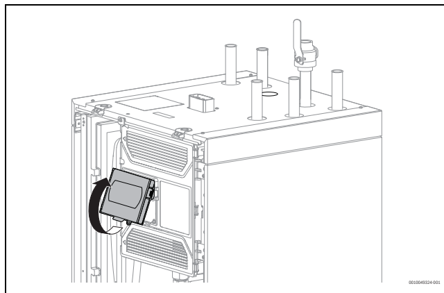
Rys. 47 Widok z przodu: skrzynka elektroniki ze śrubą zabezpieczającą
