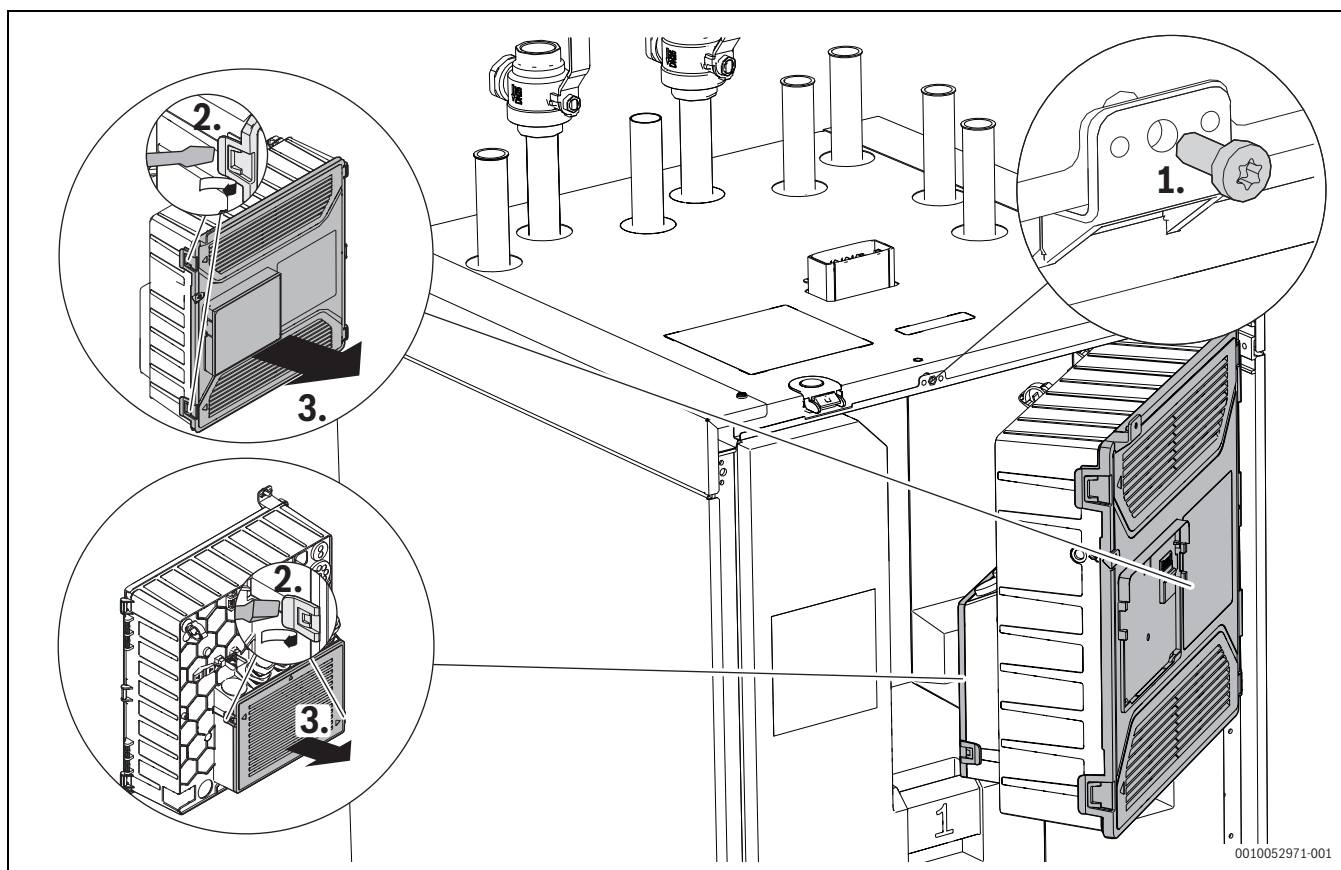
Rys. 26 Widok z przodu: skrzynka elektroniki ze śrubą zabezpieczającą
