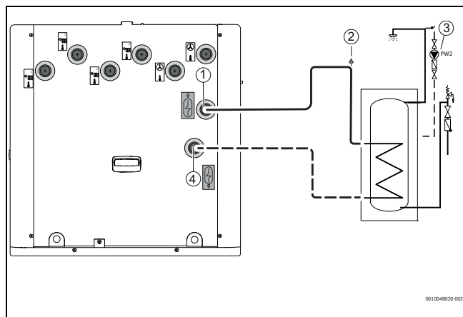
Rys. 22 Podłączanie podgrzewacza pojemnościowego c.w.u.
