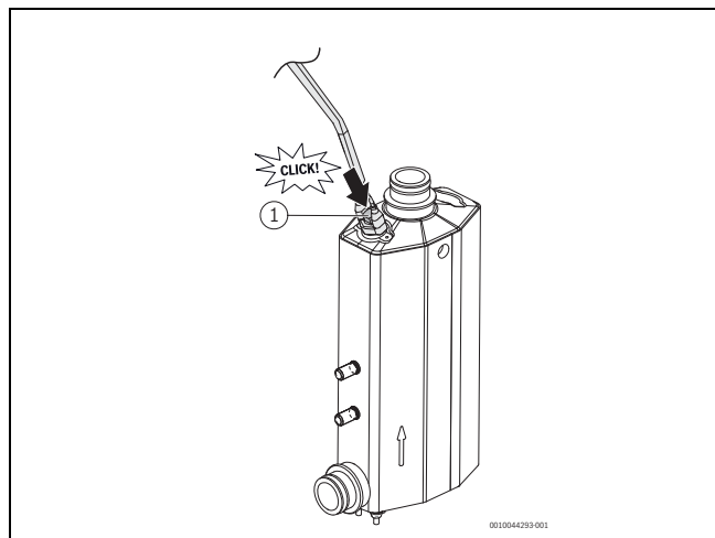
Rys. 48 Dogrzewacz elektryczny (stopnie mocy)
