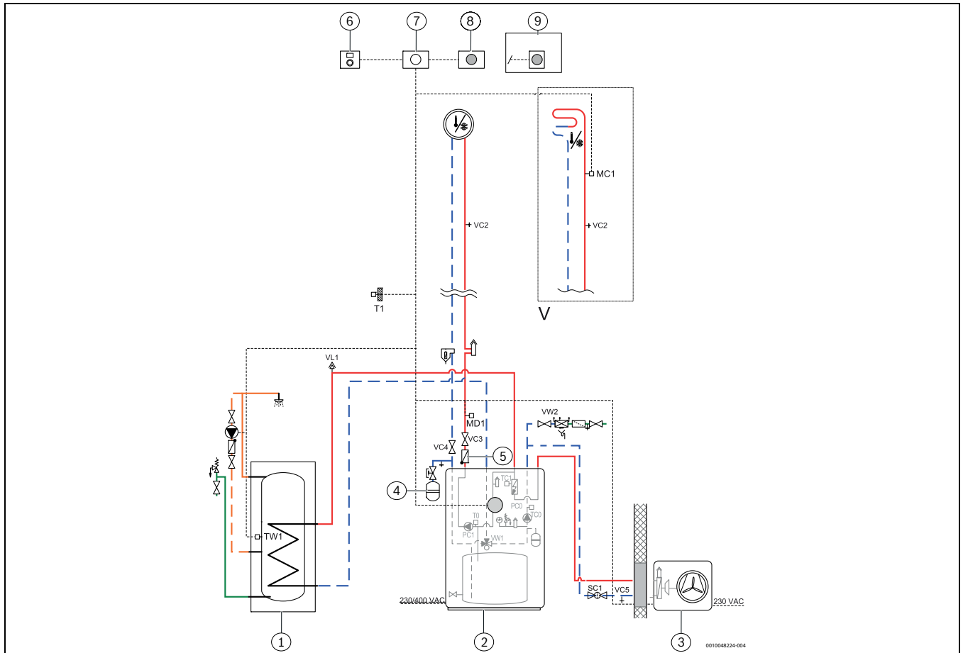
Rys. 24 Rozwiązanie systemowe z jednostką zewnętrzną, jednostką wewnętrzną ze zintegrowanym dogrzewaczem i zasobnikiem buforowym oraz jednym obiegiem grzewczym bez zaworu mieszającego
