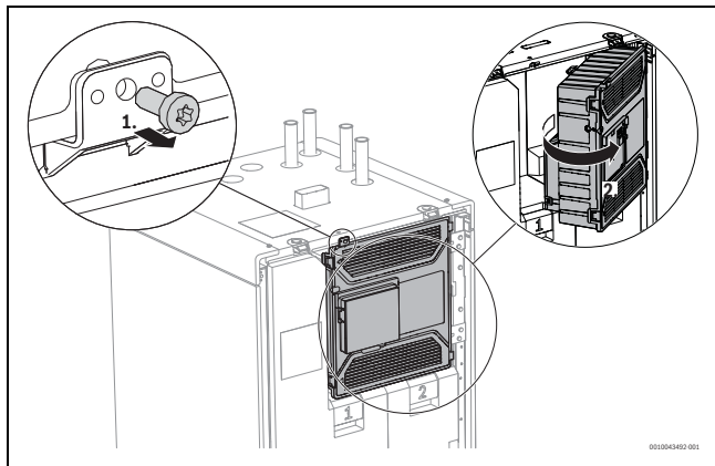
Rys. 49 Skrzynka elektroniki
