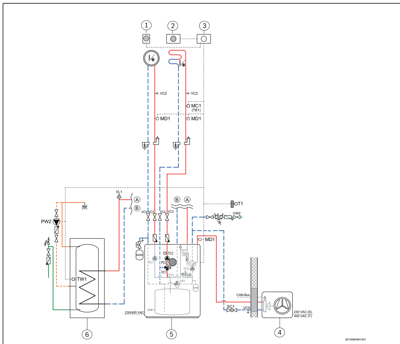
Rys. 57 Rozwiązanie systemowe z dodatkowym wewnętrznym zestawem rozszerzającym 2HK
