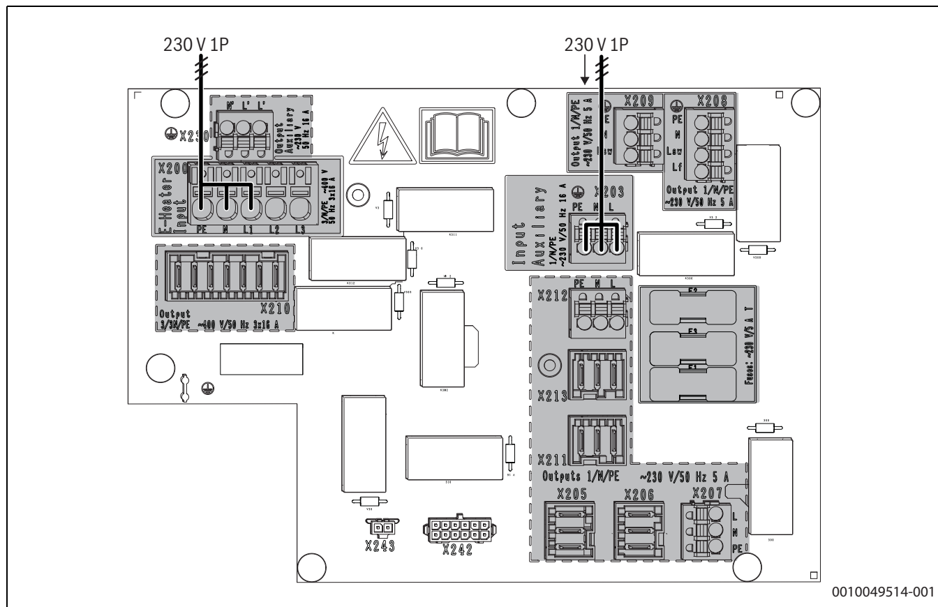
Rys. 35 Przyłącze 230 V ogrzewacza elektrycznego, przyłącze 230 V sterownika i pomp
