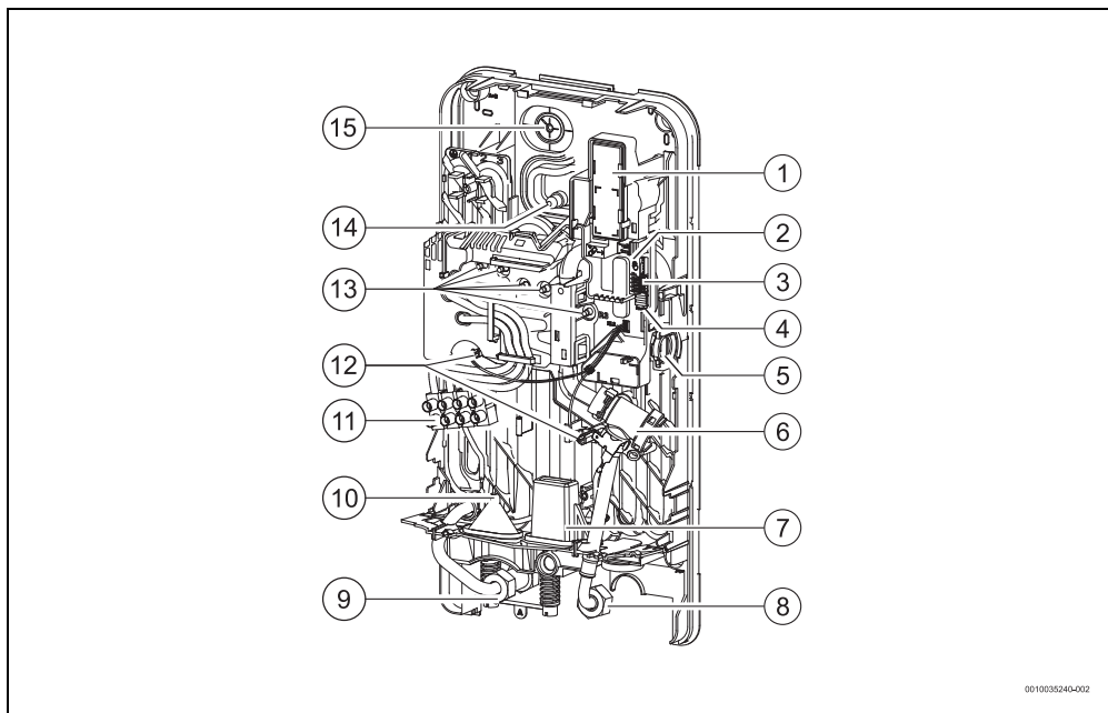
Rys. 5 Komponenty urządzenia
