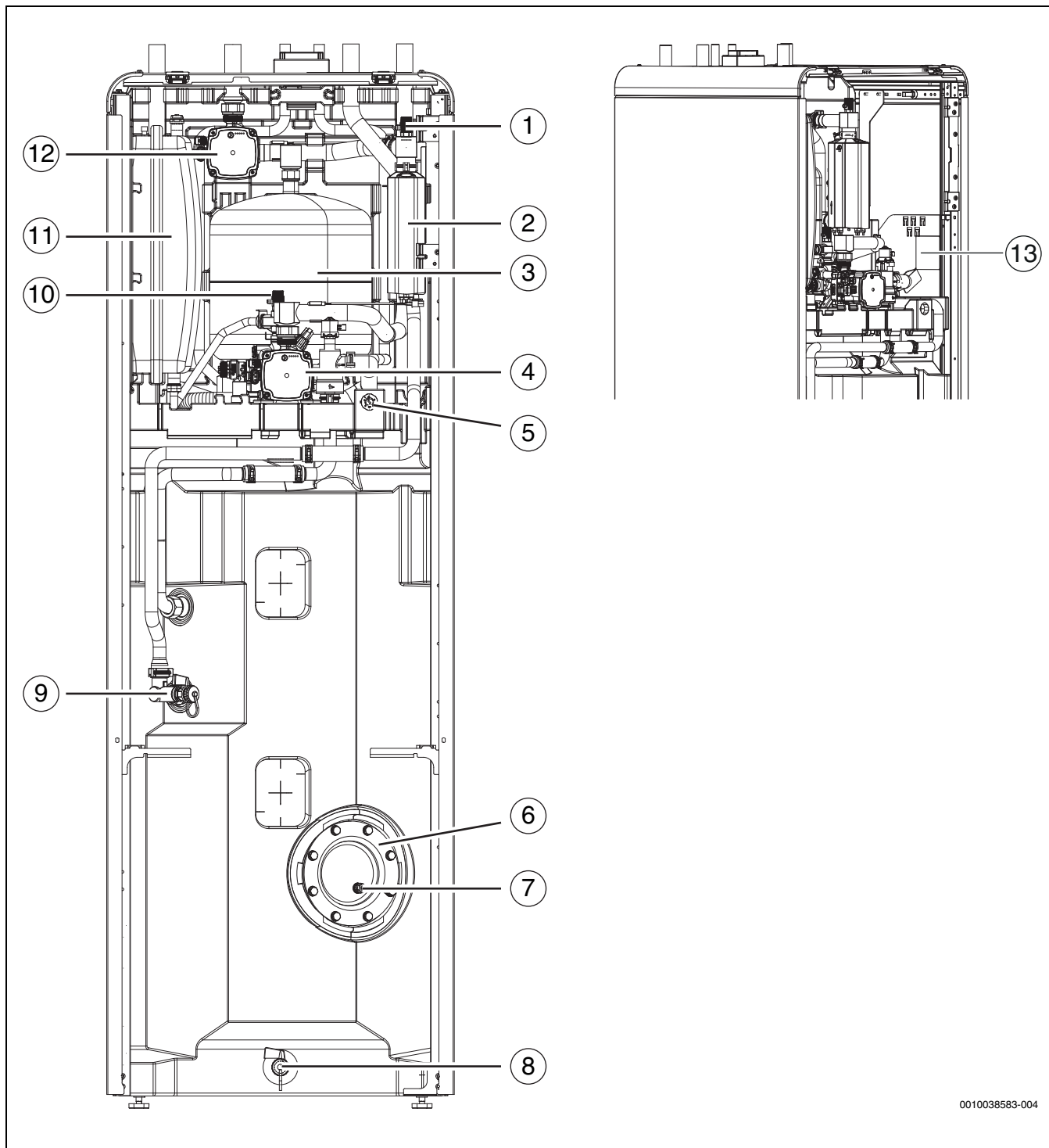
Rys. 5 Widok ogólny urządzenia, widok z przodu i z góry
