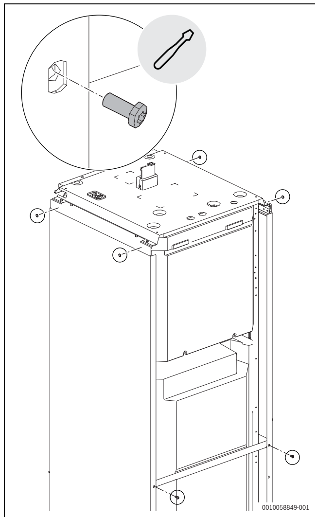
Rys. 16 Śruby ścianek bocznych
