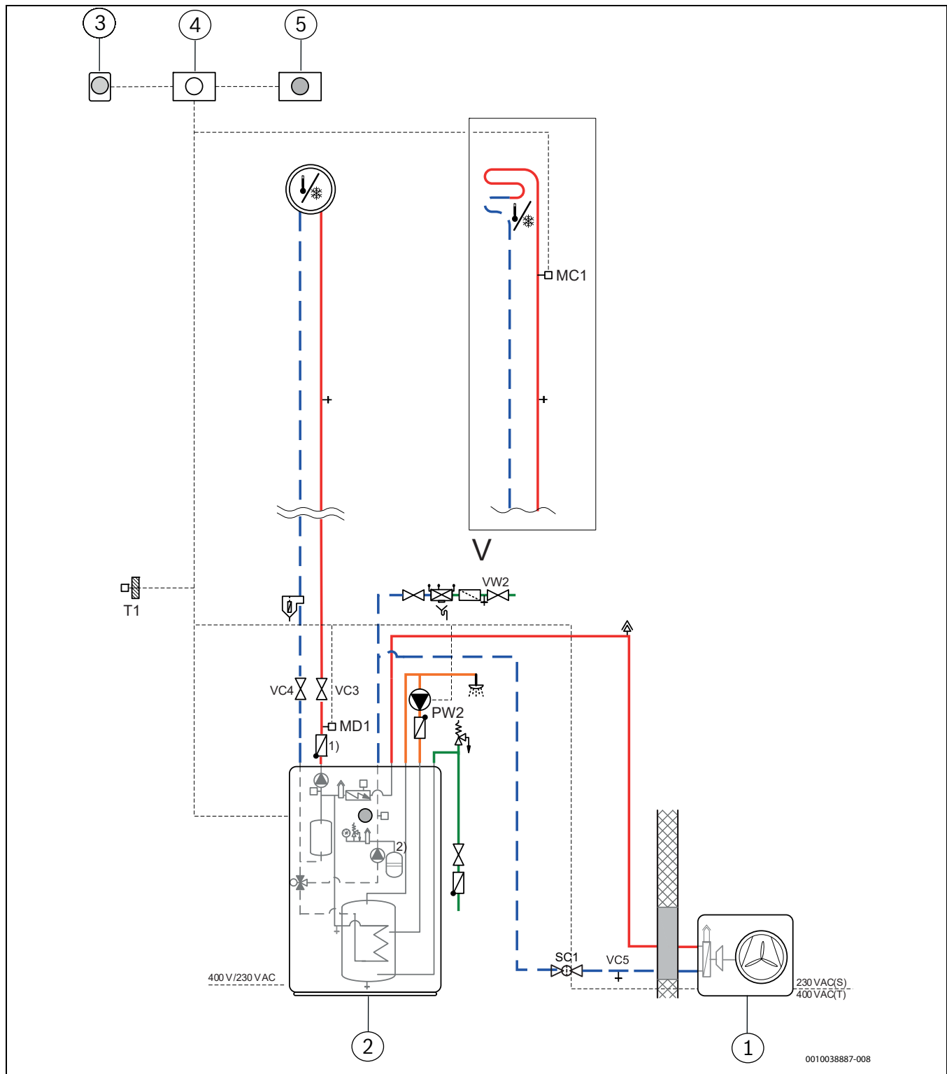
Rys. 49 Jednostka wewnętrzna Tower, pompa ciepła (ODU), jeden obieg grzewczy bez mieszania
