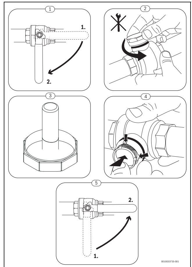
Rys. 46 Czyszczenie filtra magnetycznego
