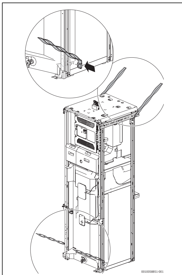
Rys. 18 Pasy transportowe
