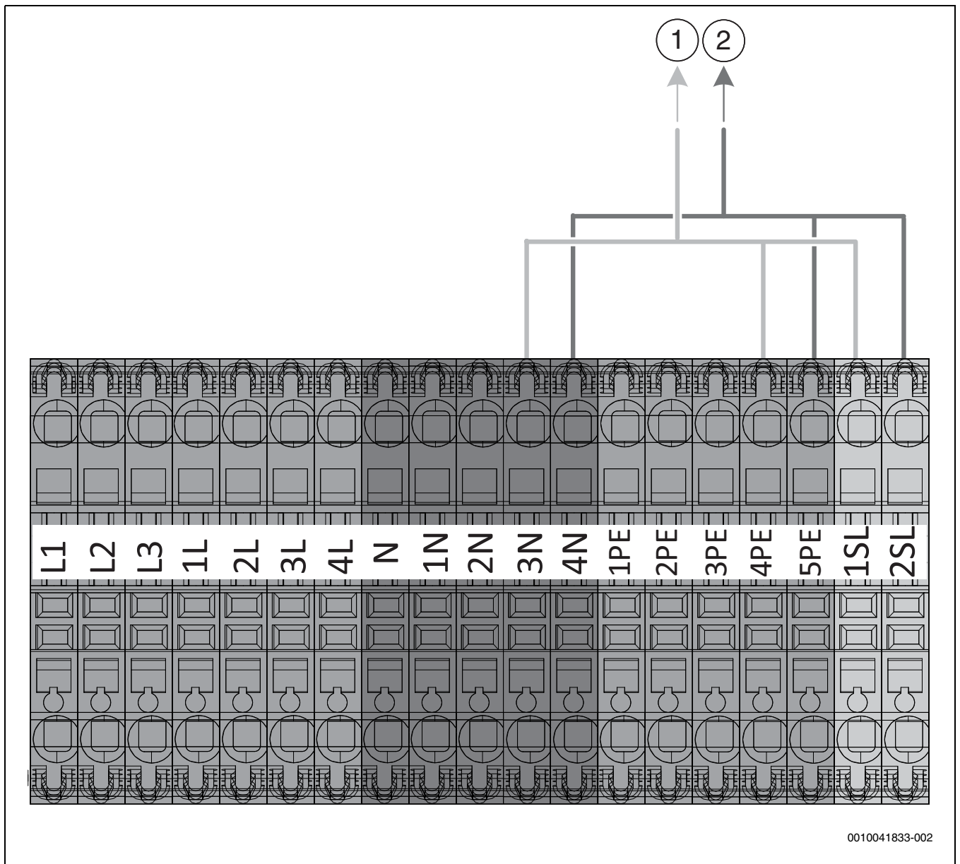
Rys. 42 Podłączenia elektryczne osprzętu dodatkowego
