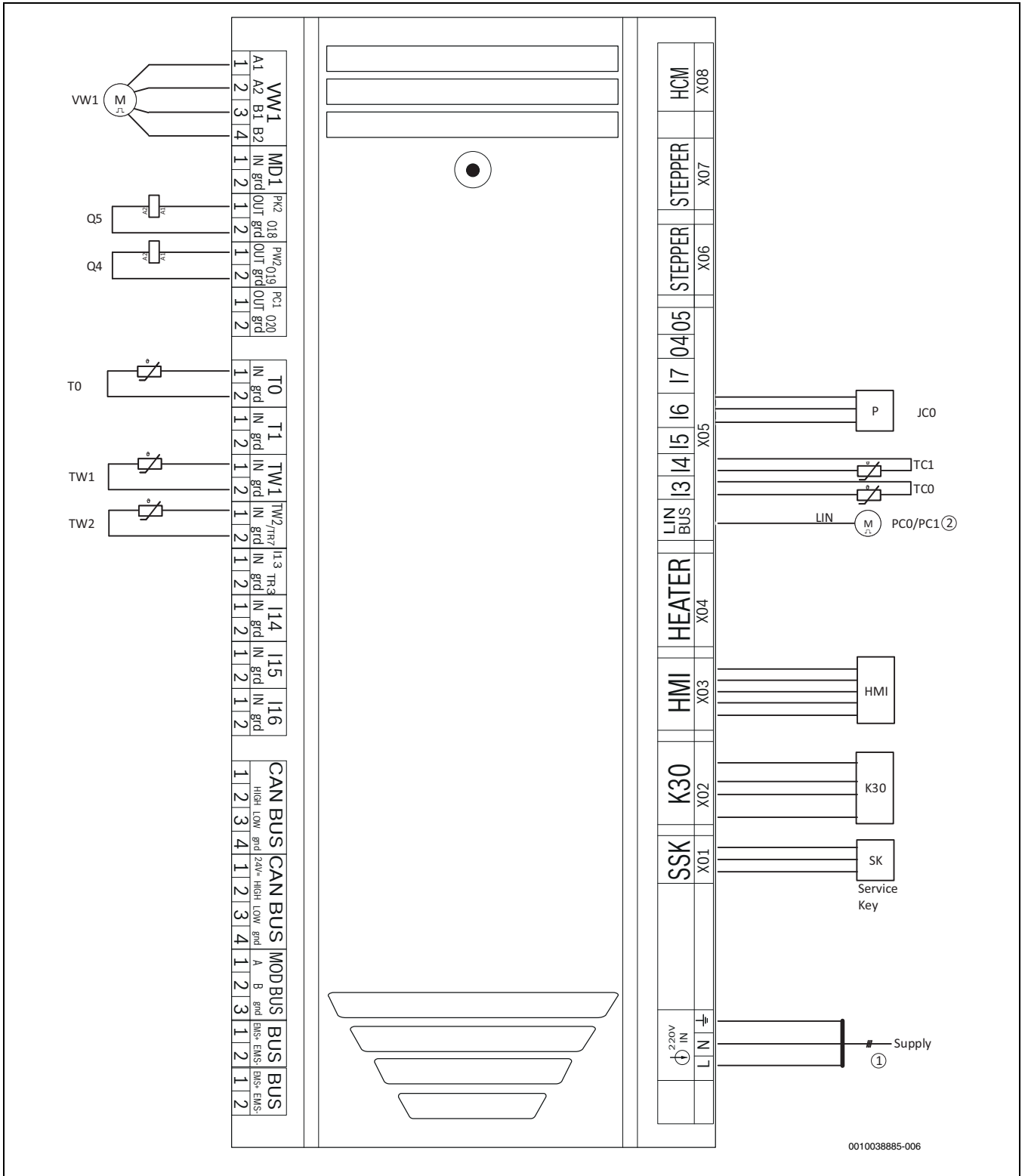
Rys. 51 Schemat elektryczny modułu XCU-THH (XCU HY)
