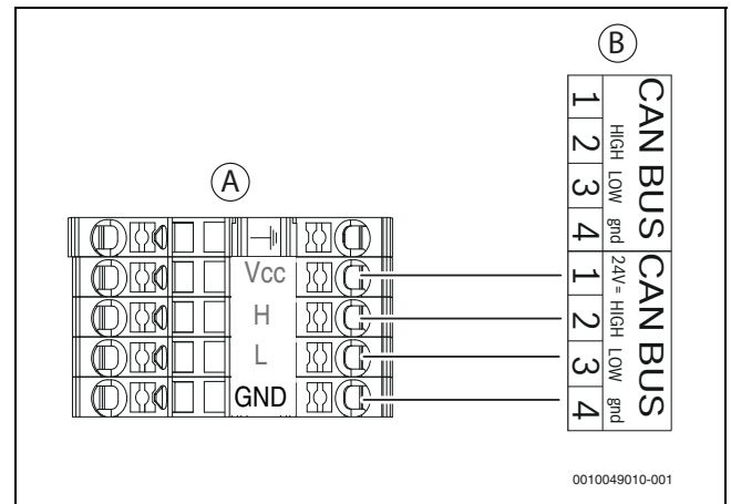
Rys. 32 Magistrala CAN-BUS pompy ciepła – jednostka wewnętrzna
