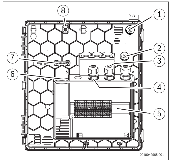
Rys. 38 Wejścia kablowe do skrzynki zaciskowej
