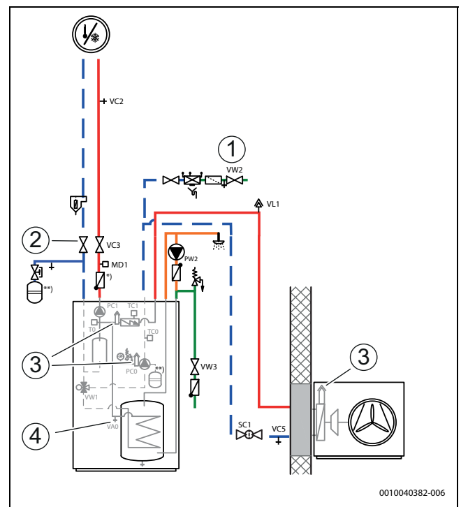
Rys. 30 Jednostka wewnętrzna, pompa ciepła i instalacja grzewcza
