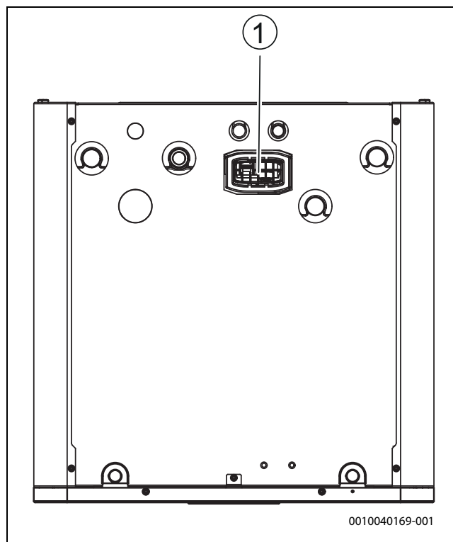
Rys. 21 Montaż Connect-Key
