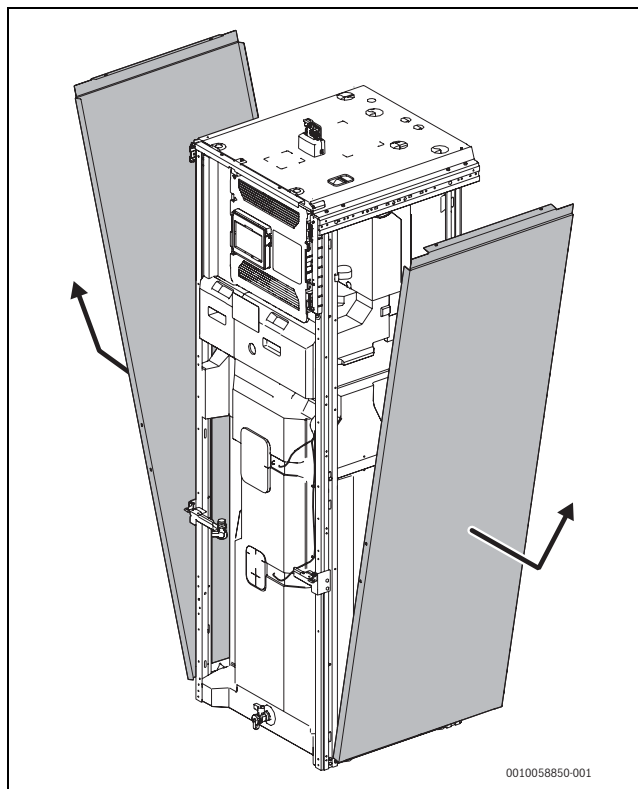
Rys. 17 Osłona boczna
