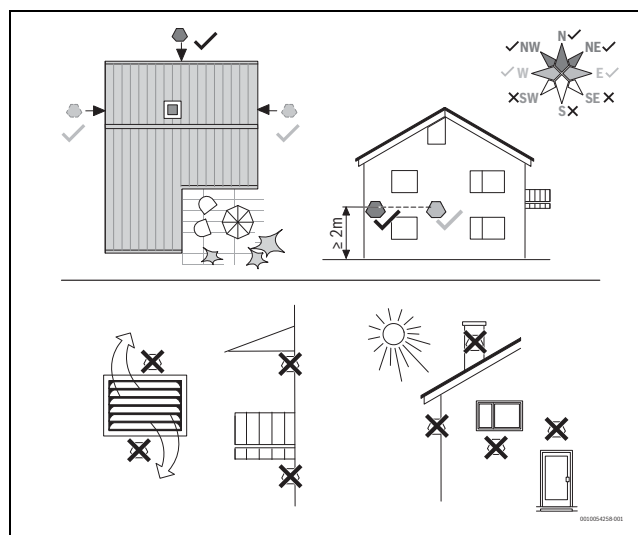
Rys. 35 Położenie czujnika temperatury zewnętrznej
