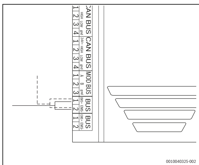
Rys. 34 Podłączenie EMS
