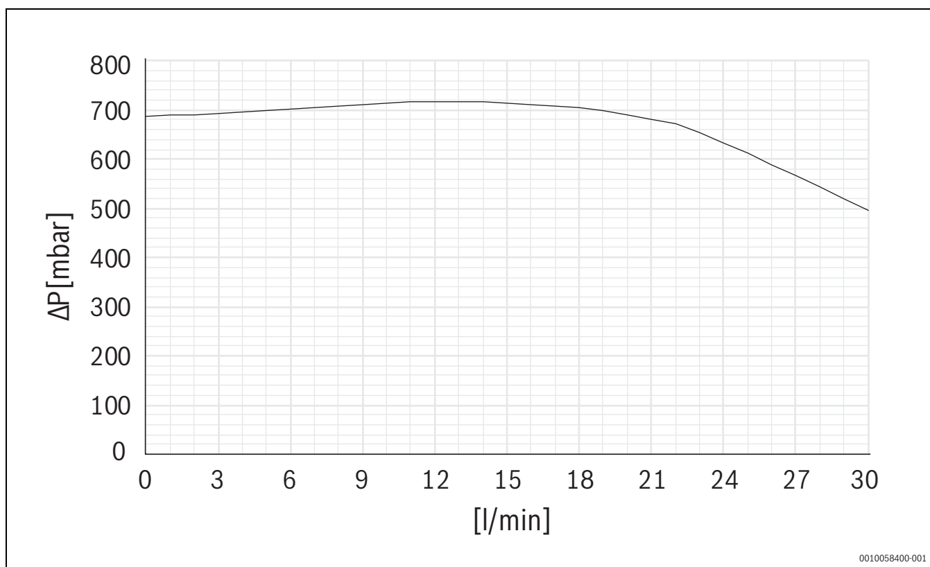
Rys. 41 Wykres wydajności PC2
