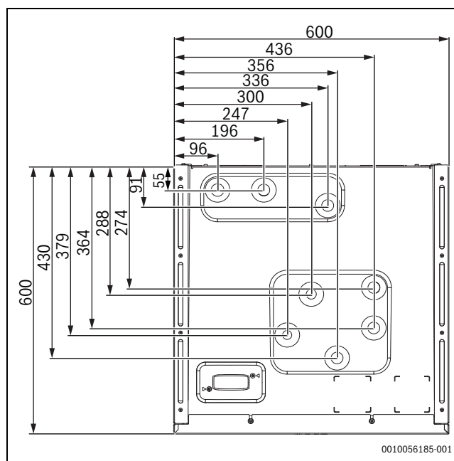
Rys. 4 Wymiary, przyłącza – widok z góry
