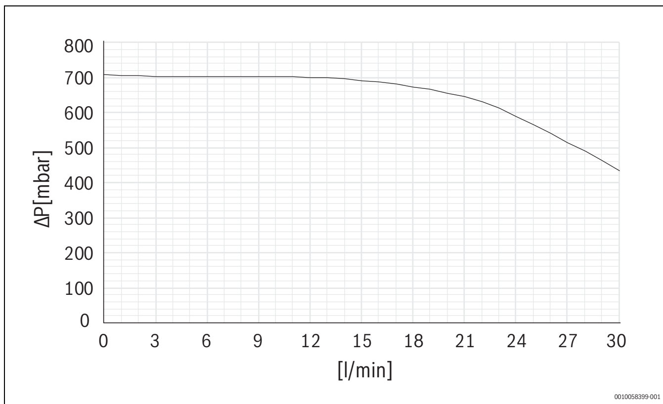
Rys. 40 Wykres wydajności PC0
