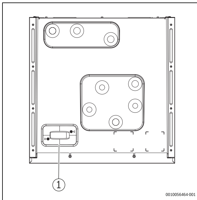
Rys. 13 Montaż Connect-Key
