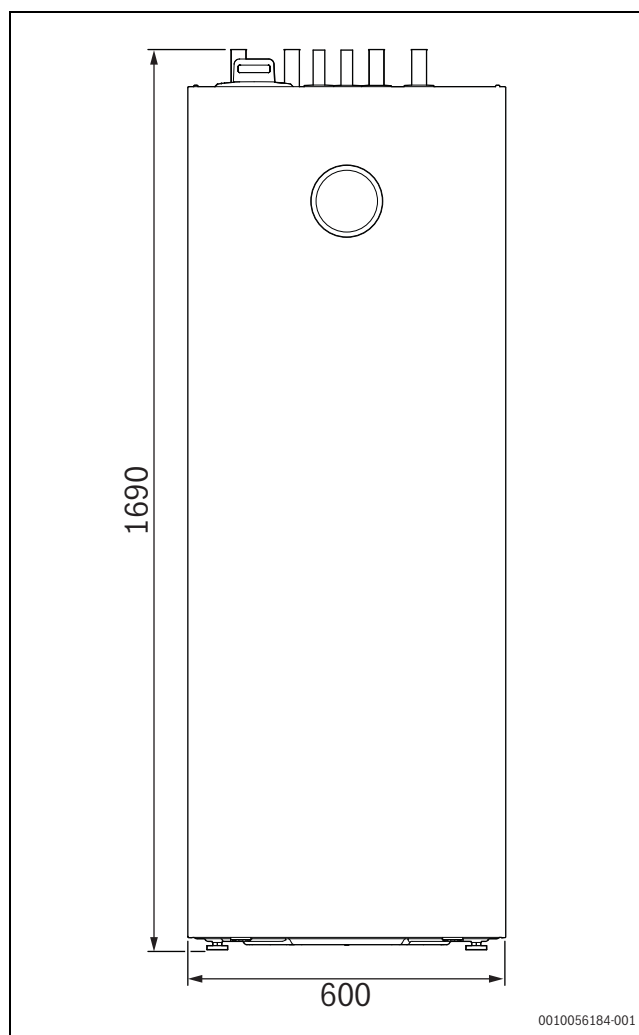
Rys. 3 Wymiary (mm)
