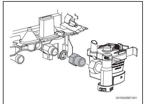
Bild 19 Zusätzliche Buchse
