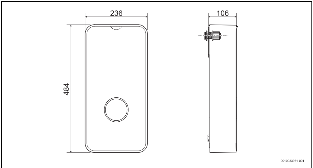
Fig. 29 Dimensions en mm
