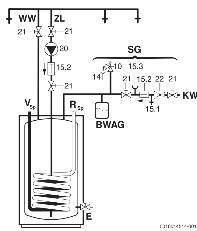
Obr. 8 Schéma pripojenia na strane pitnej vody
