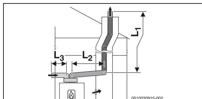
Rys. 16 Elastyczne odprowadzenie spalin wg C 53 w szachcie i instalacja powietrzno-spalinowa z odseparowanymi rurami dla dopływu powietrza i odprowadzenia spalin w pomieszczeniu zainstalowania
