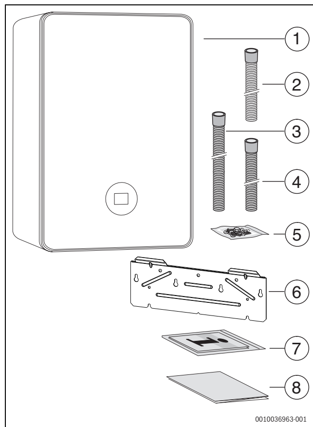
Rys. 1 Zakres dostawy
