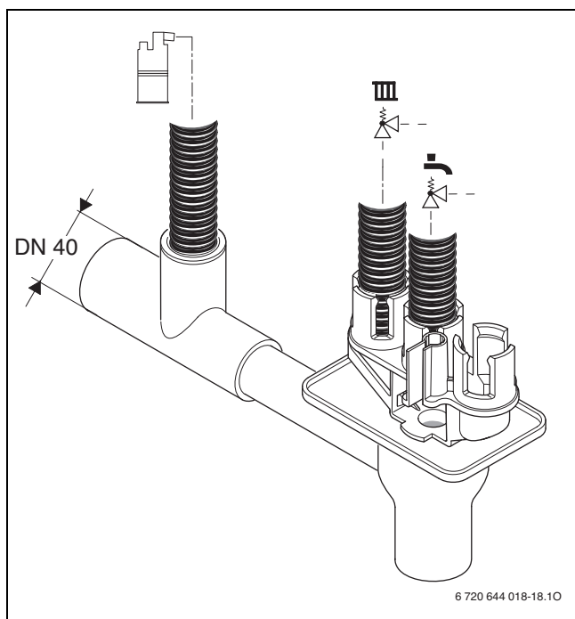
Rys. 39 Montaż węży kondensatu i węży zaworów bezpieczeństwa na syfonie
