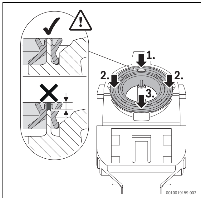
Rys. 74 Docisnięcie uszczelki
