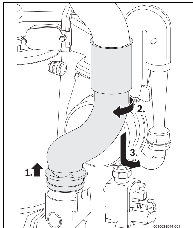
Rys. 58 Demontaż rury spalinowej
