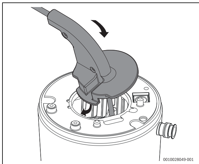
Rys. 65 Umieszczanie szczotki w bloku ciepłym
