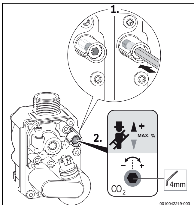
Rys. 53 Ustawianie stężenia \text{CO}_2/\text{O}_2 dla maksymalnej znamionowej mocy cieplnej, armatura gazowa z możliwością ustawienia
