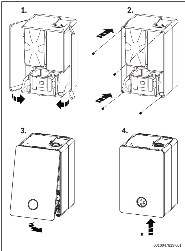
Rys. 47 Montaż obudowy
