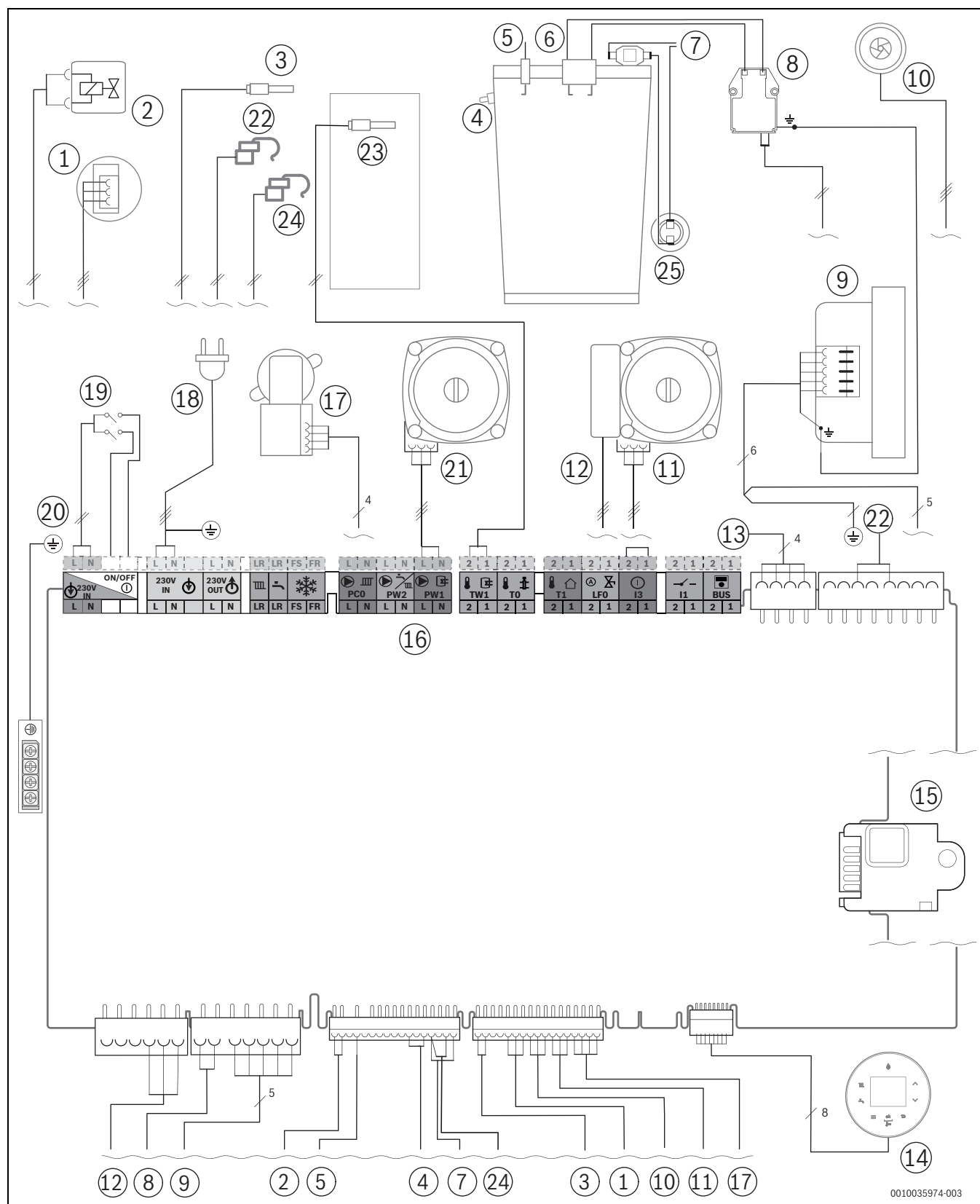
Rys. 91 Okablowanie elektryczne
