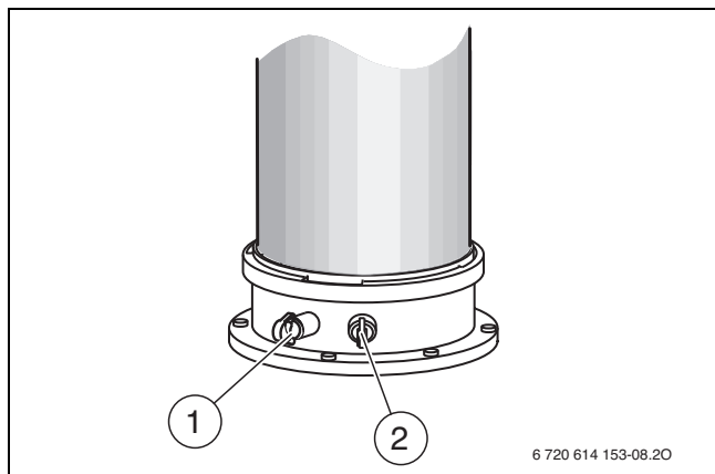
Rys. 55 Króćce pomiarowe spalin oraz powietrza do spalania
