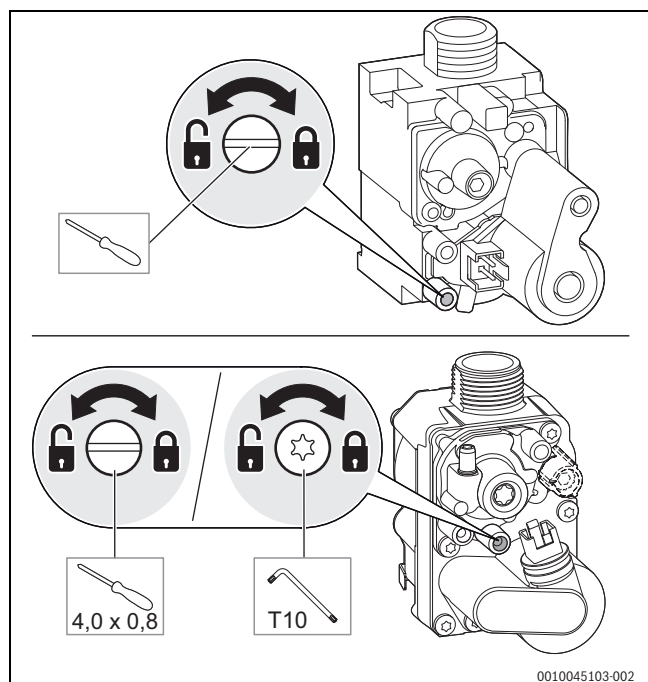
Rys. 51 Pomiar ciśnienia gazu na przyłączy
