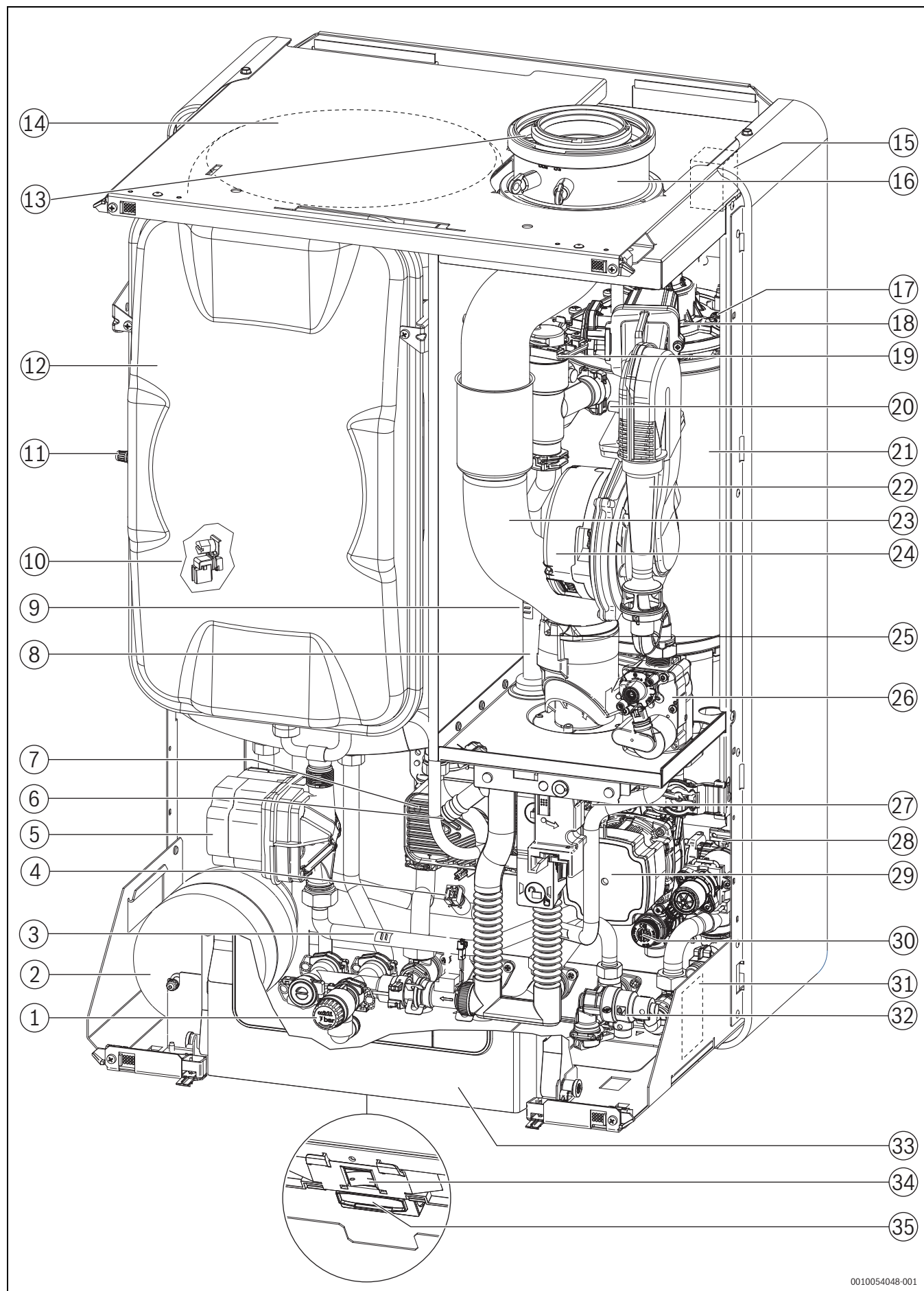
Rys. 5 Przegląd produktu
