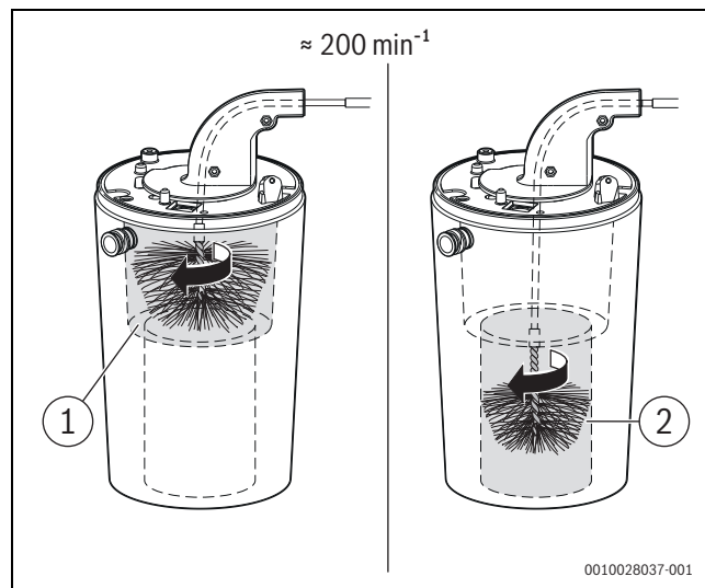
Rys. 67 Czyszczenie bloku ciepłego (ok. 200 min -1 , tylko ruch w prawo)
