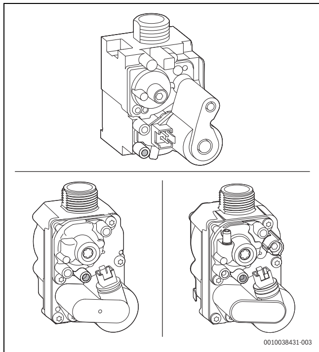
Rys. 49 U góry i na dole po lewej stronie: armatura gazowa bez możliwości ustawienia, na dole po prawej stronie: armatura gazowa z możliwością ustawienia
