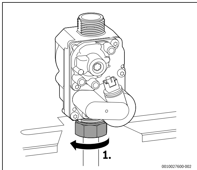
Rys. 80 Luzowanie nakrętki
