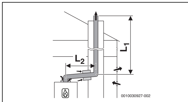
Rys. 20 Sztywne odprowadzenie spalin w szachcie wg B 23p /B 53p z zależnym od powietrza w pomieszczeniu doprowadzeniem powietrza do urządzenia i koncentryczną złączką między pomieszczeniem zainstalowania a szachtem
