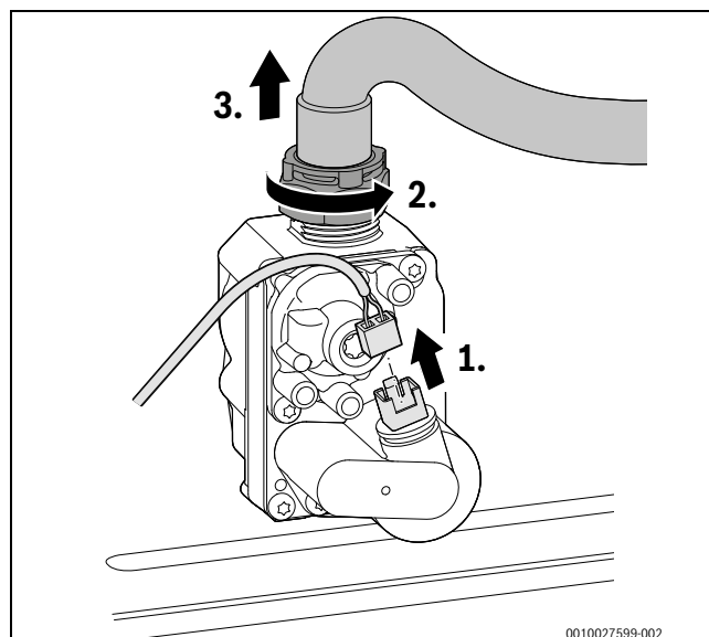
Rys. 78 Odłączanie wtyczki od armatury gazowej i usuwanie nakrętki z węzem gazowym
