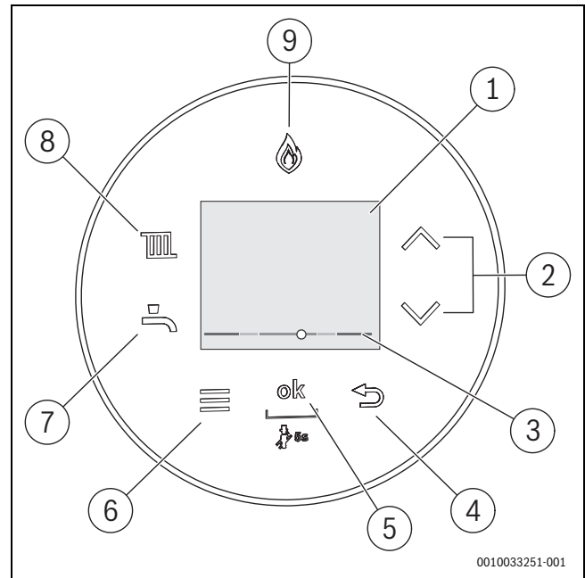
Rys. 48 Panel obsługi
