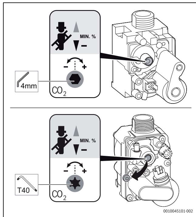
Rys. 54 Ustawianie stężenia \text{CO}_2/\text{O}_2 dla minimalnej znamionowej mocy cieplnej
