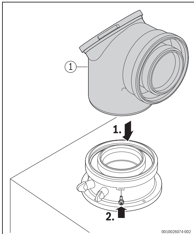
Rys. 41 Wkładanie osprzętu spalinowego i zabezpieczenie go śrubą
