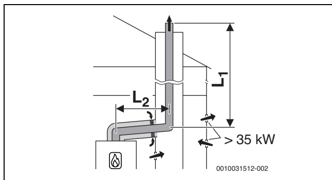
Rys. 22 Sztywne odprowadzenie spalin w szachcie wg B 33 z zależnym od powietrza w pomieszczeniu doprowadzeniem powietrza przez koncentryczną instalację powietrzno-spalinową w pomieszczeniu zainstalowania
