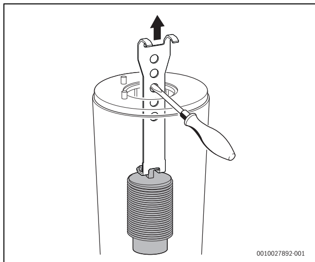
Rys. 64 Wyjmowanie dolnego elementu wyporowego
