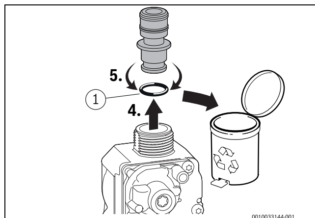
Rys. 79 Usuwanie dławika gazowego
