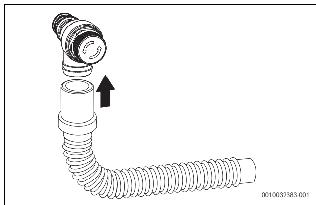
Rys. 36 Montaż węży na zaworze bezpieczeństwa (instalacji grzewczej)
