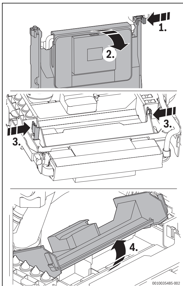
Rys. 44 Otwieranie sterownika
