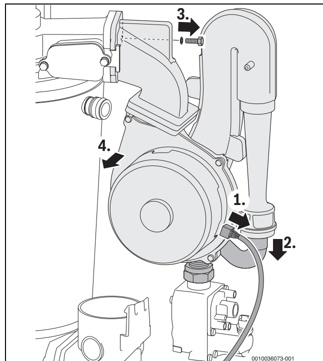
Rys. 59 Demontaż wentylatora z zespołem mieszającym
