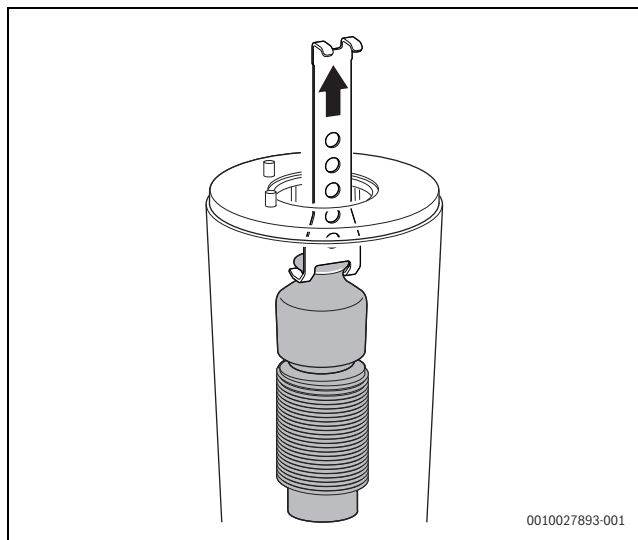
Rys. 63 Wyjmowanie górnego elementu waporowego
