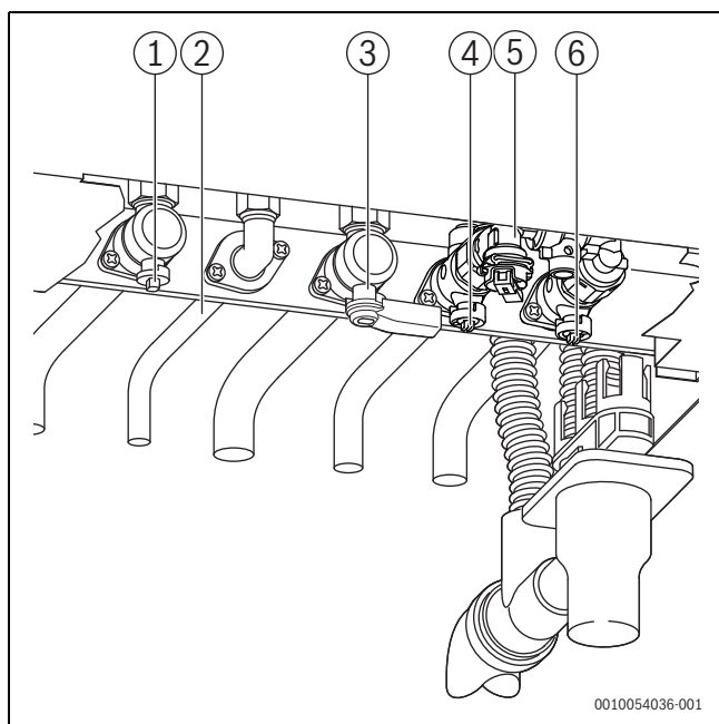
Rys. 42 Przyłącza po stronie gazowej oraz wodnej
