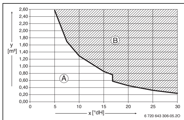
Rys. 29 Wymagania dotyczące wody do napełniania i uzupełniania w °dH do urządzeń o mocy < 50 kW
