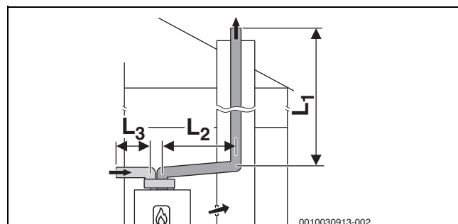
Rys. 15 Sztywne odprowadzenie spalin wg C 53 w szachcie i instalacja powietrzno-spalinowa z odseparowanymi rurami dla dopływu powietrza i odprowadzenia spalin w pomieszczeniu zainstalowania.
