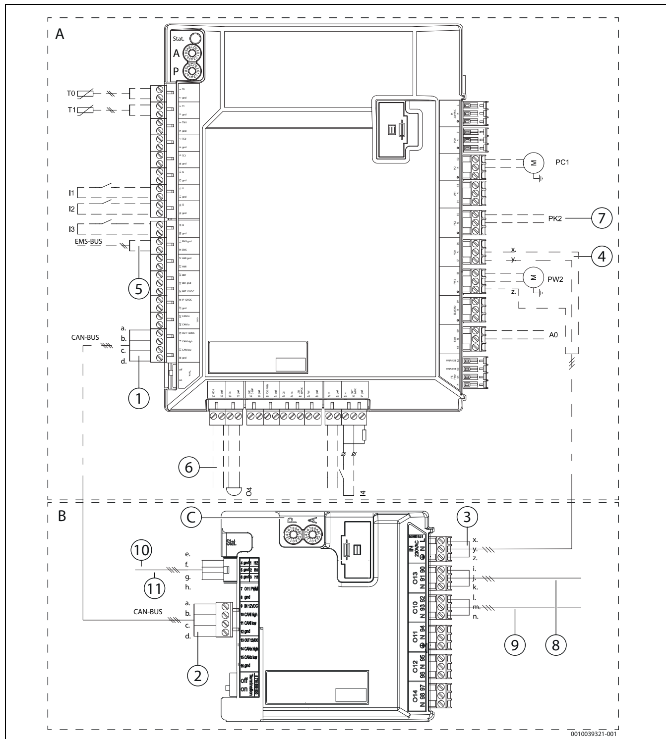
Rys. 9 Schemat połączeń płyty rozszerzającej (stacja chłodzenia) i płyty głównej montażowej (pomp ciepła)
