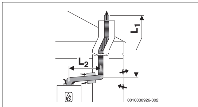
Rys. 22 Elastyczne prowadzenie spalin w szachcie zgodnie z B 53p z dopływem powietrza zależnym od powietrza w pomieszczeniu przy urządzeniu i koncentrycznej złączce między pomieszczeniem instalacyjnym a szachtem
