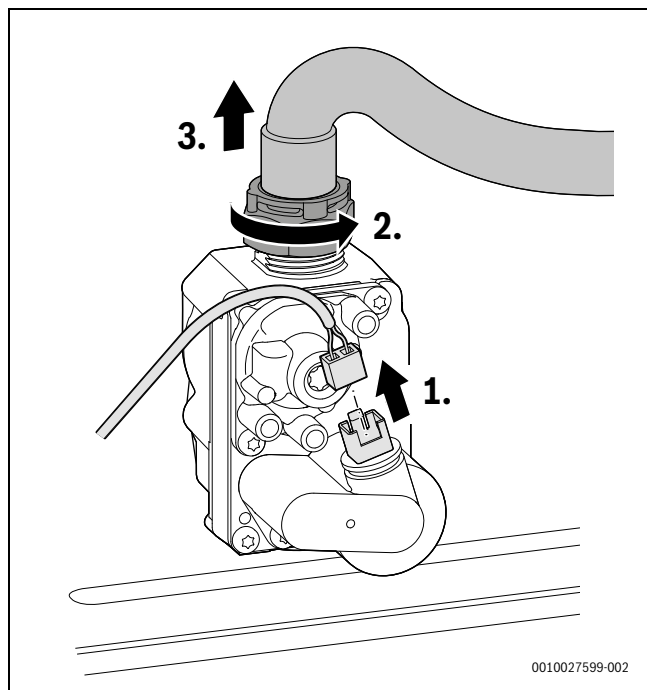
Rys. 73 Odłączanie wtyczki od armatury gazowej i usuwanie nakrętki z węzłem gazowym
