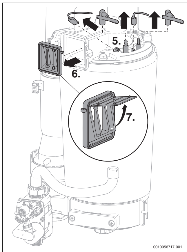
Rys. 56 Odłączanie kabli
