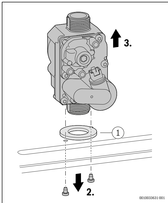
Rys. 76 Demontaż armatury gazowej
