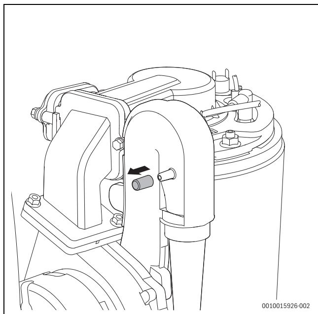
Rys. 52 Króciec pomiarowy na zespole mieszającym
