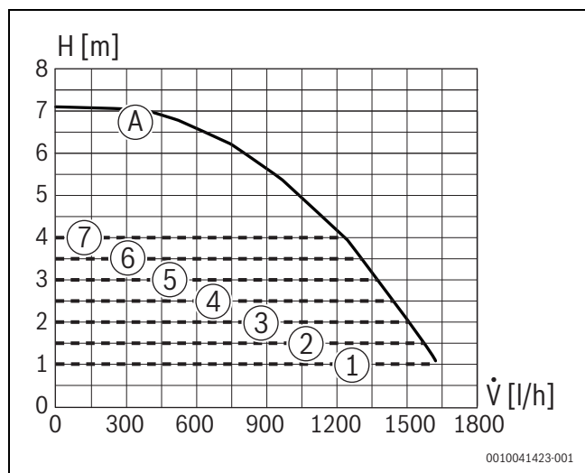
Rys. 91 Charakterystyki wykreslna pompy i charakterystyki pompy
