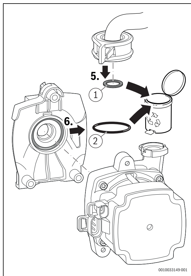
Rys. 72 Utylizacja uszczelki
