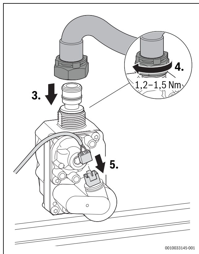
Rys. 80 Podłączanie węża gazowego i wtyczki – Przestrzeganie momentu dokręcenia
