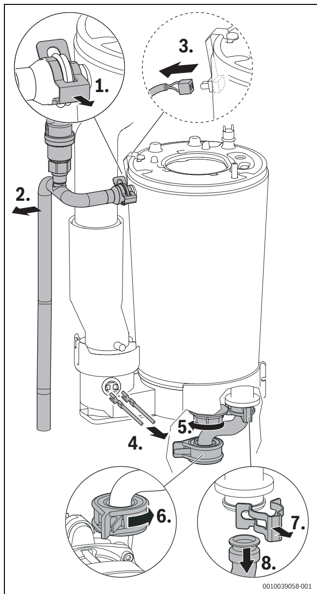
Rys. 67 Odłączanie rury zasilania, kabla i rury powrotu
