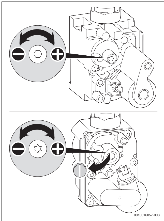
Rys. 49 Regulacja armatury gazowej
