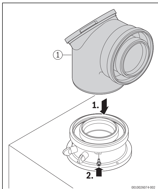
Rys. 39 Wkładanie osprzętu spalinowego i zabezpieczenie go śrubą
