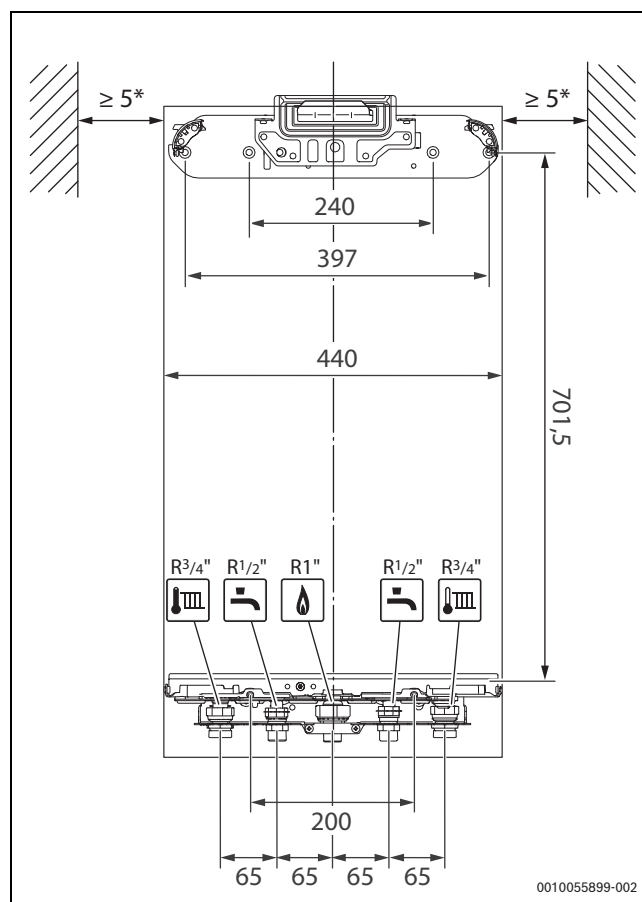
Rys. 3 Widok z przodu (mm)
