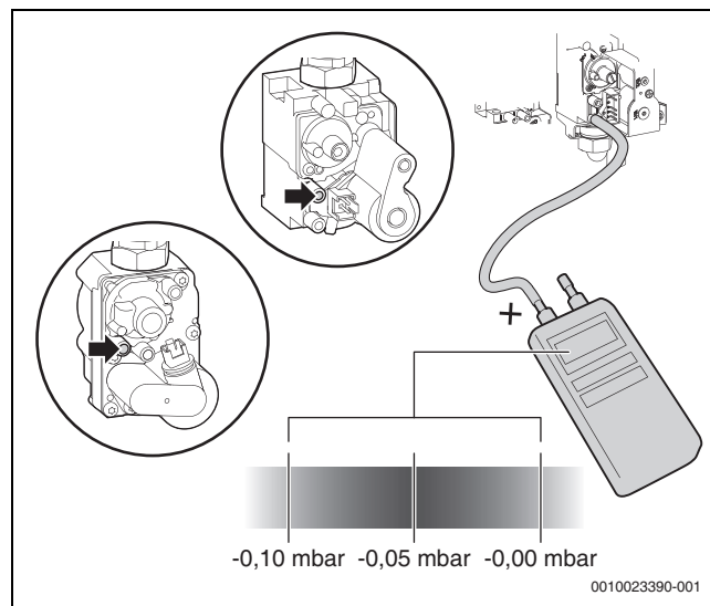
Rys. 48 Pomiar różnicy ciśnień
