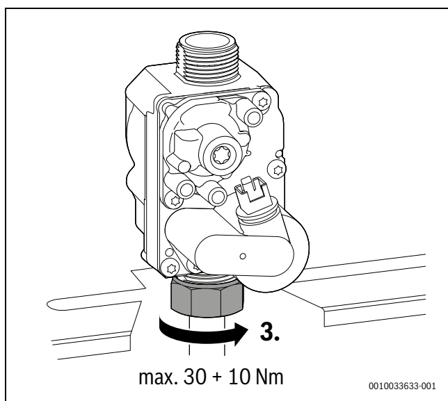
Rys. 78 Przestrzeganie momentu dokręcenia
