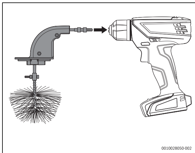
Rys. 62 Łączenie szczotki z wkrętkarką akumulatorową
