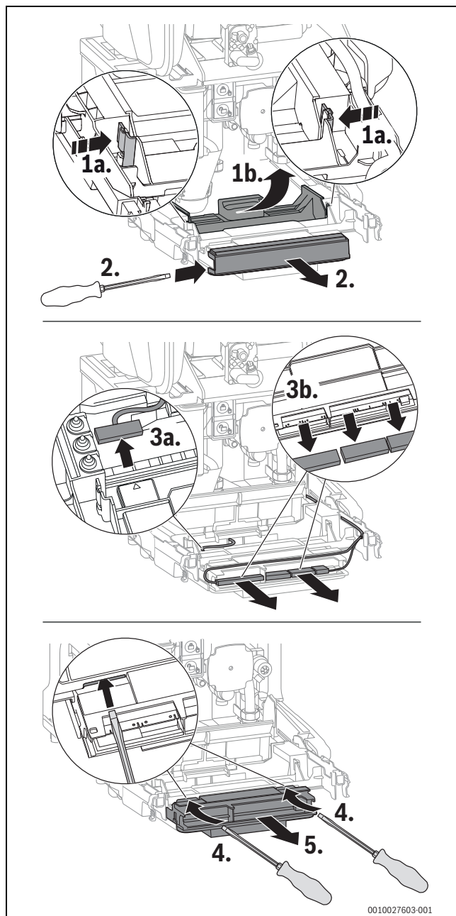
Rys. 81 Wyjmowanie sterownika
