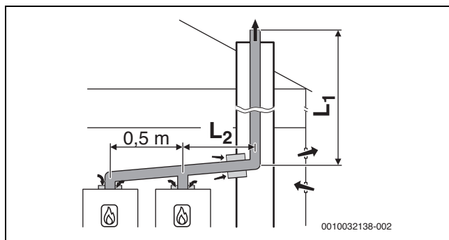
Rys. 29 Kaskada z 2 urządzeniami: Sztywne odprowadzenie spalin w szachcie wg B 53p z zależnym od powietrza w pomieszczeniu doprowadzeniem powietrza do urządzenia
