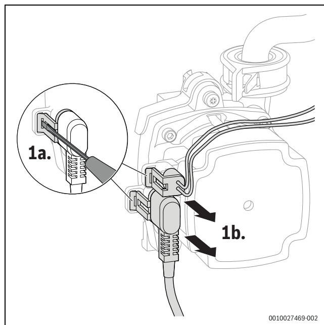
Rys. 69 Odłączanie wtyczki od pompy c.o.
