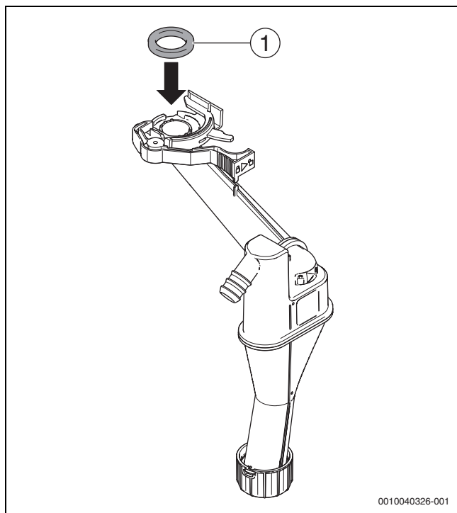
Rys. 84 Ułożenie nowej uszczelki na syfonie kondensatu
