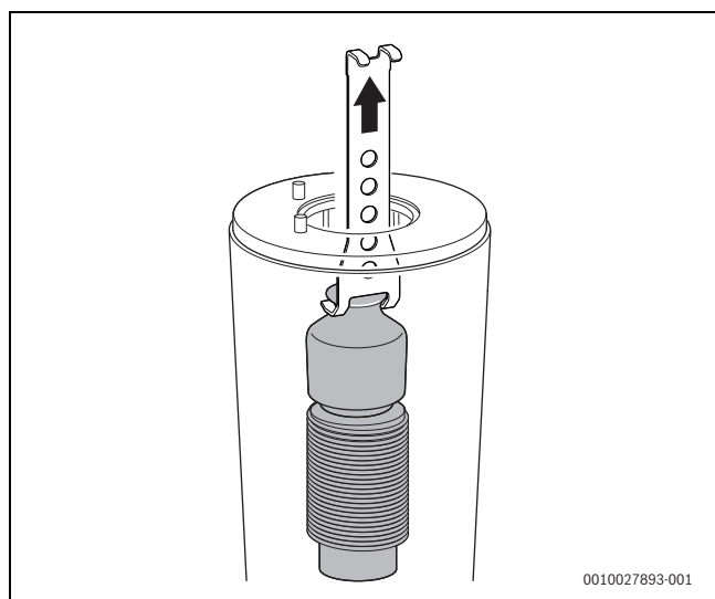
Rys. 59 Wyjmowanie górnego elementu wyporowego
