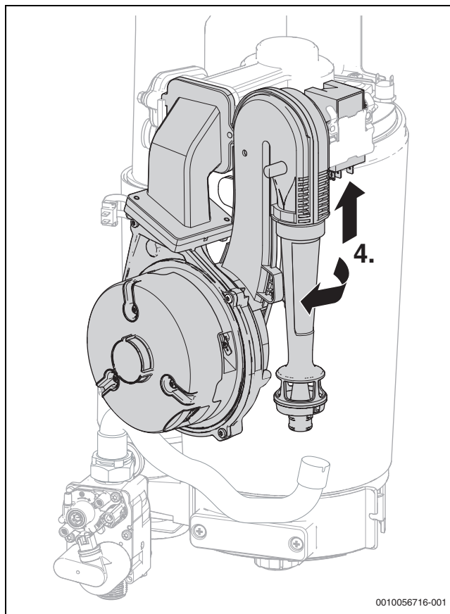
Rys. 55 Wyjąć rurkę Venturiego z zespołem mieszającym i wentylator
