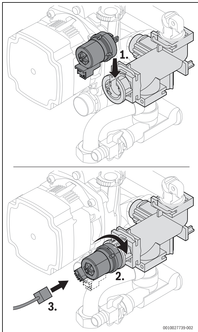
Rys. 88 Montaż napędu zaworu 3-drogowego (wariant bez śrub)
