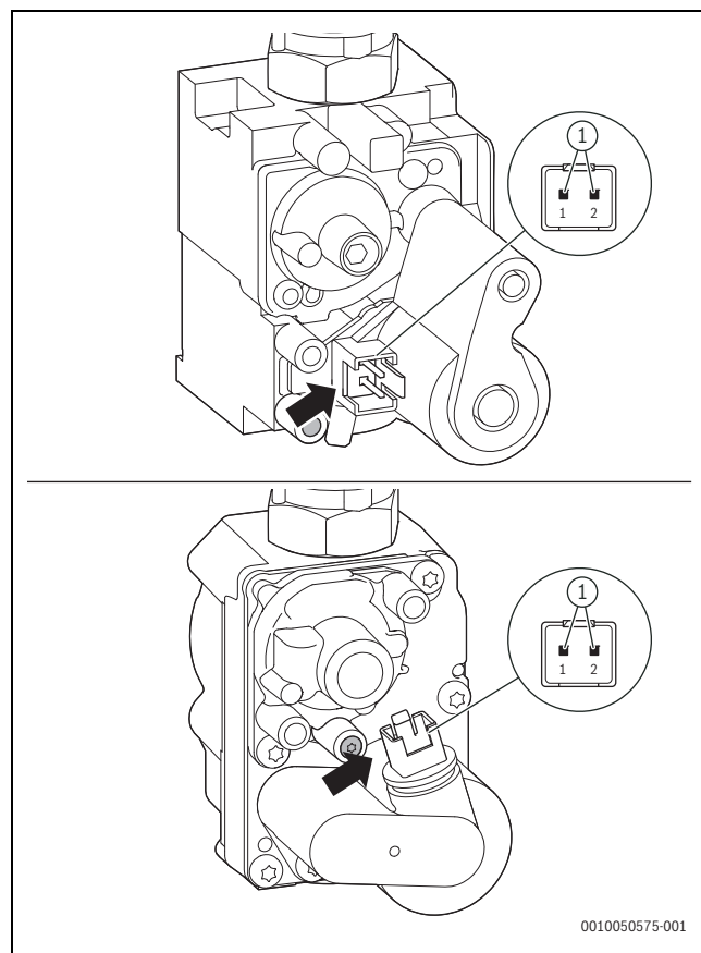
Rys. 53 Punkty pomiarowe na armaturze gazowej
