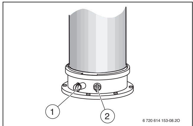
Rys. 51 Króćce pomiarowe spalin oraz powietrza do spalania
