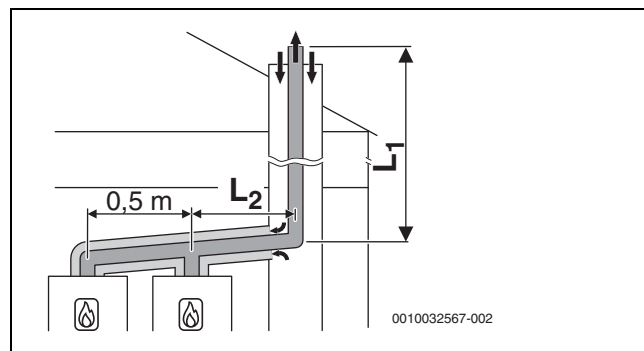
Rys. 30 Kaskada z 2 urządzeniami: Sztywne odprowadzenie spalin wg C 93x w szachcie i koncentryczna instalacja powietrzno-spalinowa w pomieszczeniu zainstalowania
