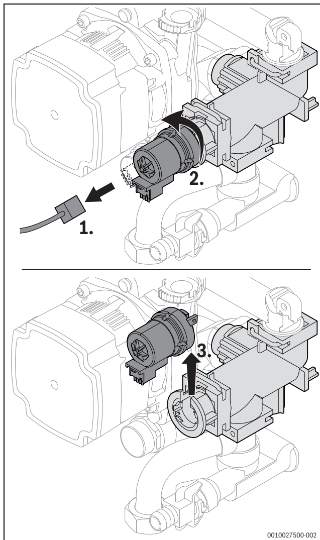
Rys. 87 Demontaż napędu zaworu 3-drogowego (wariant bez śrub)
