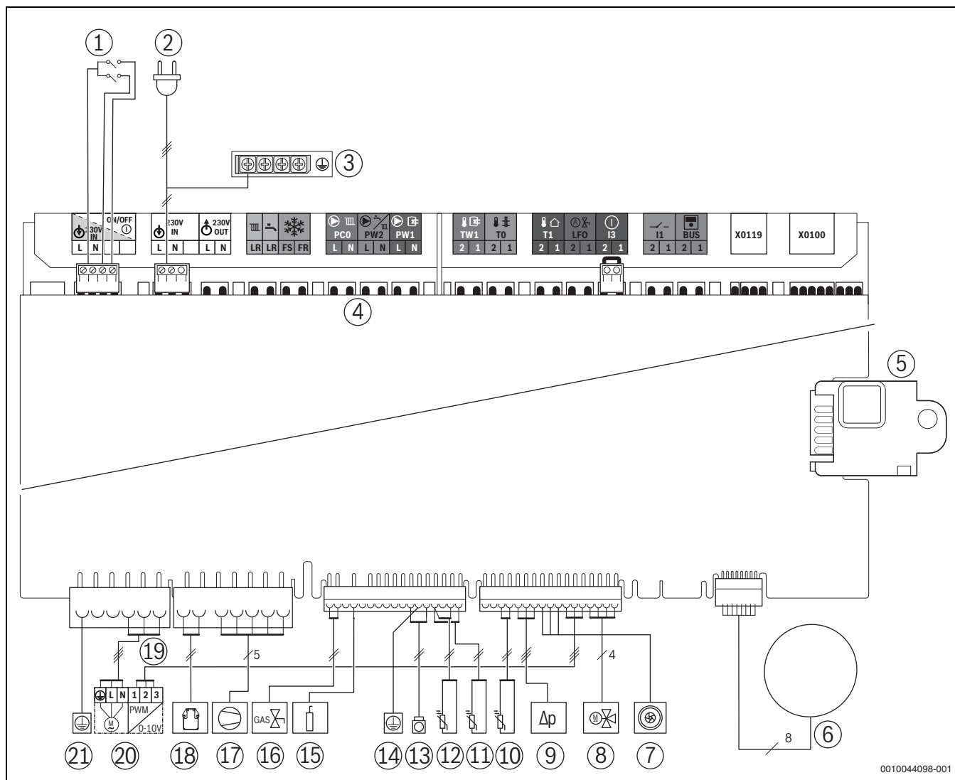
Rys. 92 Okablowanie elektryczne
