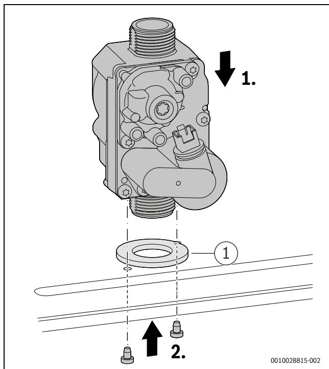
Rys. 77 Montaż armatury gazowej
