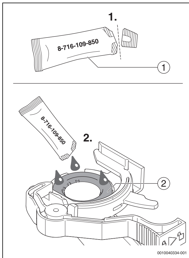
Rys. 85 Smarowanie uszczelki
