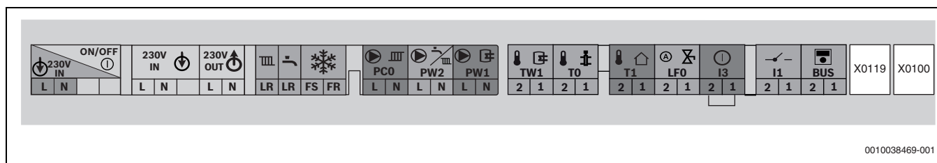
Rys. 43 Listwa zaciskowa dla zewnętrznego osprzętu dodatkowego
