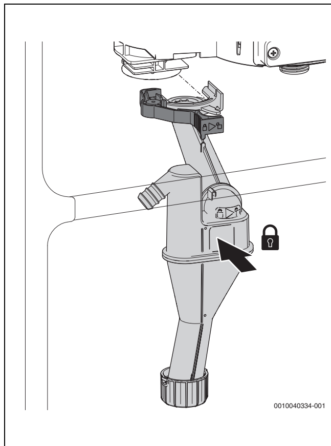
Rys. 86 Zakładanie syfonu kondensatu
