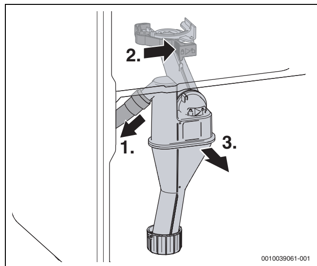
Rys. 82 Demontaż syfonu kondensatu
