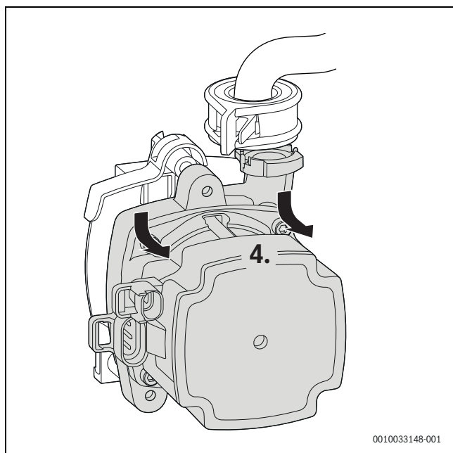
Rys. 71 Wyjmowanie pompy c.o.
