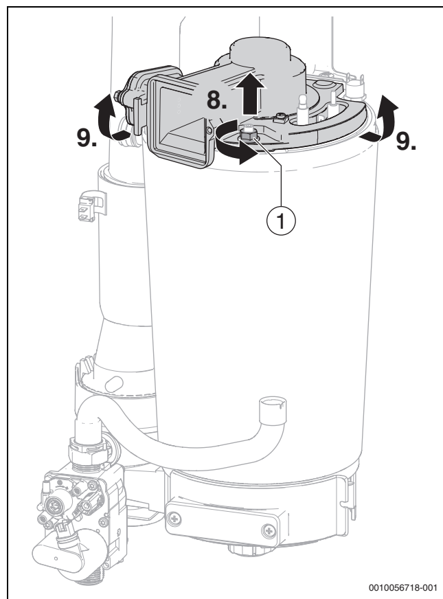
Rys. 57 Zdejmowanie pokrywy palnika z wentylatorem i z zespołem mieszającym
