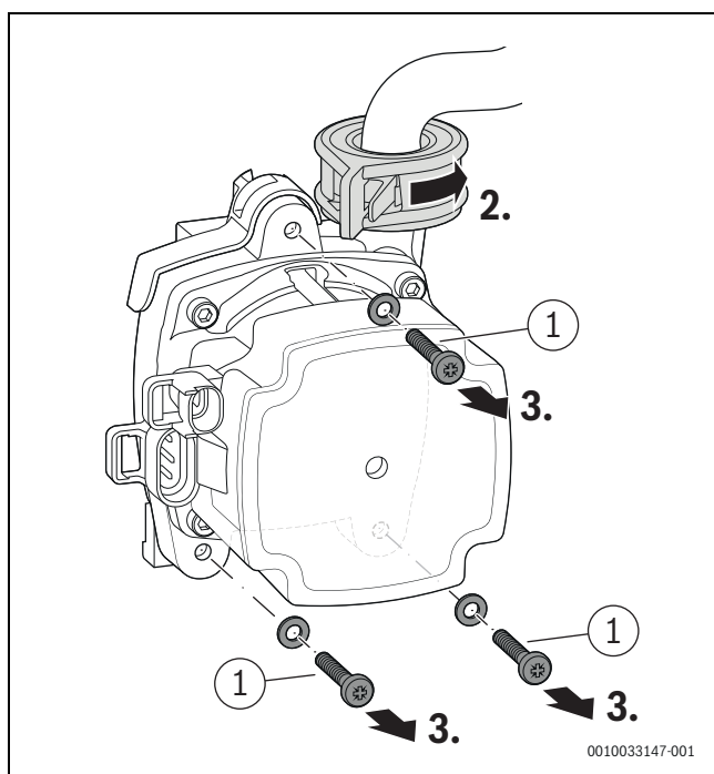
Rys. 70 Odblokowanie pompy c.o. i usuwanie śrub
