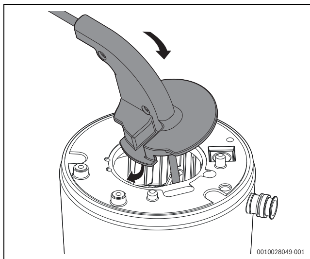
Rys. 61 Umieszczanie szczotki w bloku cieplnym
