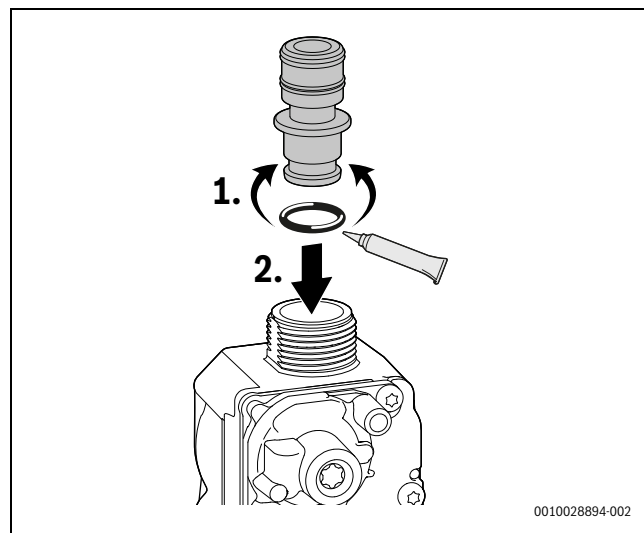
Rys. 79 Wkładanie dławika gazowego
