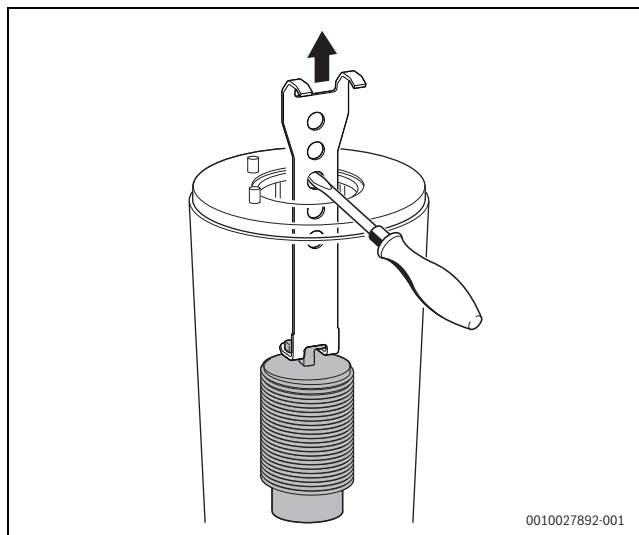
Rys. 60 Wyjmowanie dolnego elementu wyporowego
