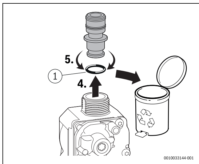
Rys. 74 Usuwanie dławika gazowego
