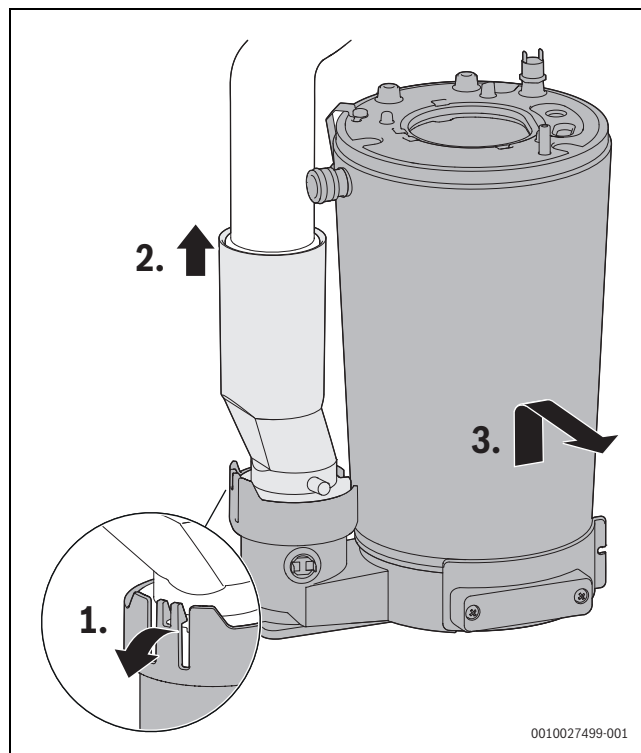
Rys. 68 Demontaż bloku cieplnego
