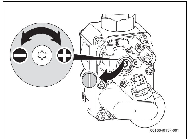
Rys. 50 Zdejmowanie plomby ze śruby nastawczej
