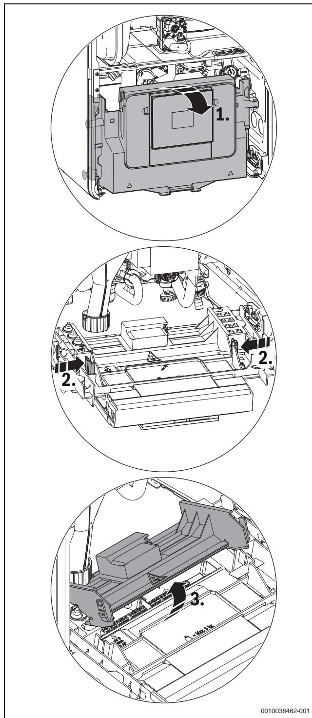
Rys. 41 Otwieranie pokrywy
