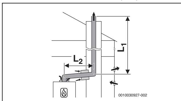
Rys. 21 Sztywne prowadzenie spalin w szachcie zgodnie z B 53p z dopływem powietrza zależnym od powietrza w pomieszczeniu przy urządzeniu i koncentrycznej łączce między pomieszczeniem instalacyjnym a szachtem
