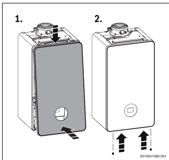
Rys. 44 Montaż obudowy
