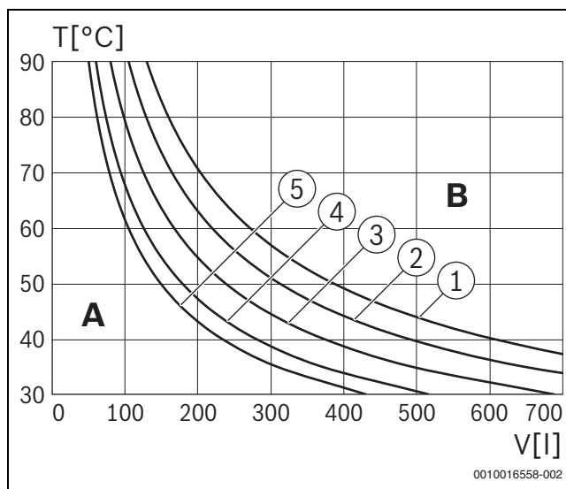
Rys. 32 Charakterystyki naczynia wzbiórczego
