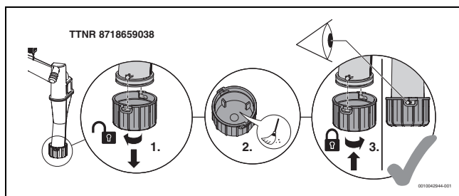
Rys. 83 Czyszczenie osadnika zanieczyszczeń
