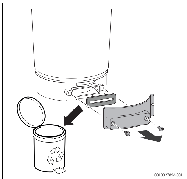
Rys. 64 Otwieranie otworu kontrolnego
