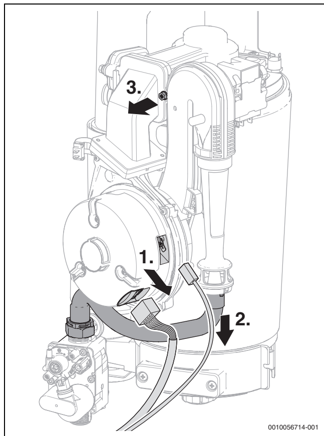
Rys. 54 Wyciągnąć wtyczkę i odłączyć wąż gazu, odkręcić śrubę
