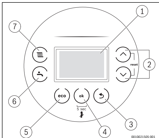
Rys. 2 Panel obsługi
